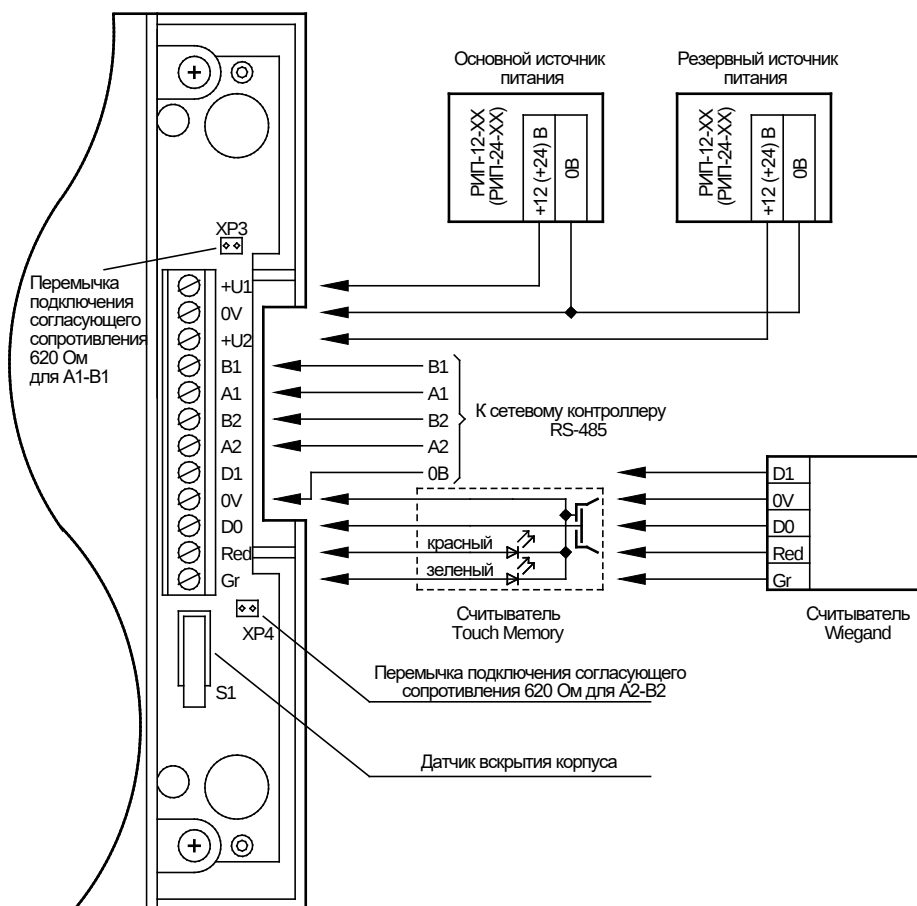
Рисунок 3. Схема внешних соединений блока «C2000-БИ 2RS485», «C2000-БИ исп.02 2RS485»
