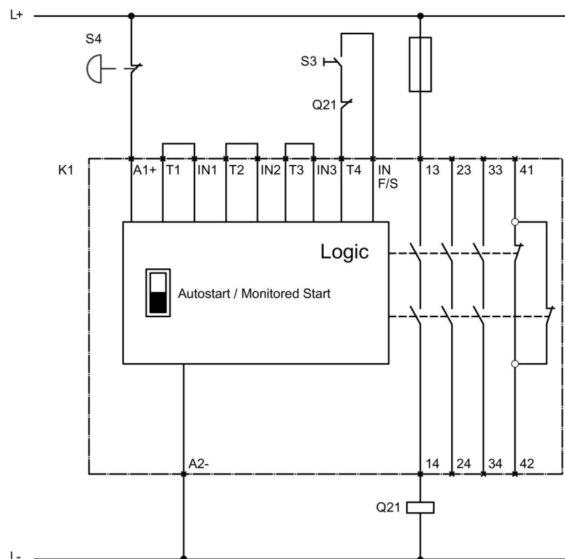
Электрическая схема подключения реле безопасности 3SK1
