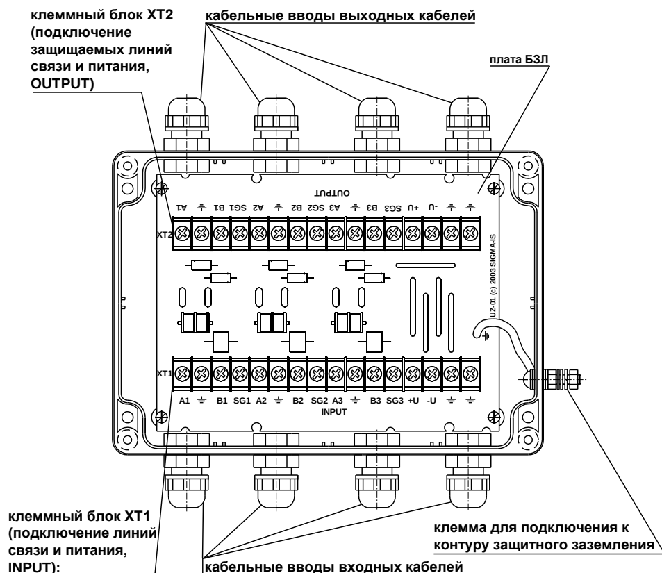
Рис. 9. БЗЛ-01, БЗЛ-04. Кабельные вводы и клеммные блоки
