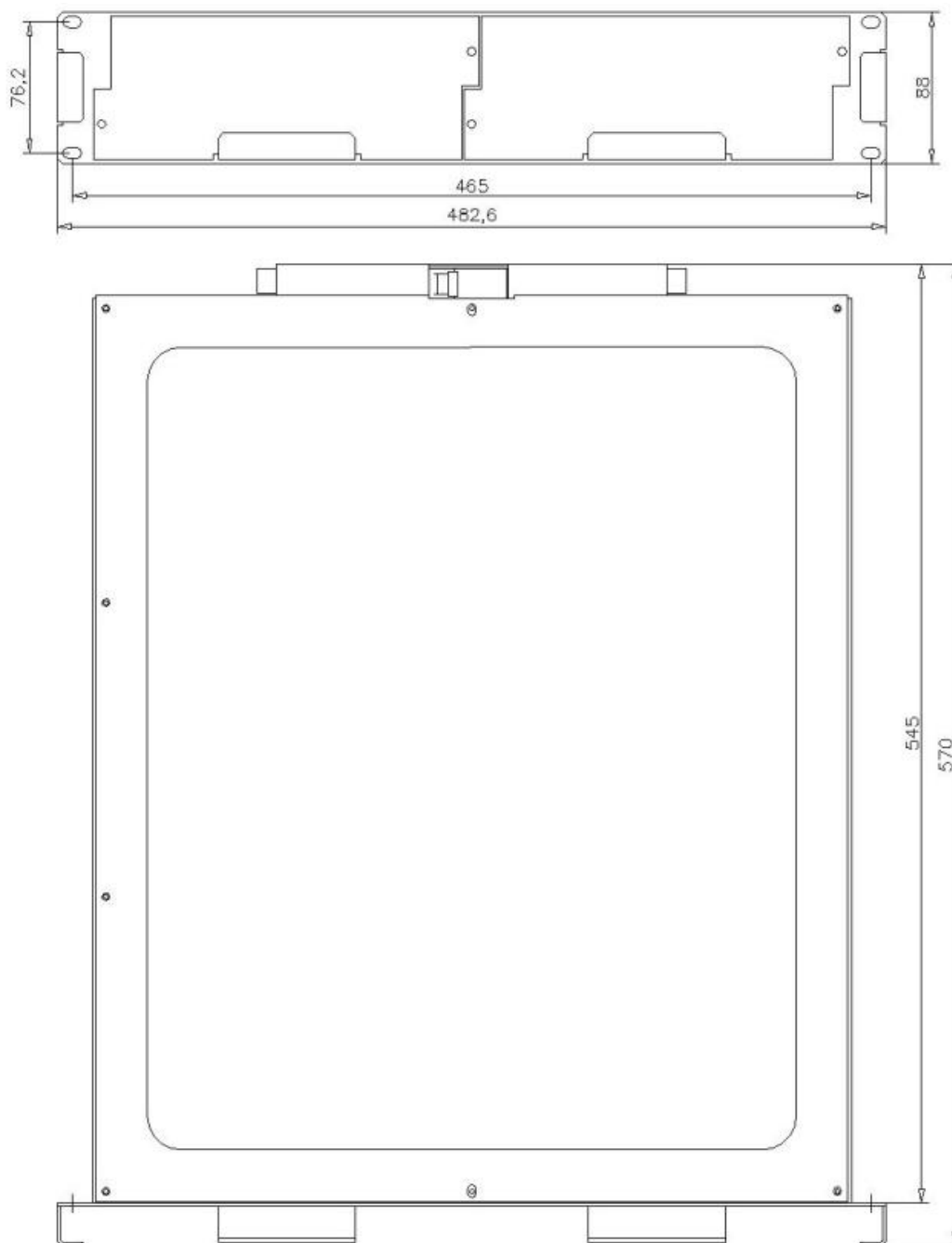
Рисунок 1 – Габаритные размеры и внешний вид изделия
