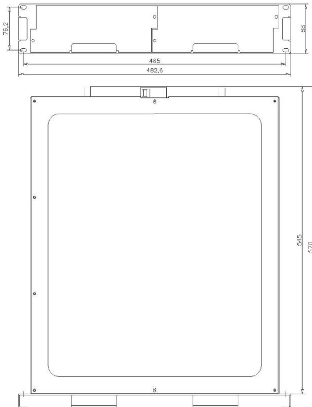
Рисунок 1 – Габаритные размеры и внешний вид изделия
