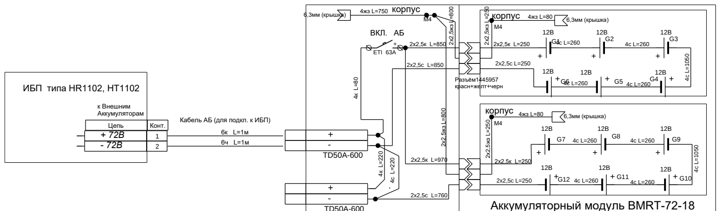
Рисунок 3 - Схема электрическая соединений
