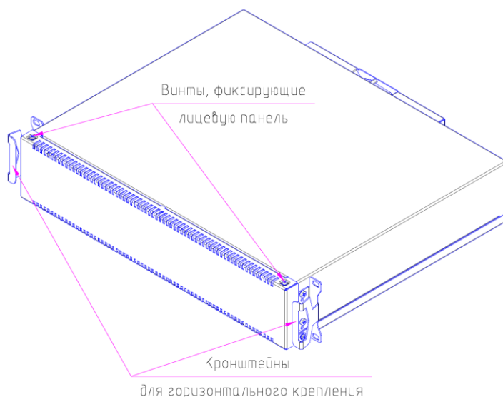
б) горизонтальная установка
