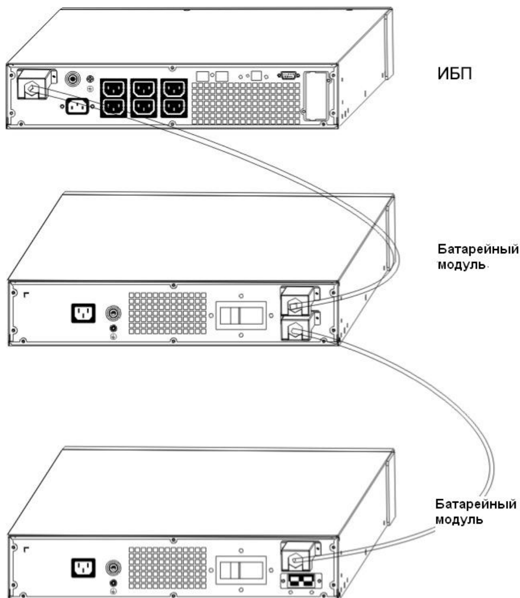
Рисунок 17 Последовательное соединение
