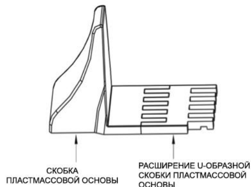
Рисунок 6 Пластмассовая основа 1,5/2/3 кВА (В)
