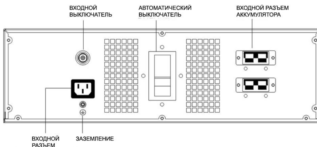
Рисунок 3 Задняя панель аккумуляторного блока 1,5 / 2 / 3 кВА
