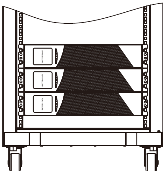
Рисунок 13. Стойка в собранном виде
