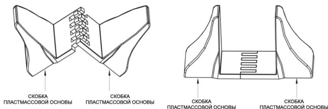
Рисунок 4 Сборка пластмассовой основы аккумуляторного блока 1 кВА
