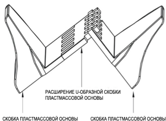
Рисунок 5 Пластмассовая основа 1,5/2/3 кВА (А)
