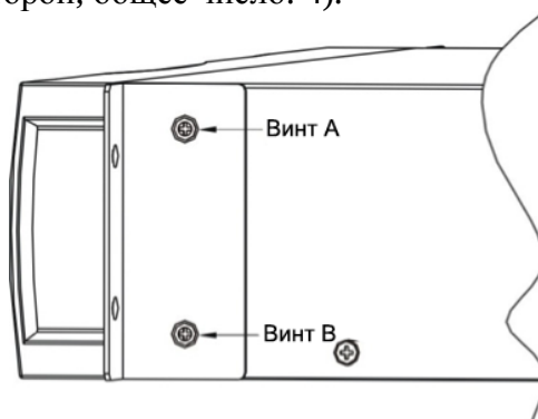
Рисунок 12 Сборка крепления для установки в 19' стойку
