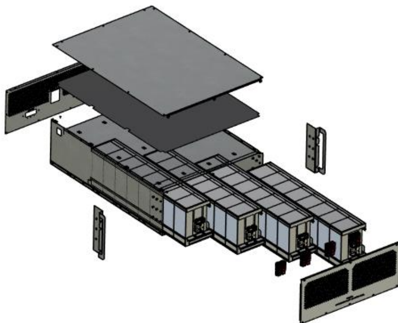
Рис.4. Батарейный модуль в разобранном виде
