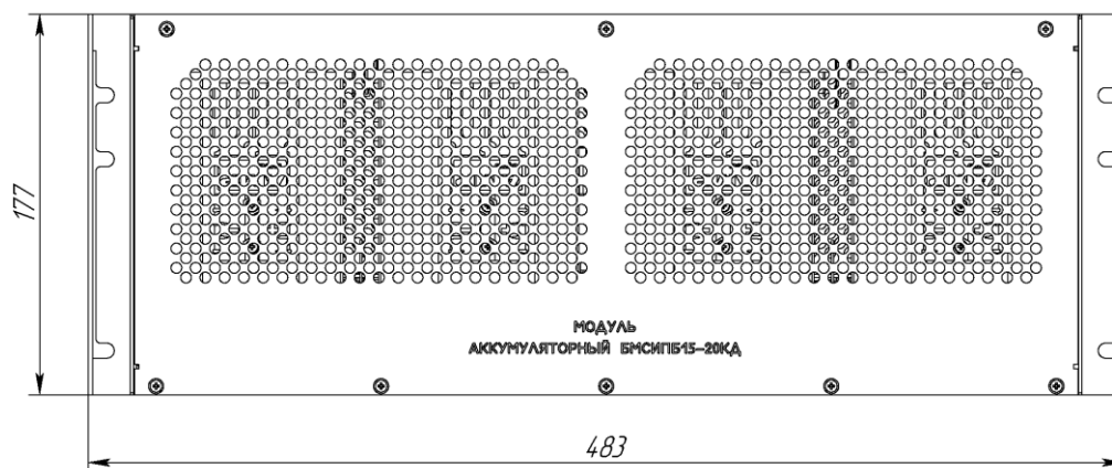
Вид спереди
