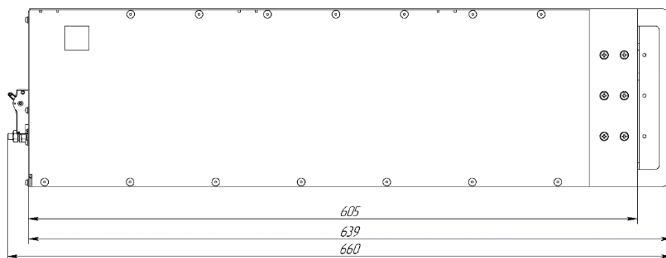
Вид сбоку
