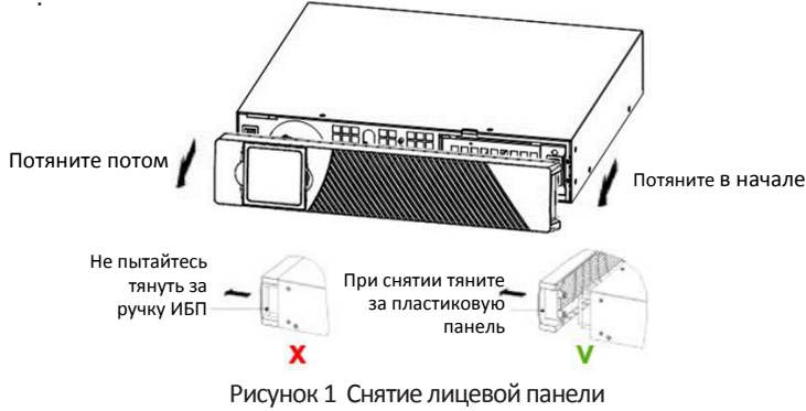
Рисунок 1 Снятие лицевой панели
