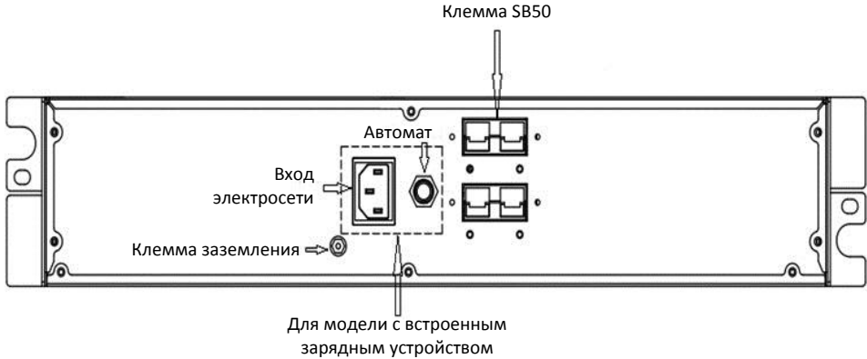
Рис.8 Задняя панель батарейного блока
