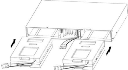
Рис.5 Снятие и установка блоков аккумуляторов
