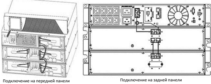
Рисунок 3 Подключение БМ
