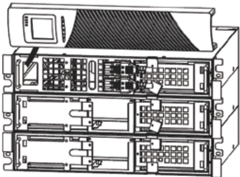
Рисунок 3 Типовая установка дополнительных батарейных блоков
