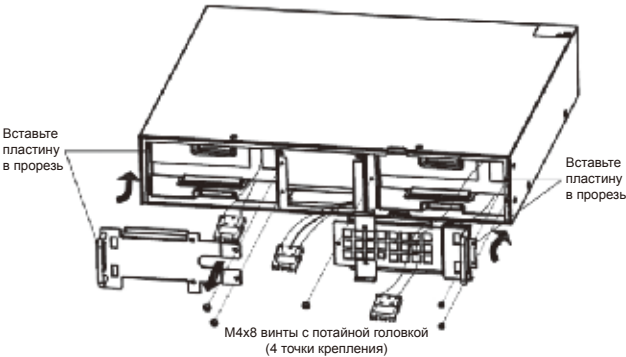
Рисунок 6 Установка перегородок блоков батарей
