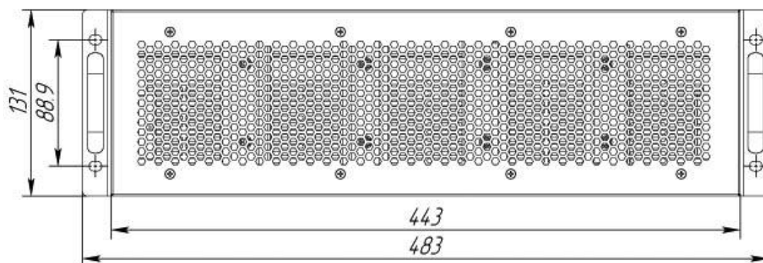
Вид спереди
