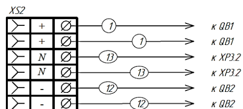
Панель внешних подключений
