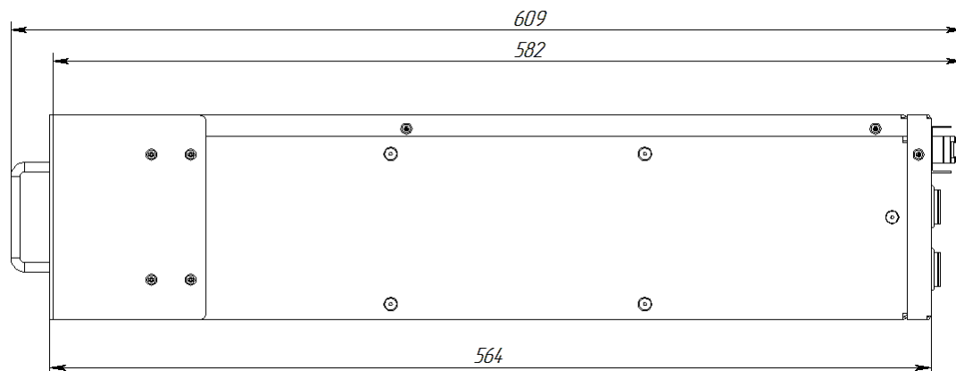
Вид справа
