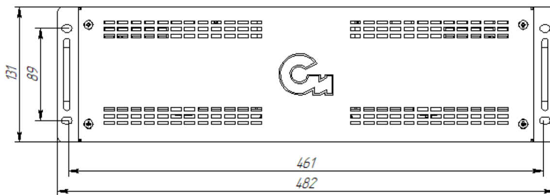
Вид спереди
