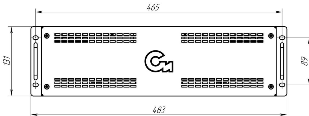
Вид спереди
