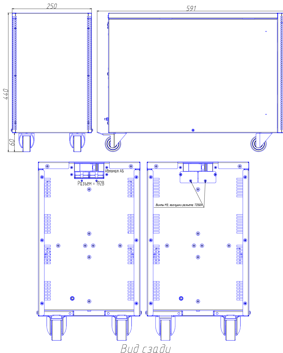
Рисунок 1 – Габаритные размеры и внешний вид изделия
