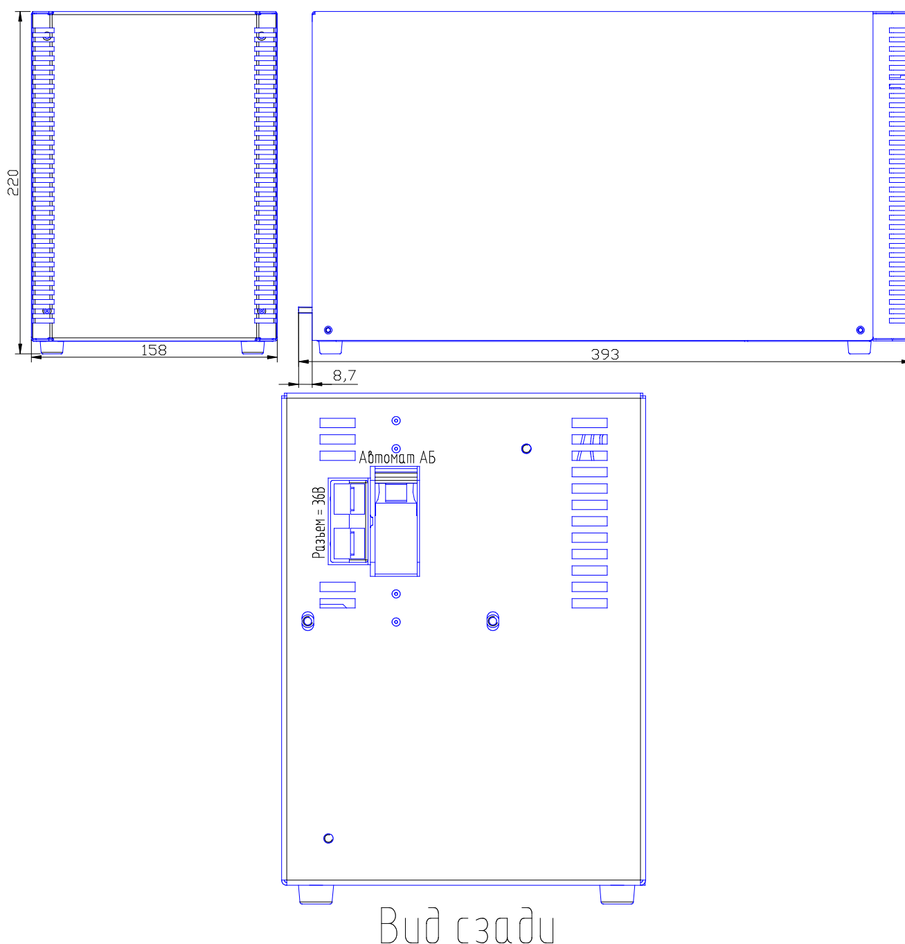
Рисунок 1 – Габаритные размеры и внешний вид изделия
