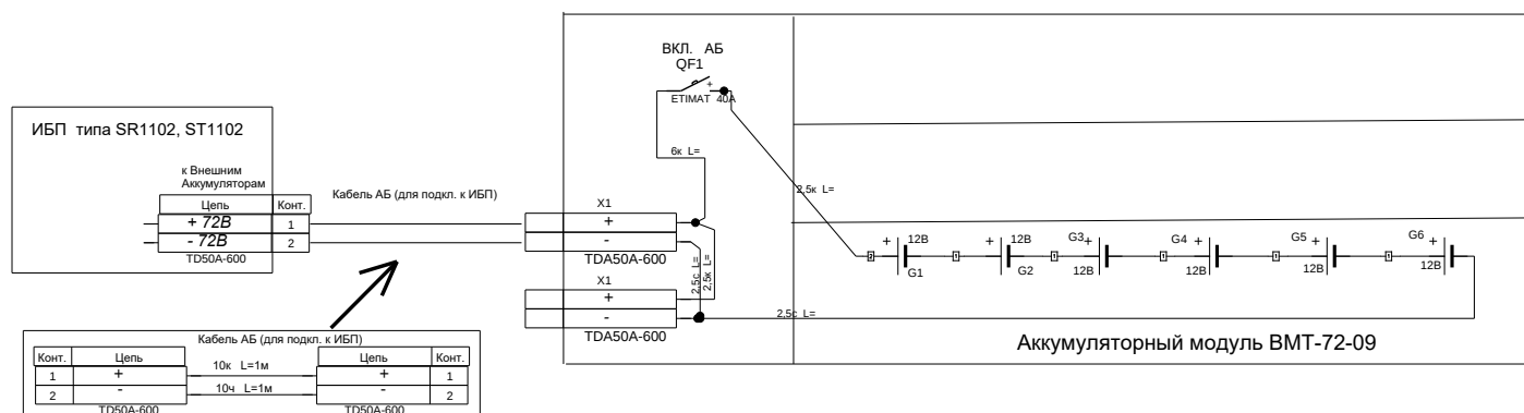
Рисунок 2 – Схема электрическая соединений
