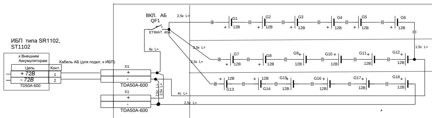
Рисунок 2 – Схема электрическая соединений
