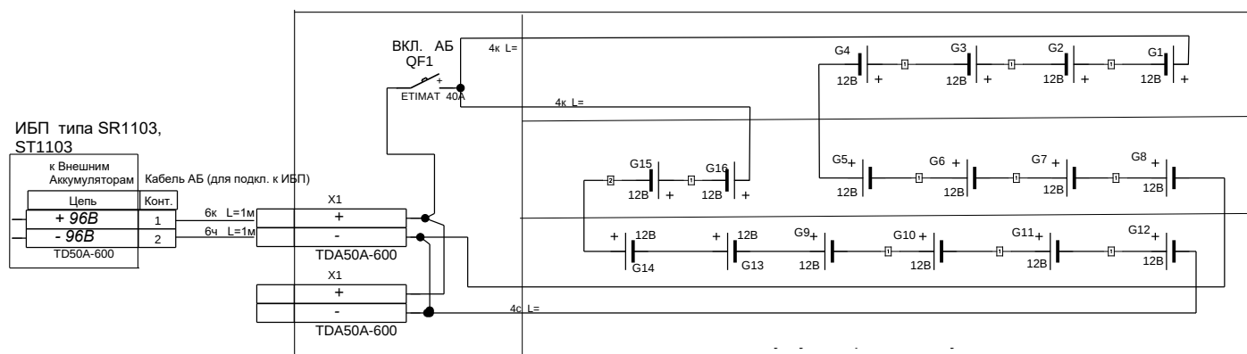
Рисунок 2 – Схема электрическая соединений
