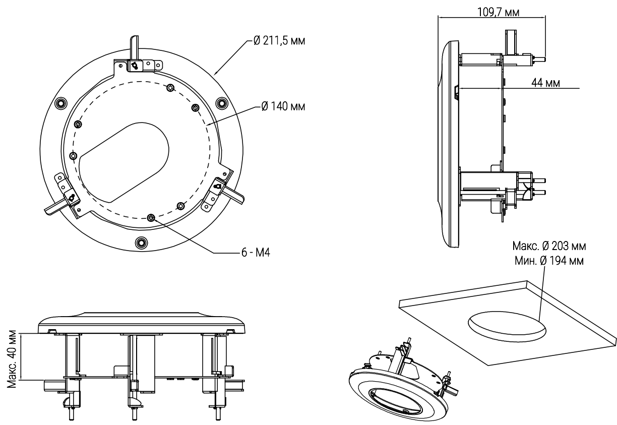
Рисунок 4.1 – Габаритные размеры
