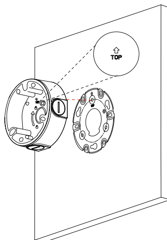
Рисунок 4.5 – Монтаж
