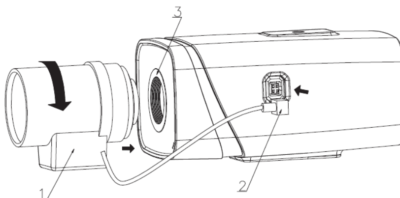
Рисунок 5.2 – Установка объектива на камеру
