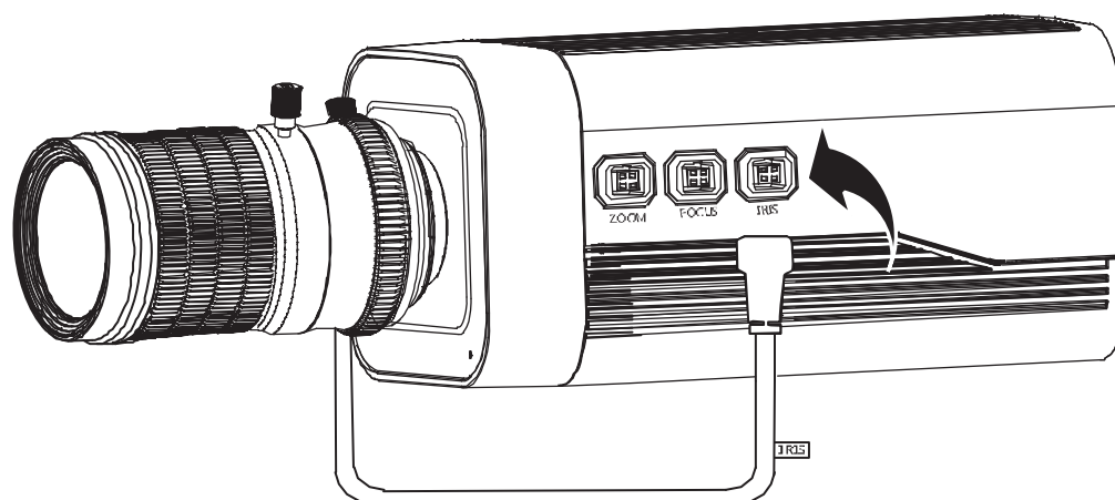
Рисунок 7.3 – Установка объектива
