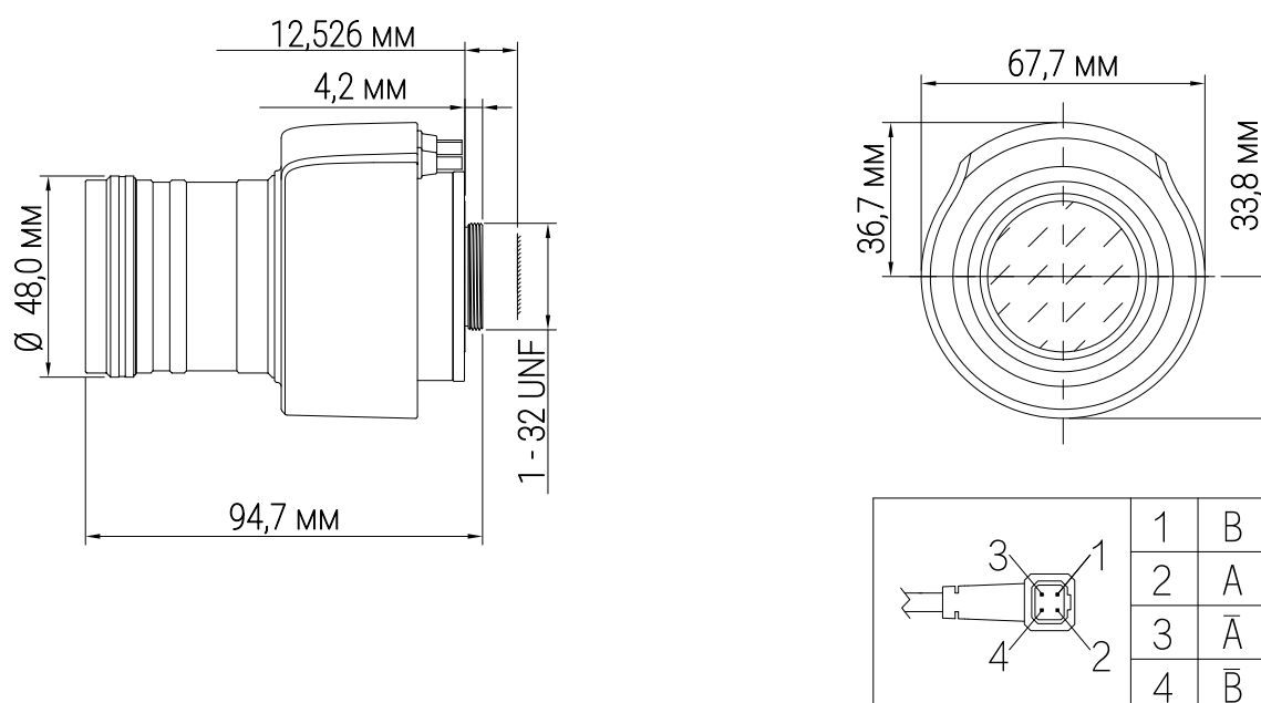
Рисунок 5.1 – Габаритные размеры
