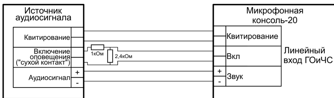
Рисунок 1.4.2. Схема подключения источника сигнала ГОиЧС.
