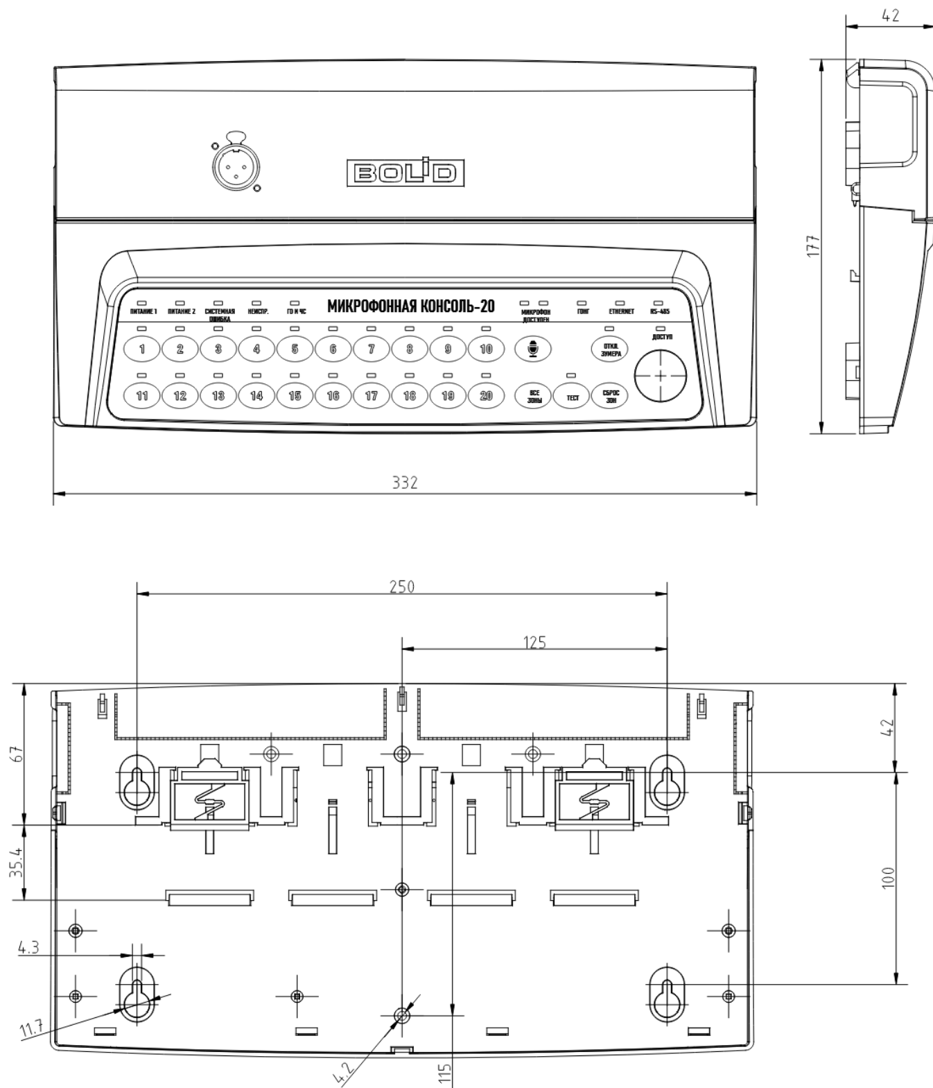
Рисунок 2.2.2. Габаритные и установочные размеры консоли.
