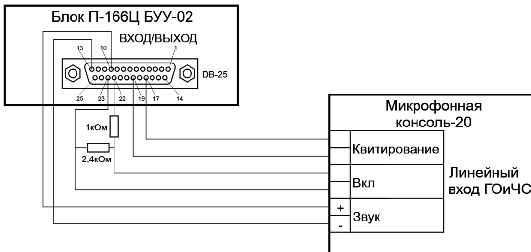
Рисунок 1.4.3. Схема подключения блока управления П-166Ц БУУ-02.
