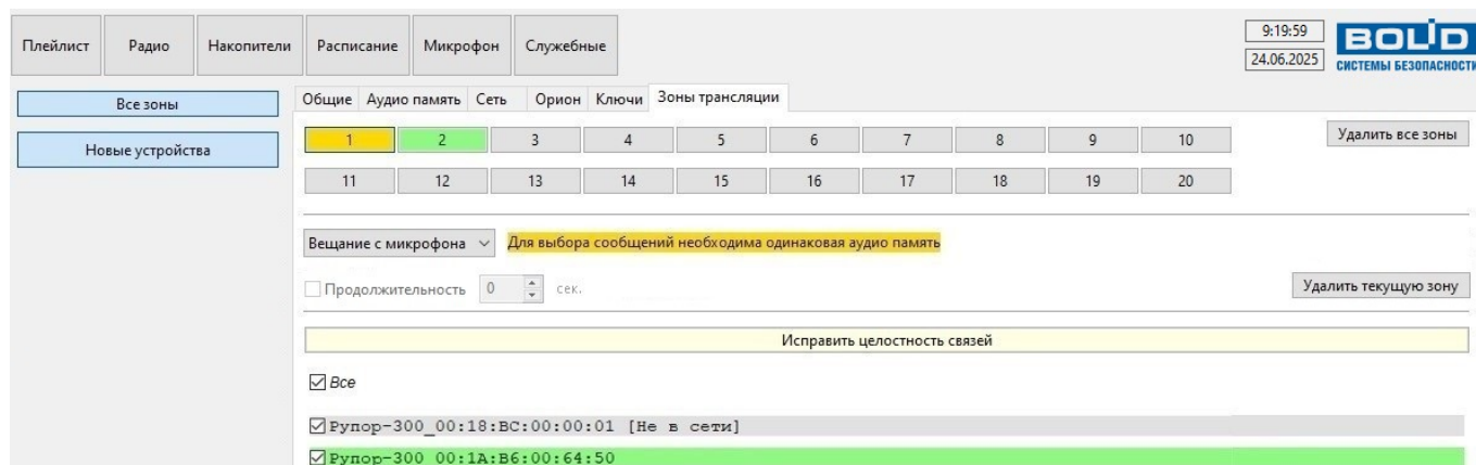
Рисунок 2.2.23. Отображение неисправности зоны.
