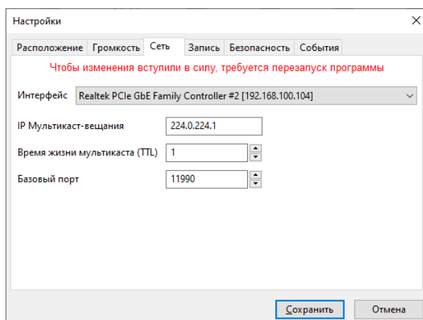
Рисунок 2.2.6. Окно настройки ПО «Аудио сервер»
