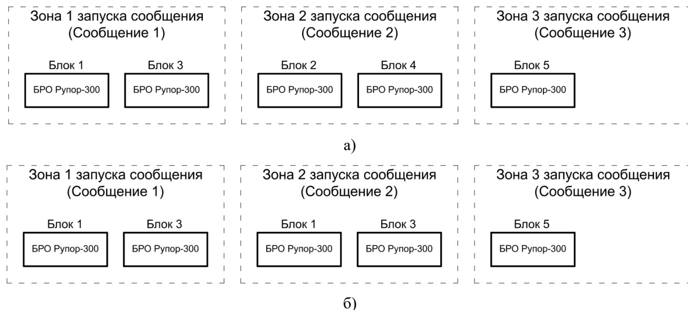
Рисунок 2.2.21. Примеры корректного создания зон запуска сообщения.
