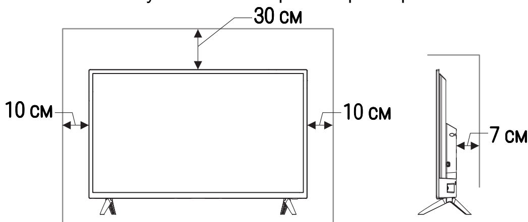
Рисунок 4.2 – Установка
