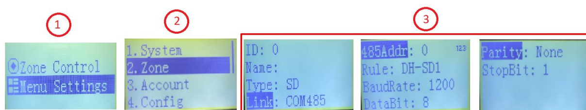
Рисунок 7.4 Настройка контрольной точки через RS-485
