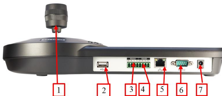
Рисунок 4.2 Задняя панель
