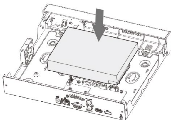
Рисунок 4.5 – Установка жесткого диска
