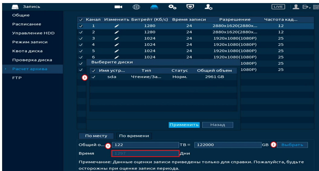
Рисунок 13.20 – Выбор диска для расчета и результат
