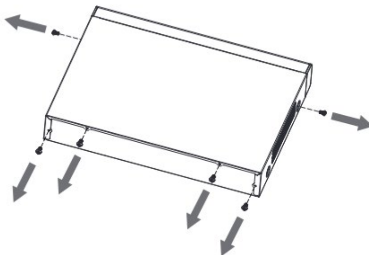
Рисунок 4.3 – Установка жесткого диска
