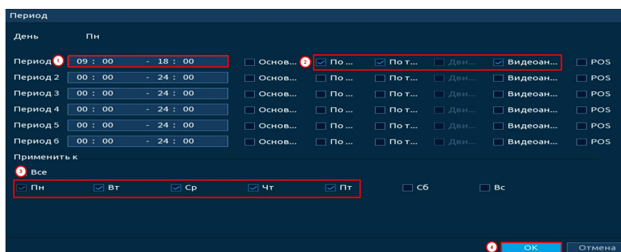
Рисунок 13.5 – Настройка расписания записи
