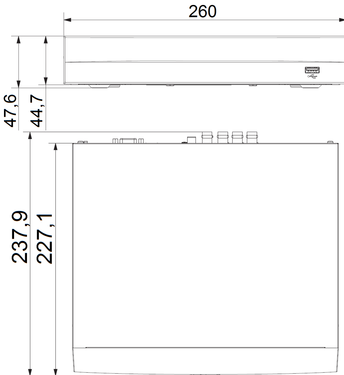
Рисунок 4.2 – Габаритные размеры
