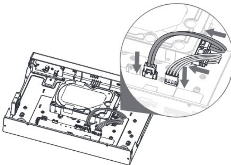
Рисунок 4.7 – Установка жесткого диска
