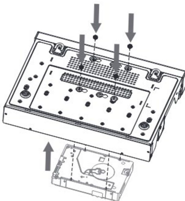
Рисунок 4.6 – Установка жесткого диска
