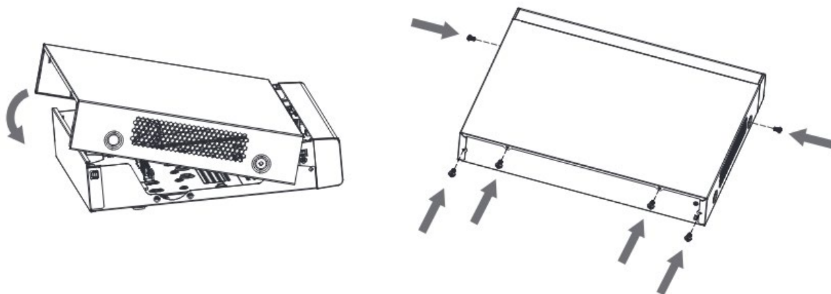
Рисунок 4.8 – Установка жесткого диска
