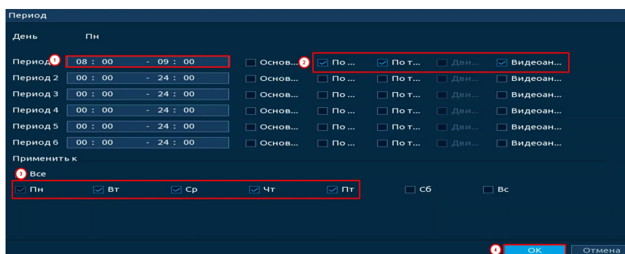
Рисунок 13.10 – Настройка расписания записи
