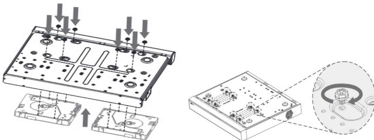
Рисунок 4.5 – Установка жёсткого диска
