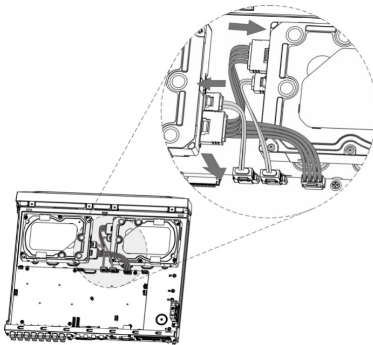
Рисунок 4.6 – Установка жёсткого диска
