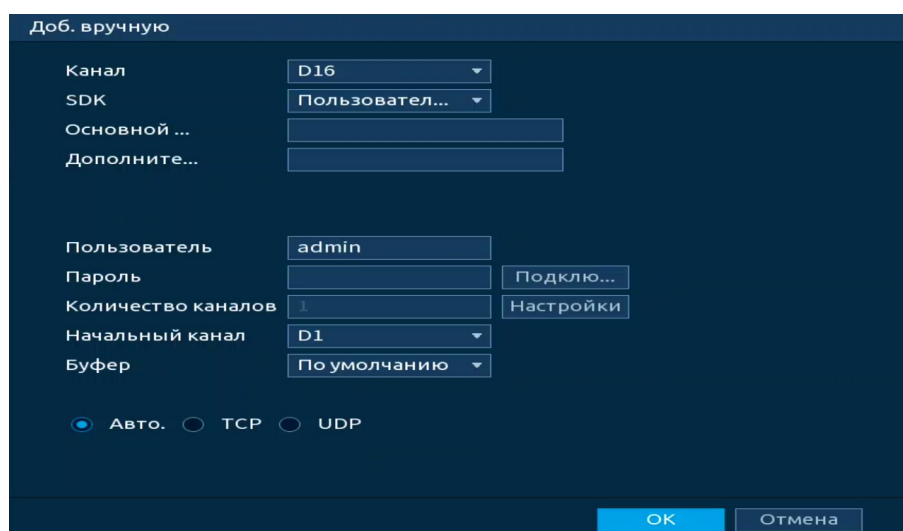
Рисунок 11.26 – Подключение к стороннему RTSP потоку
