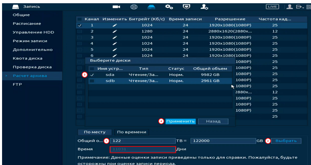
Рисунок 13.25 – Выбор диска для расчёта и результат
