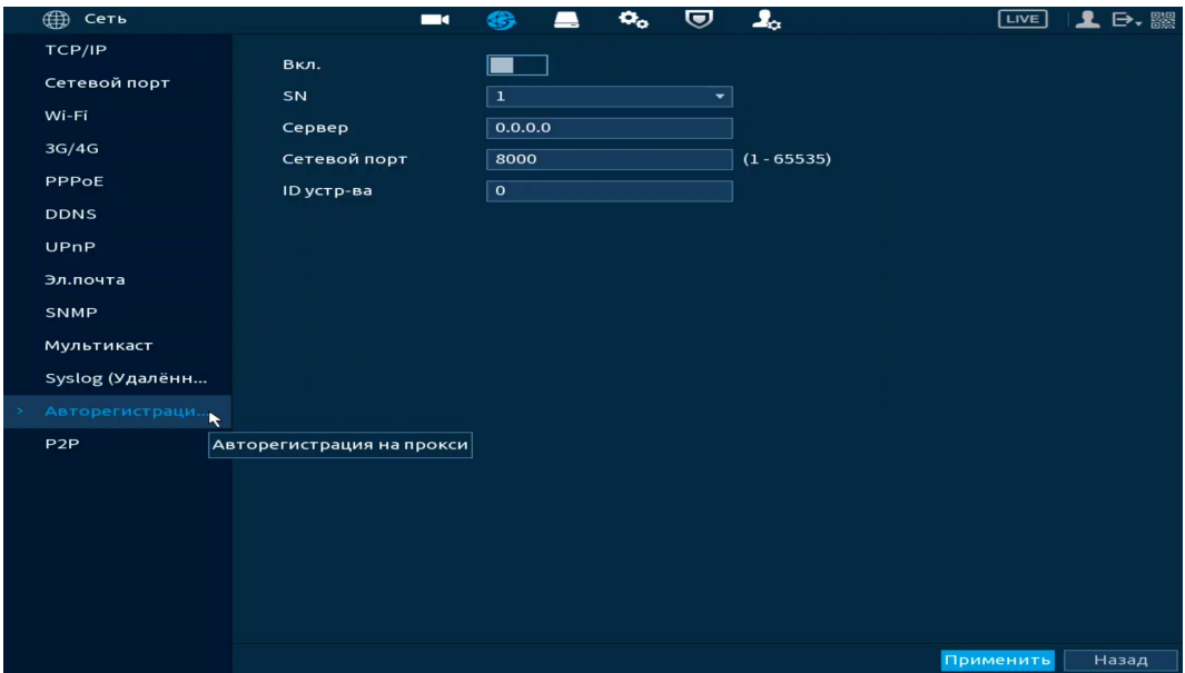
Рисунок 12.14 – Интерфейс настройки «Авторегистрация на прокси»
