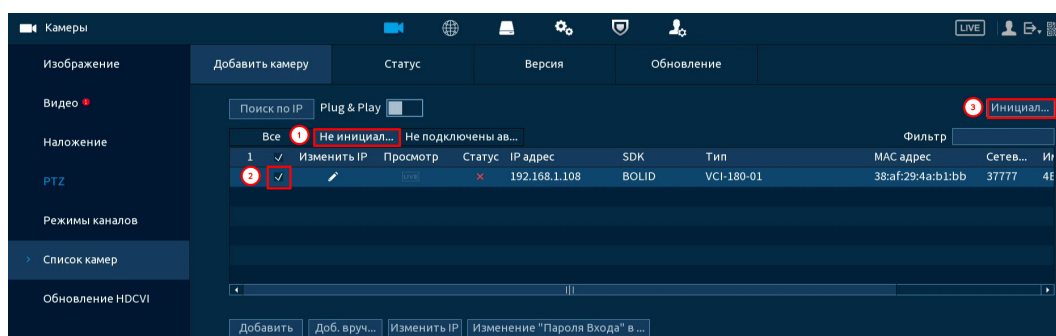
Рисунок 11.19 – Инициализация устройства
