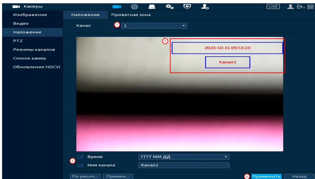
Рисунок 11.8 – Наложенные параметры
