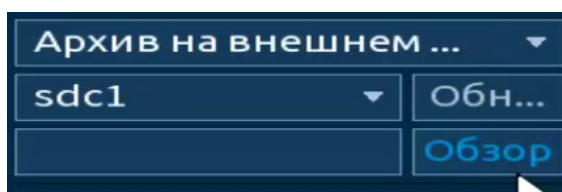
Рисунок 17.16 – Тип поиска
