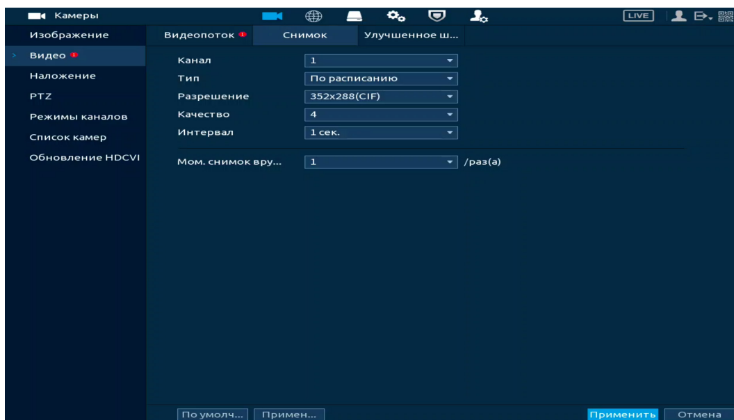
Рисунок 11.6 – Настройка снимка
