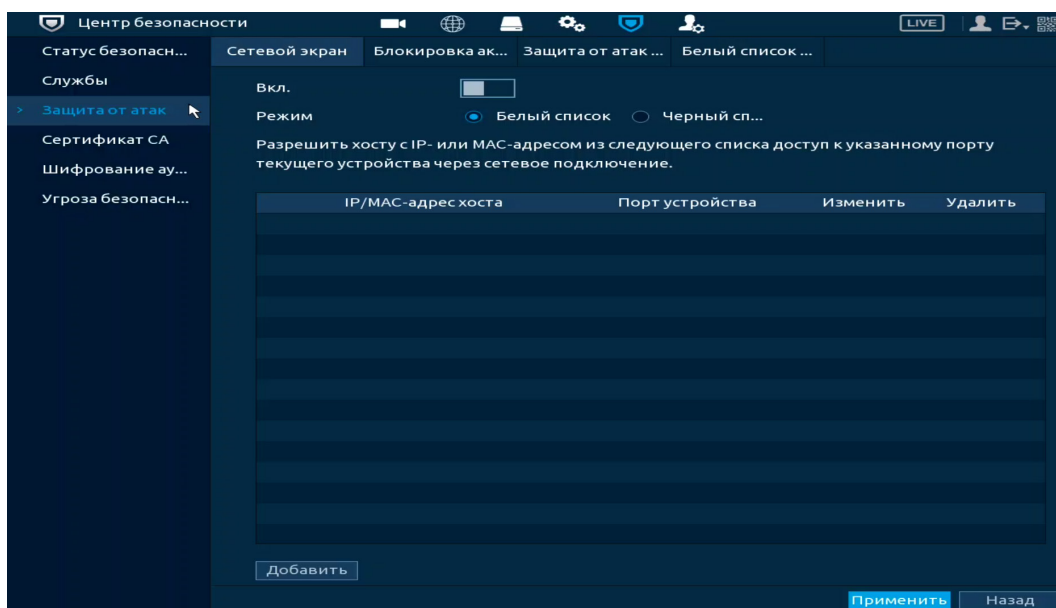
Рисунок 15.7 – Сетевой экран
