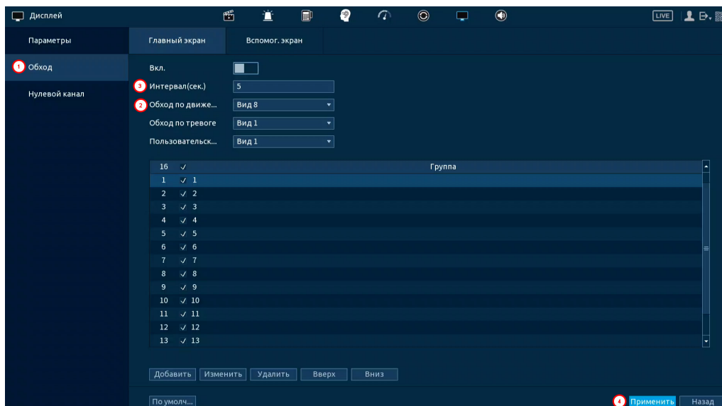
Рисунок 23.4 – Пример настройки
