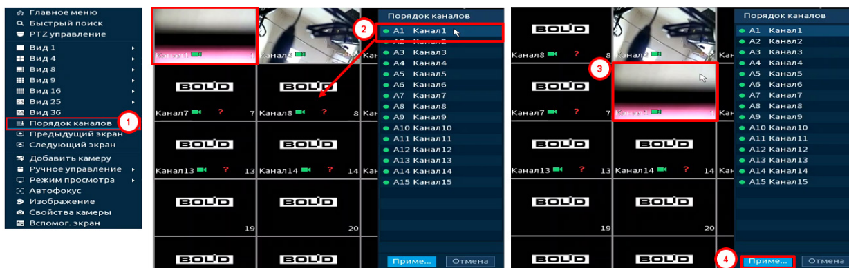
Рисунок 7.7 – Изменение раскладки
