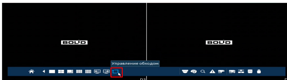
Рисунок 23.12 – Выключение/включение обхода
