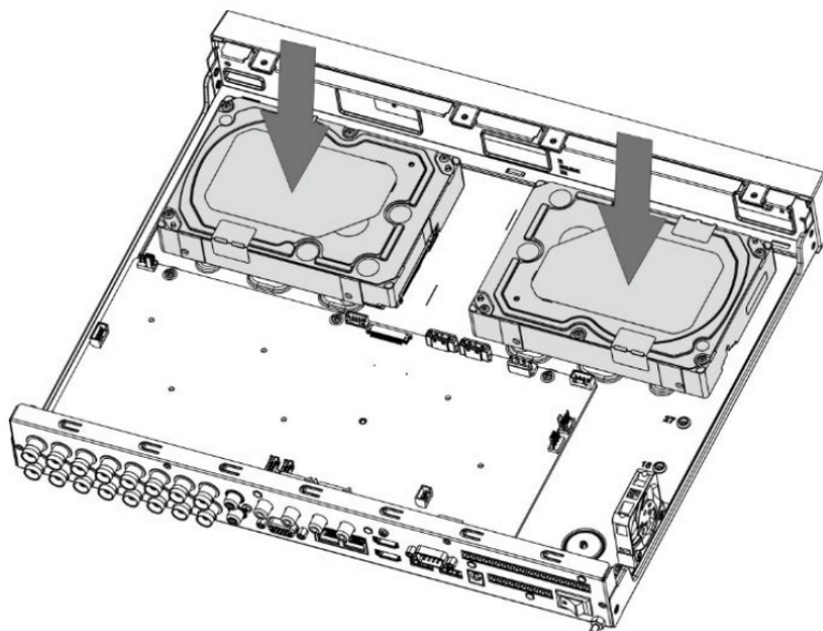
Рисунок 4.4 – Установка жёсткого диска
