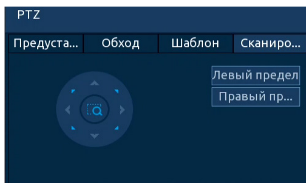
Рисунок 8.11 – Интерфейс «Сканирование»
