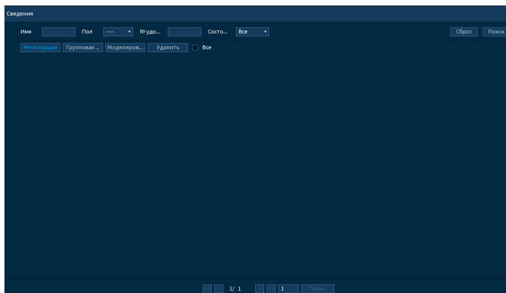
Рисунок 20.43 – Настройка
