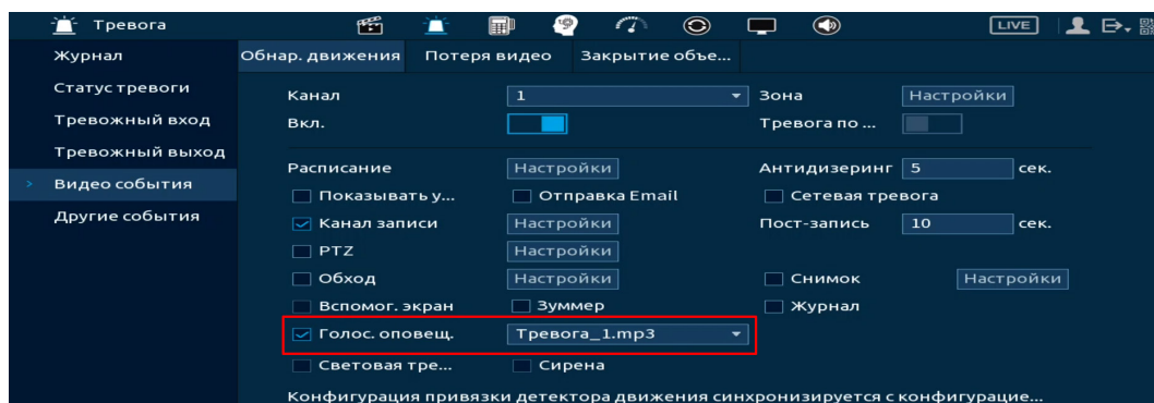
Рисунок 24.2 – Пример применения
