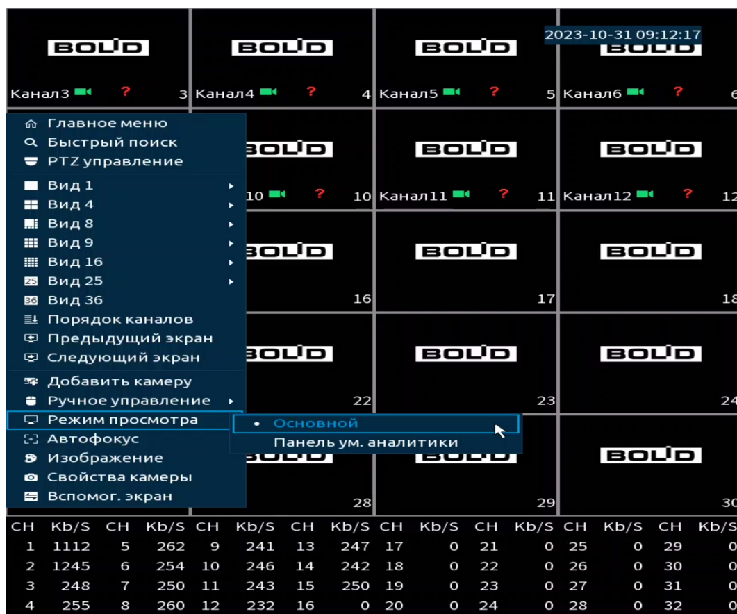
Рисунок 7.9 – Режим просмотра «Основной»
