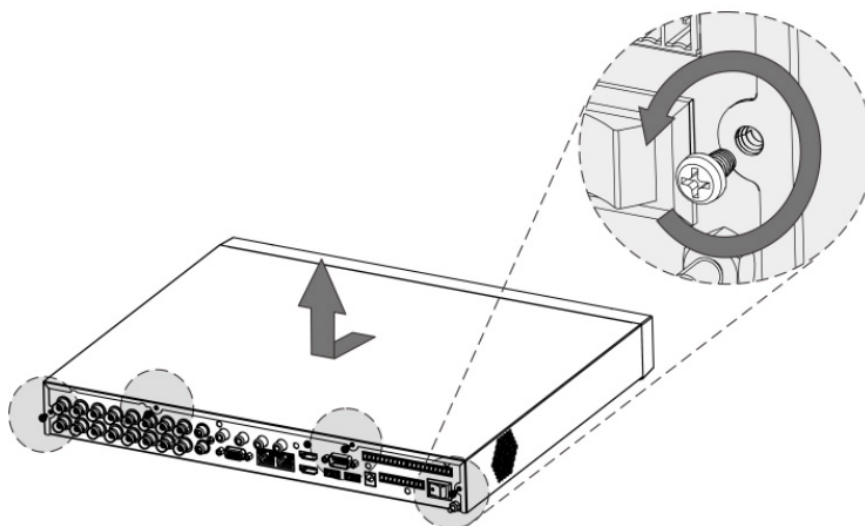
Рисунок 4.3 – Установка жёсткого диска
