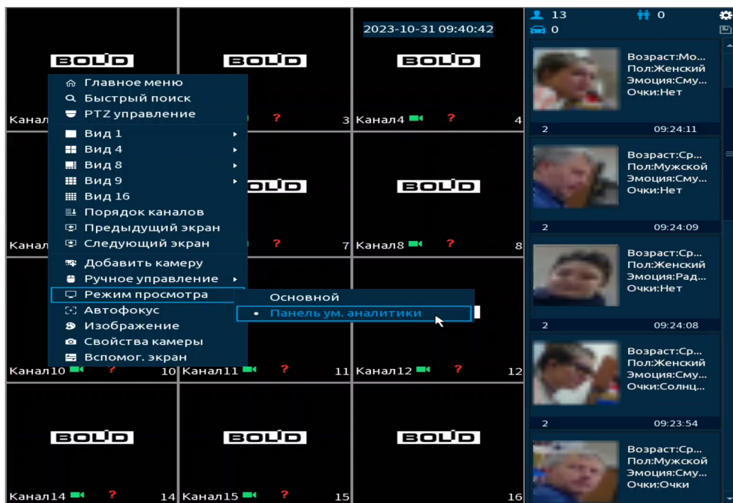
Рисунок 7.10 – Режим просмотра «Панель ум. аналитики»
