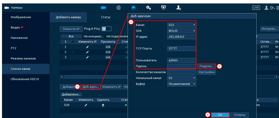
Рисунок 11.25 – Интерфейс ручного добавления удалённого устройства
