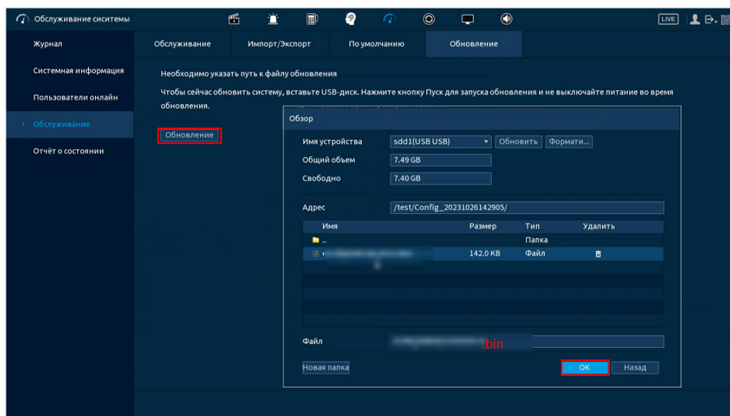
Рисунок 21.17 – Выбор файла для обновления
