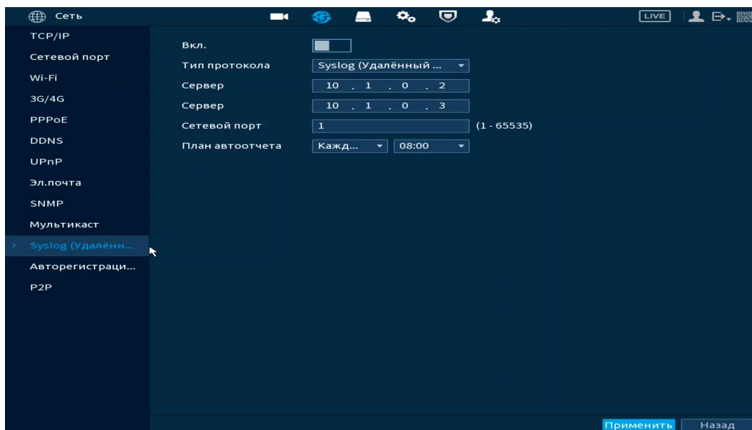
Рисунок 12.13 – Интерфейс настройки «Syslog (Удалённый журнал)»
