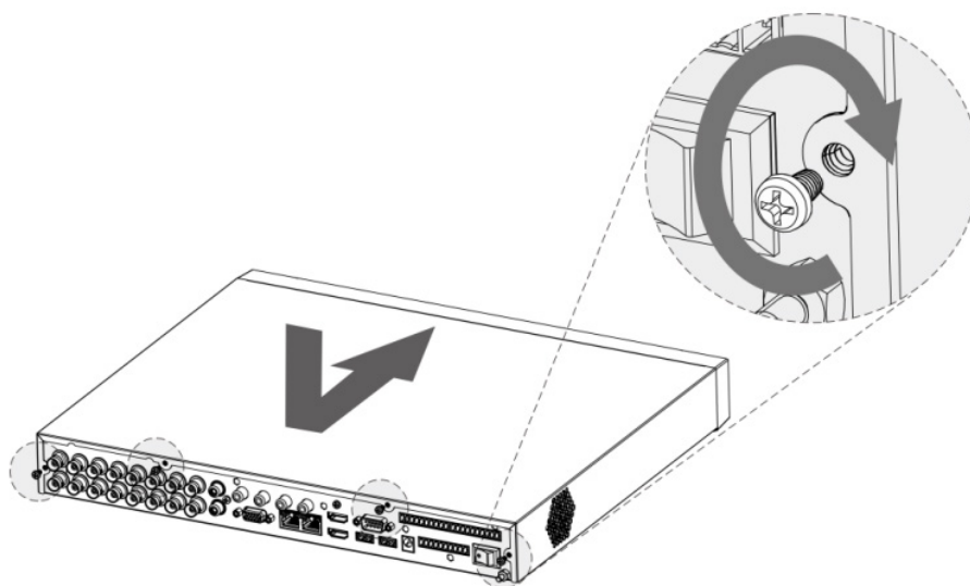
Рисунок 4.7 – Установка жёсткого диска
