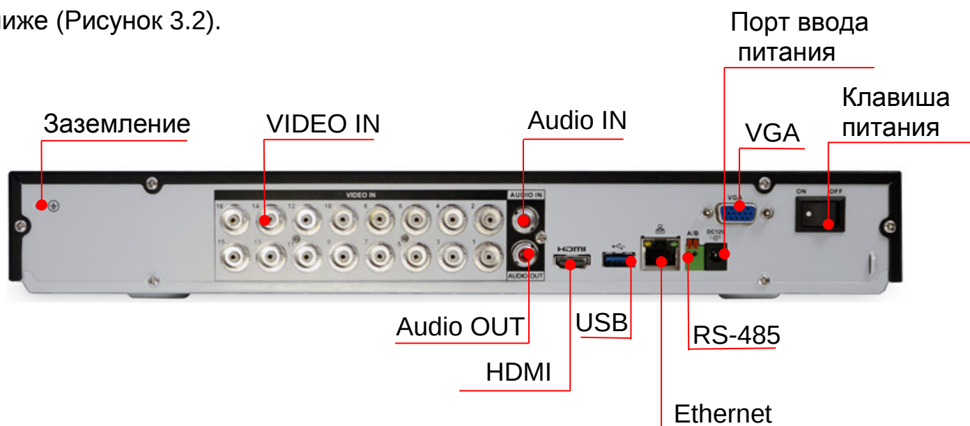
Рисунок 3.2 – Внешний вид задней панели
