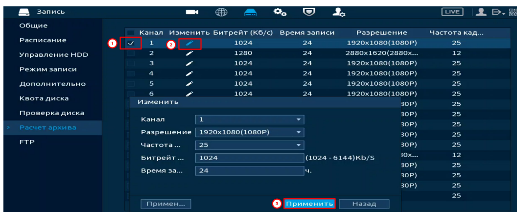
Рисунок 13.24 – Расчёт времени. Выбор канала
