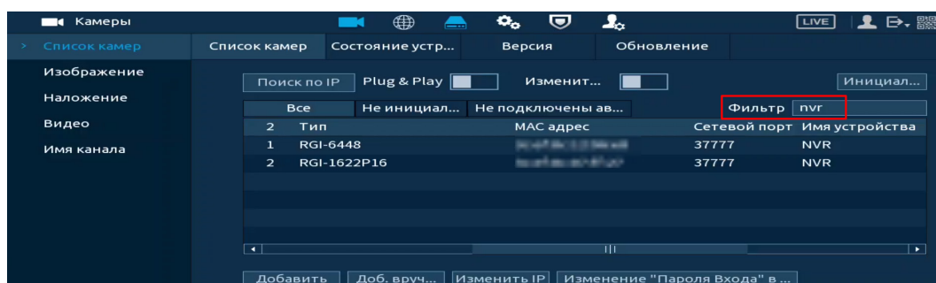
Рисунок 10.7 – Фильтр
