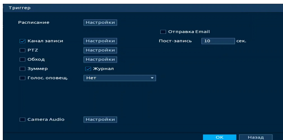
Рисунок 18.31 – Настройка параметров
