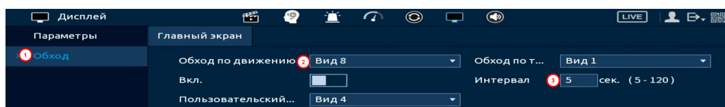
Рисунок 21.3 – Пример настройки
