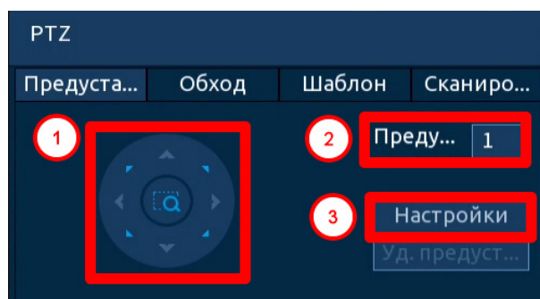
Рисунок 8.3 – PTZ предустановка
