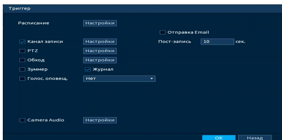
Рисунок 18.49 – Настройка параметров
