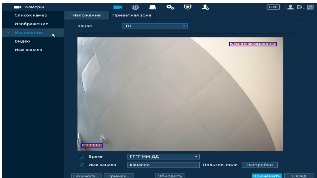
Рисунок 10.31 – Наложенные параметры
