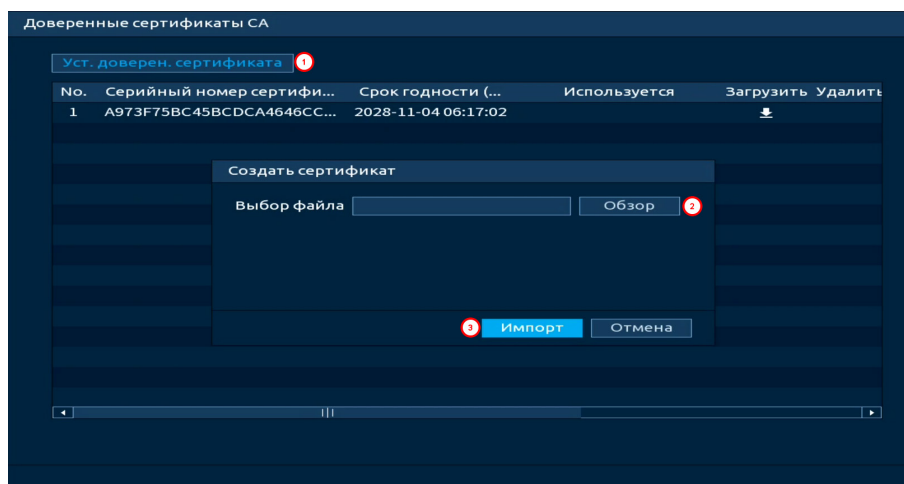
Рисунок 14.4 – Импорт
