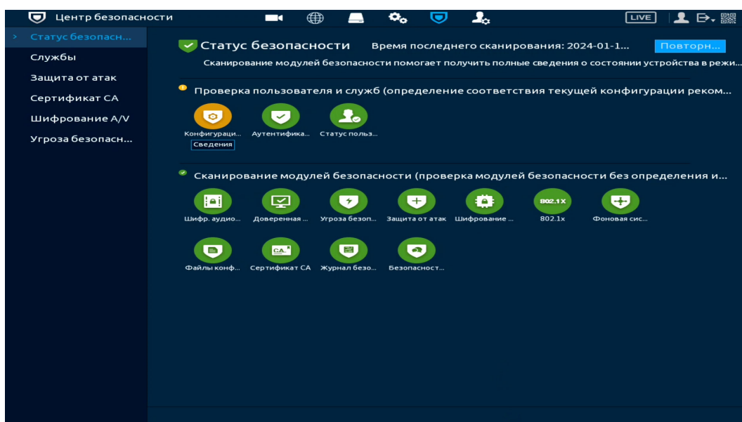
Рисунок 14.1 – Статус безопасности
