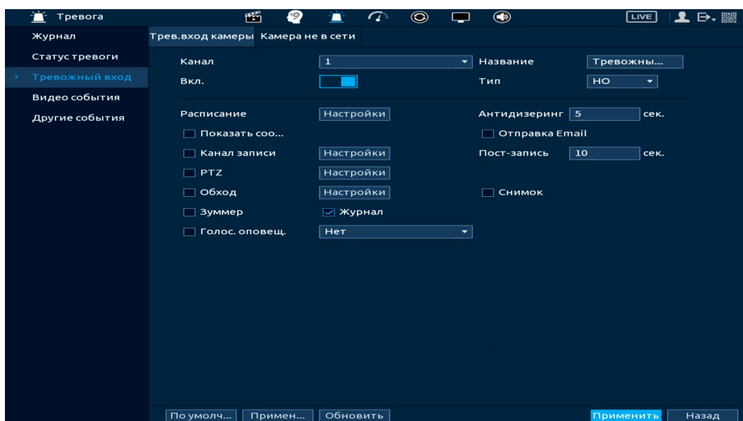
Рисунок 17.3 – Интерфейс настройки
