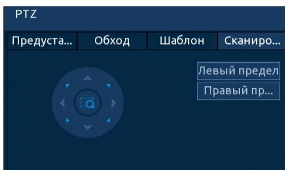
Рисунок 8.10 – Интерфейс «Сканирование»
