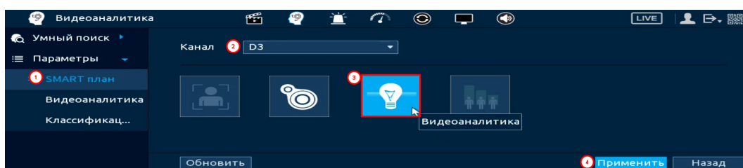
Рисунок 18.22 – Настройка
