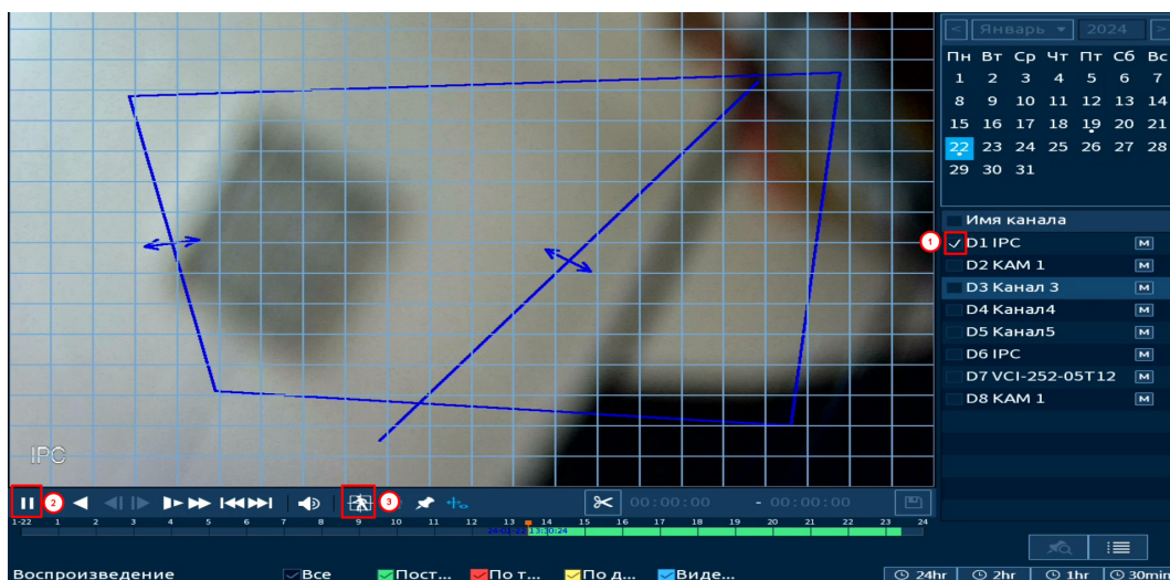
Рисунок 16.6– Настройка
