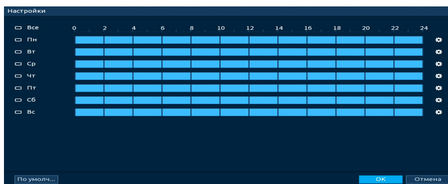
Рисунок 18.53 – Расписание
