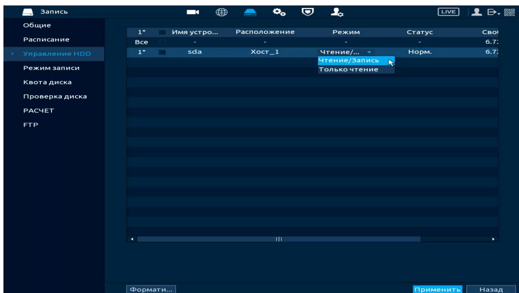
Рисунок 12.14 – Интерфейс настройки
