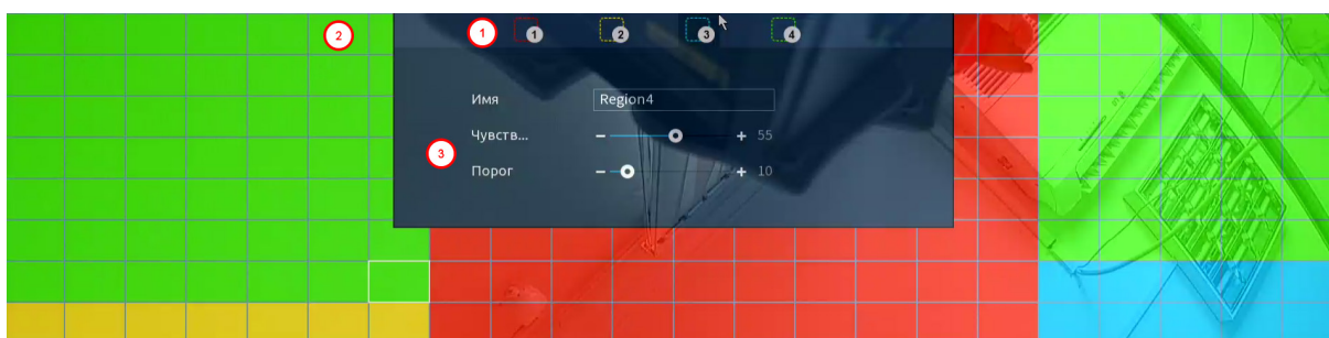
Рисунок 17.9 – Настройка области
