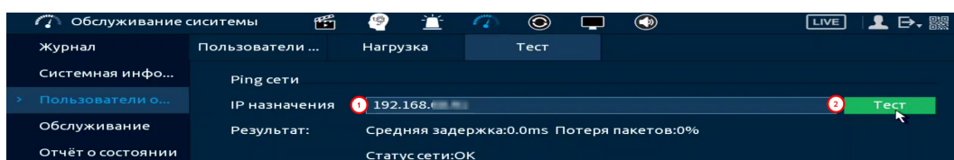
Рисунок 19.7 – Проверка IP-адреса
