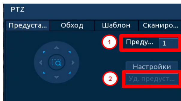
Рисунок 8.6 – PTZ предустановка
