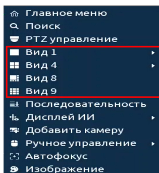
Рисунок 7.1 – Контекстное меню
