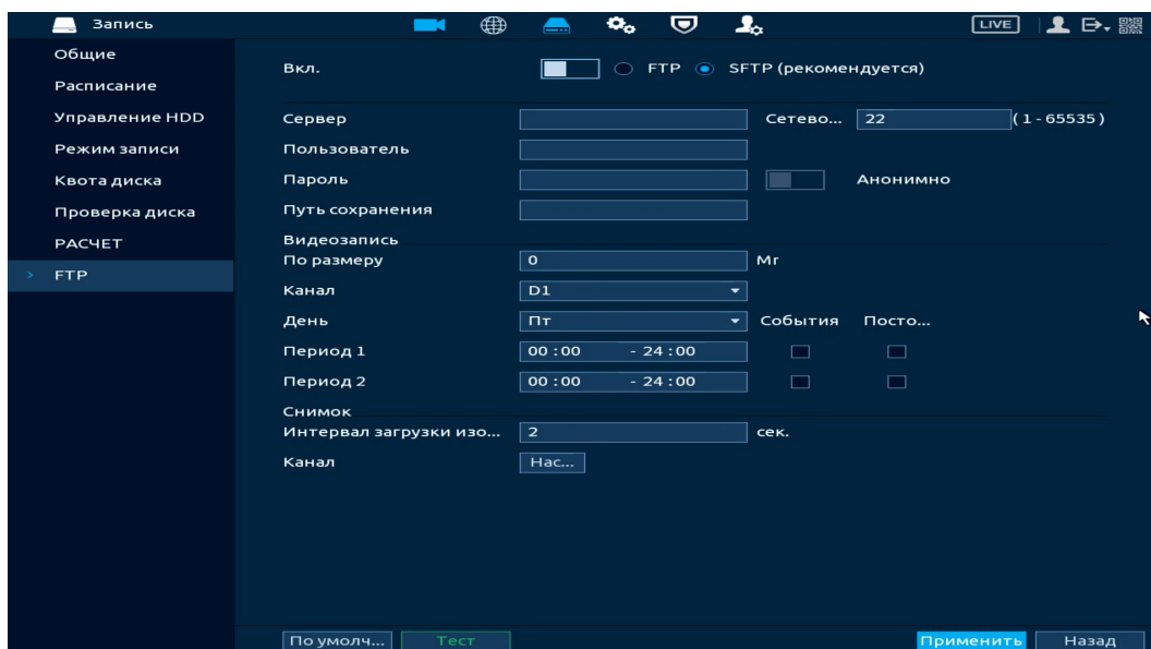
Рисунок 12.24 – Настройка FTP
