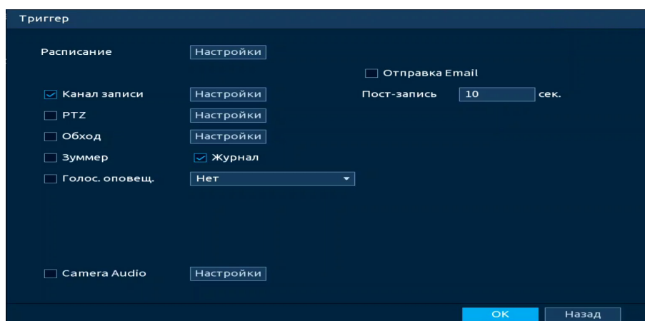
Рисунок 18.25 – Настройка параметров
