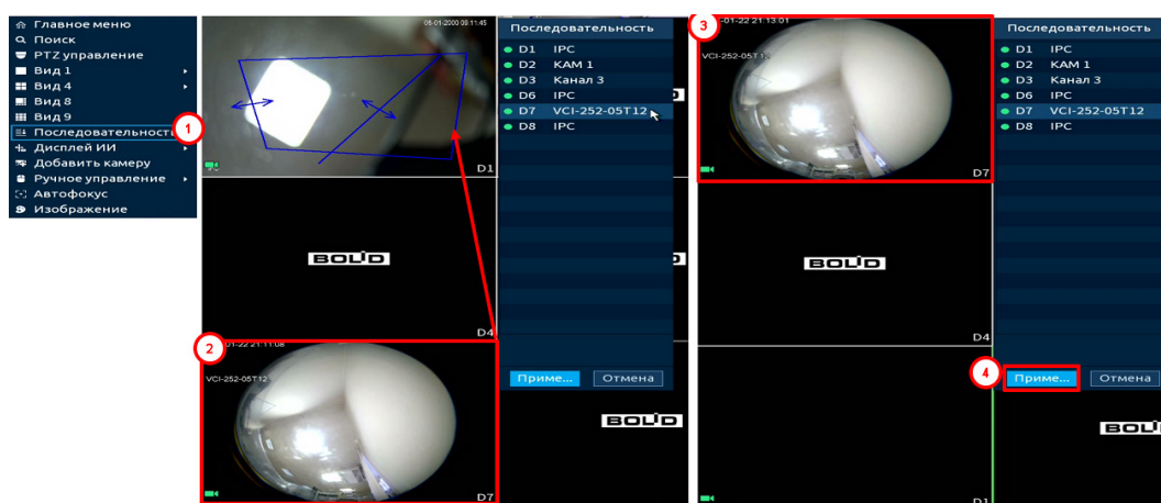
Рисунок 7.5 – Изменение раскладки
