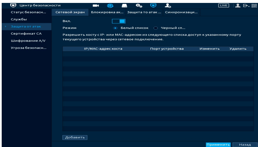
Рисунок 14.8 – Сетевой экран
