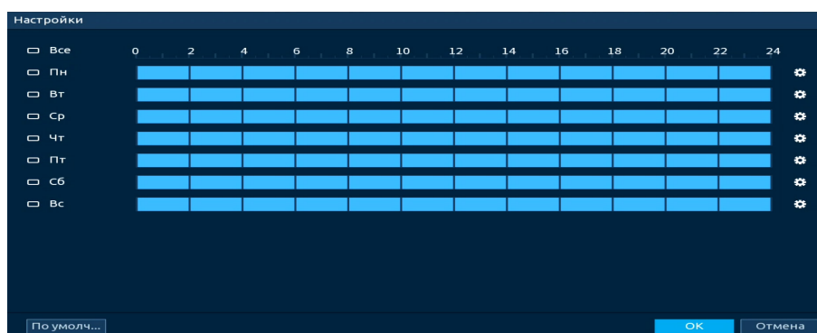
Рисунок 18.50 – Расписание
