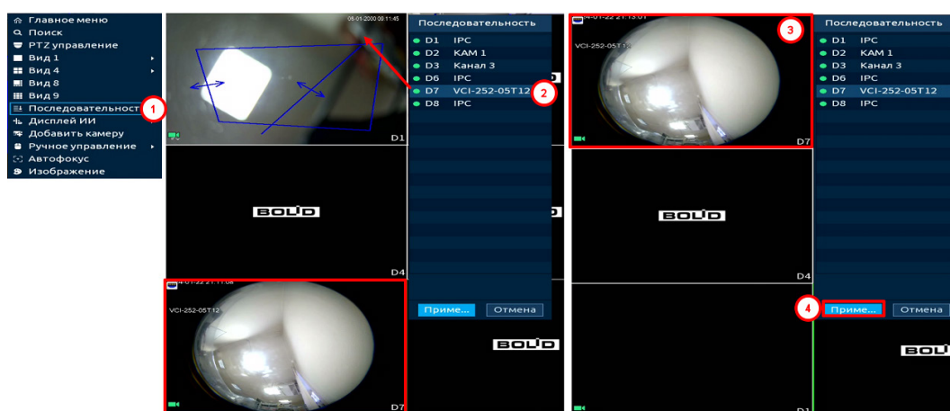
Рисунок 7.4 – Изменение раскладки
