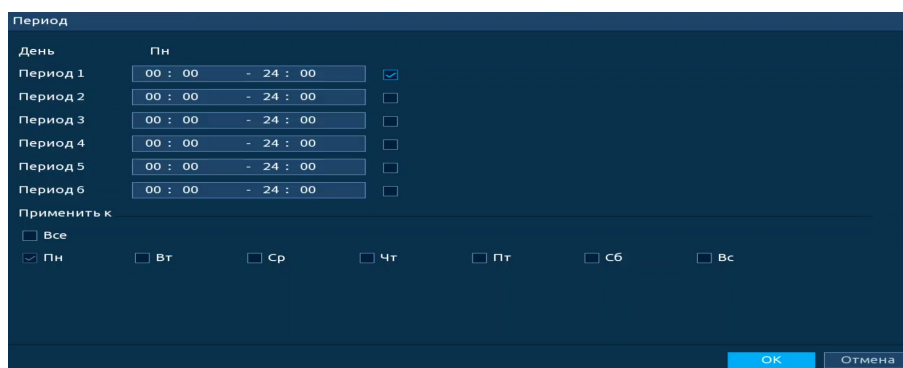
Рисунок 17.19 – Расписание
