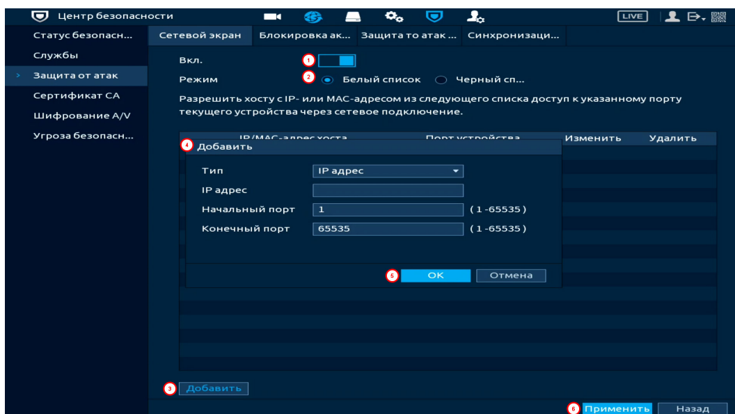
Рисунок 14.9 – Добавить
