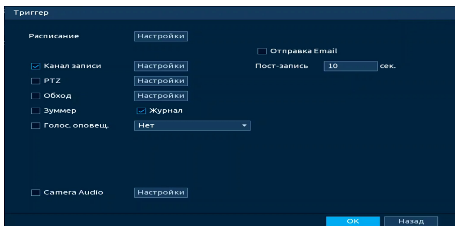
Рисунок 18.43 – Настройка параметров
