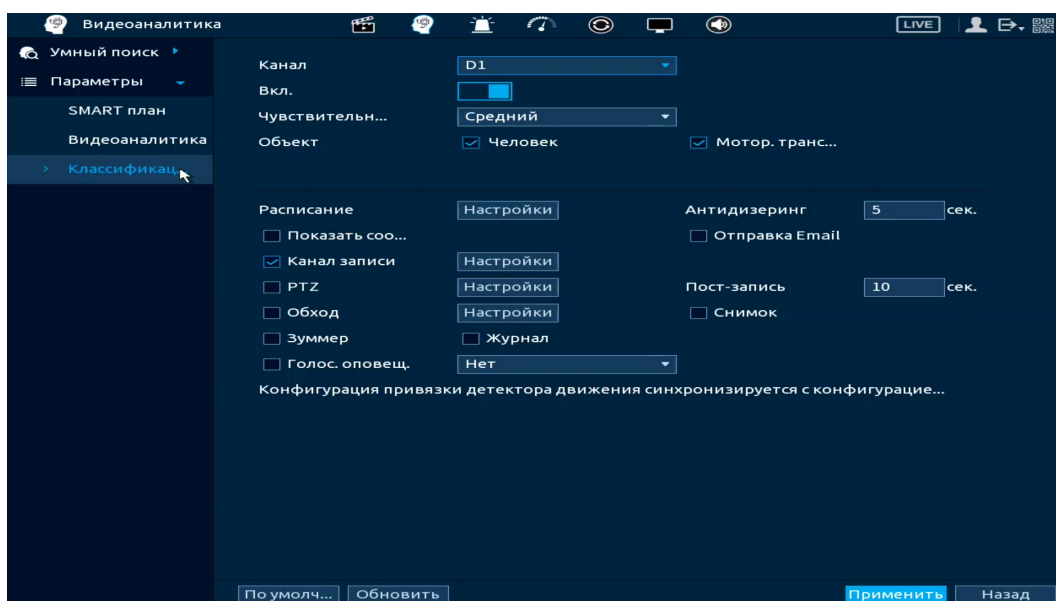
Рисунок 18.52 – Классификация объектов
