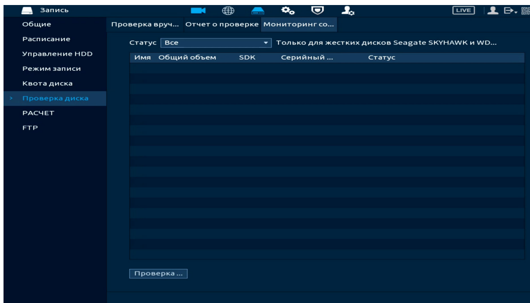
Рисунок 12.19 – Мониторинг состояния
