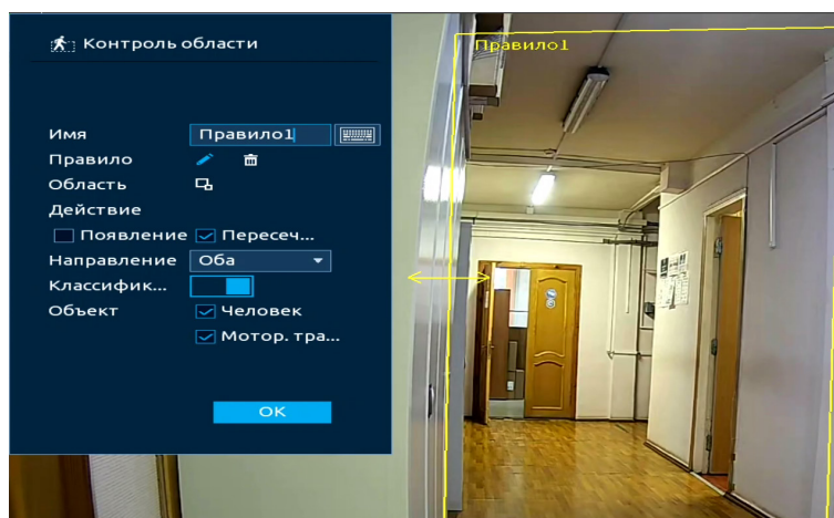
Рисунок 18.12 – Настройка правила
