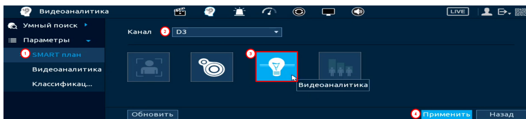
Рисунок 18.46 – Настройка
