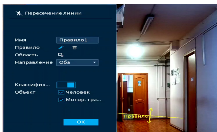
Рисунок 18.6 – Настройка правила
