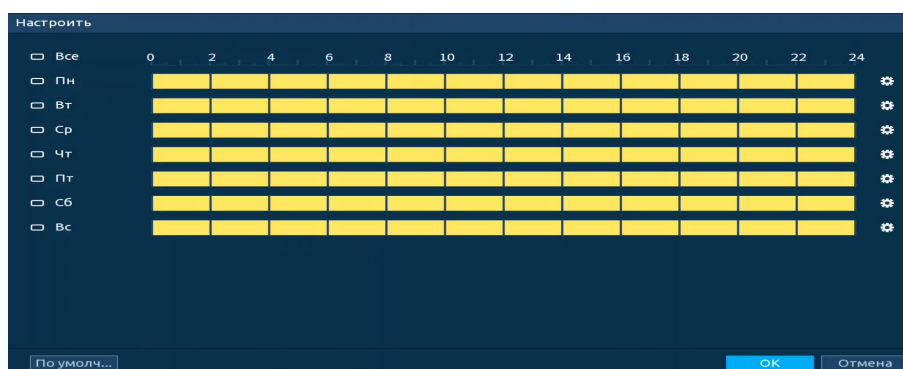
Рисунок 17.18 – Панель расписания
