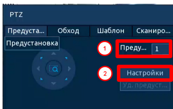
Рисунок 8.5 – PTZ предустановка
