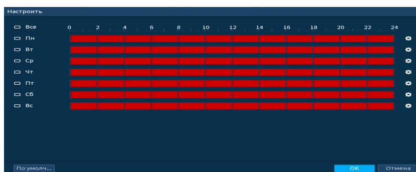
Рисунок 17.4 – Панель расписания
