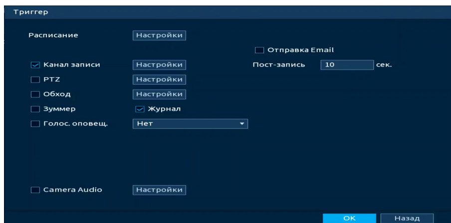
Рисунок 18.13 – Настройка параметров
