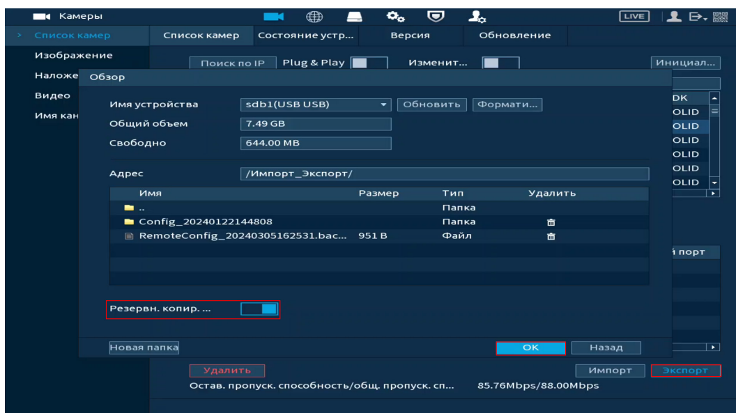
Рисунок 10.21 – Экспорт
