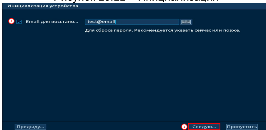
Рисунок 10.12 – Инициализация
