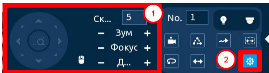
Рисунок 8.4 – PTZ предустановка
