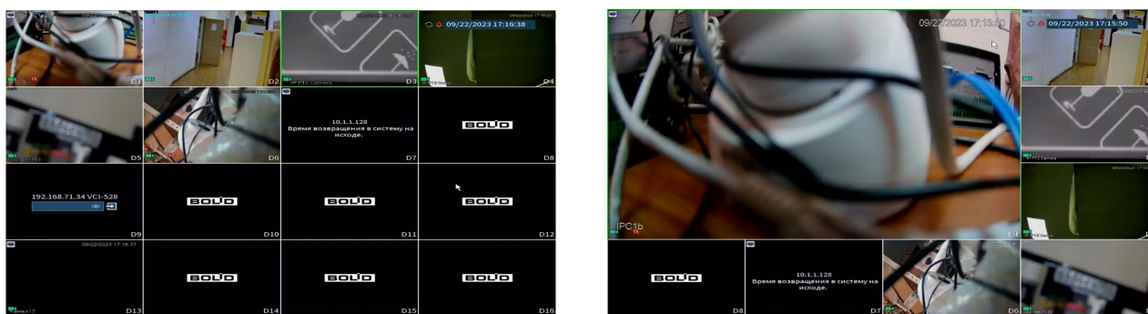
Рисунок 21.5 – Пример настройки
