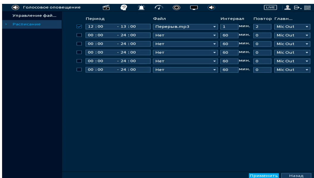
Рисунок 22.4 – Расписание
