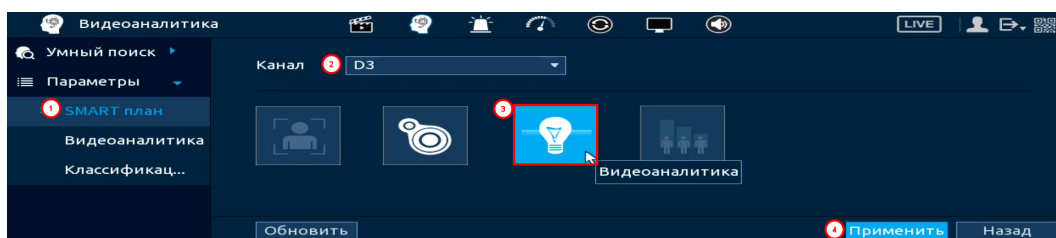
Рисунок 18.16 – Настройка
