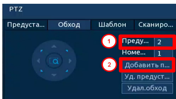
Рисунок 8.8 – Обход
