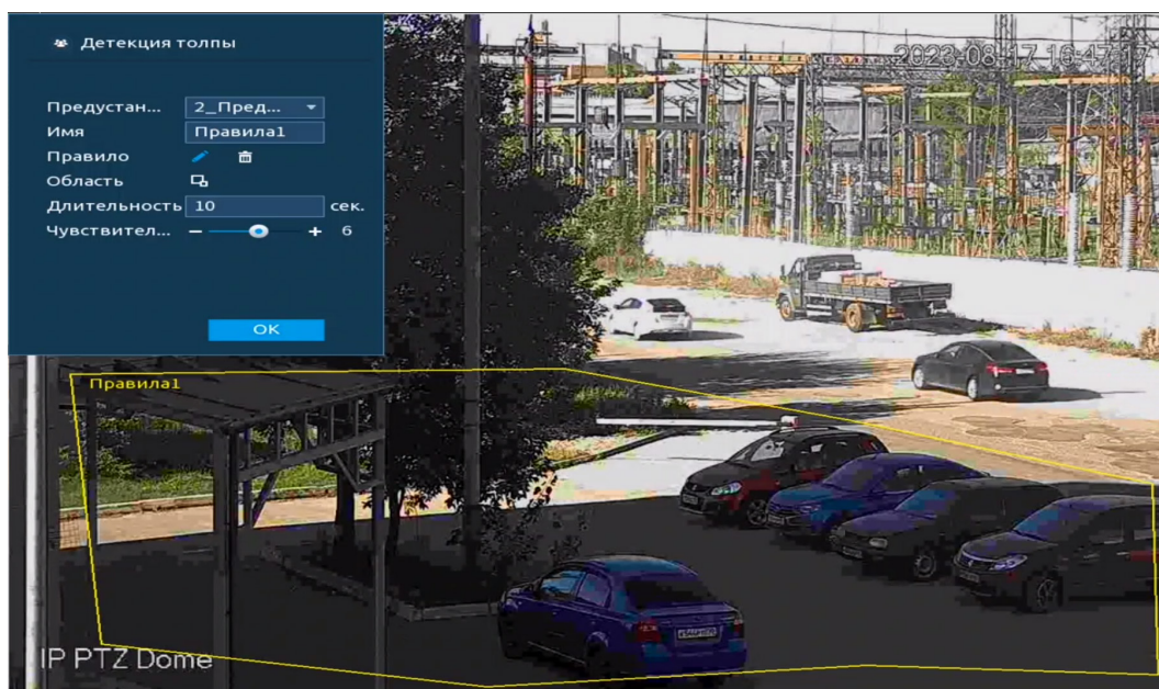
Рисунок 18.42 – Настройка правила
