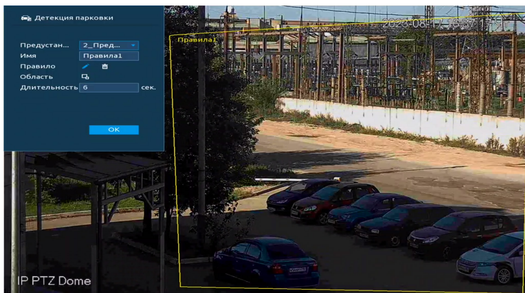
Рисунок 18.36 – Настройка правила
