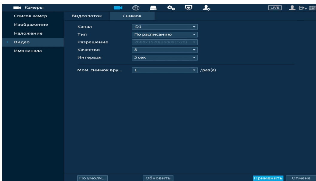
Рисунок 10.30 – Настройка снимка
