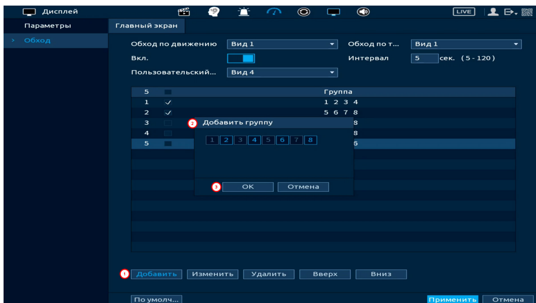
Рисунок 21.9 – Добавление группы
