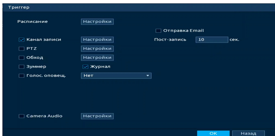
Рисунок 18.37 – Настройка параметров
