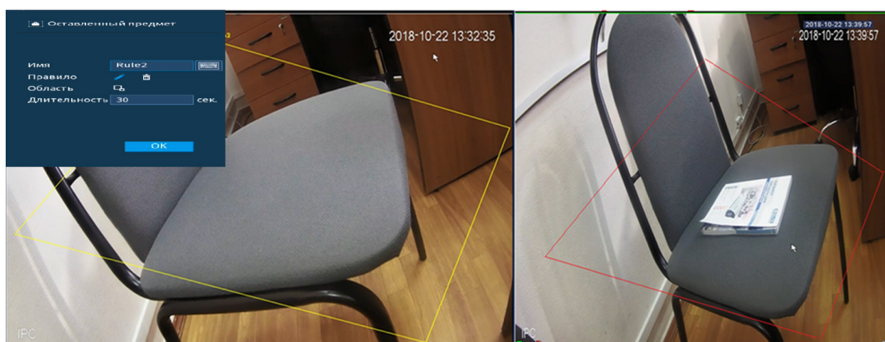
Рисунок 18.18 – Настройка функции
