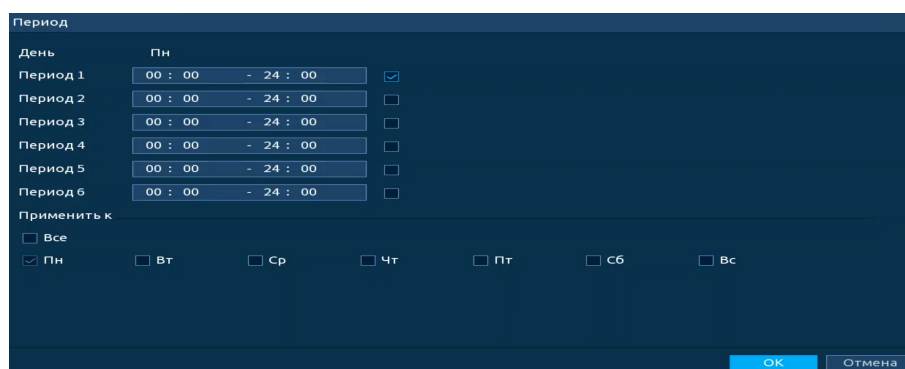
Рисунок 17.5 – Расписание
