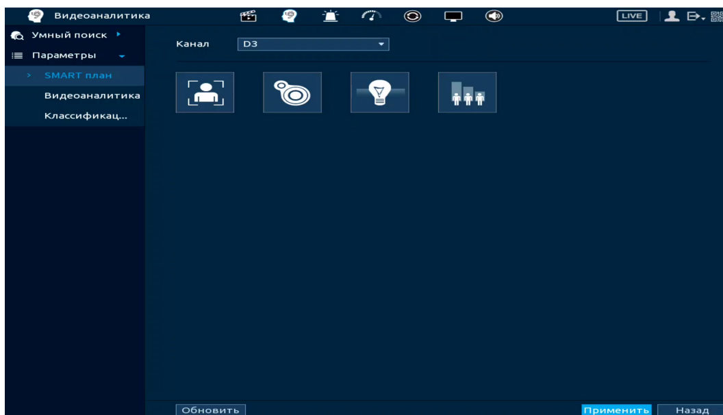
Рисунок 18.3 – Выбор функции
