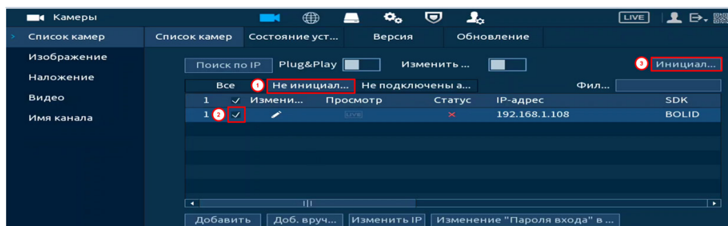
Рисунок 10.9 – Инициализация устройства
