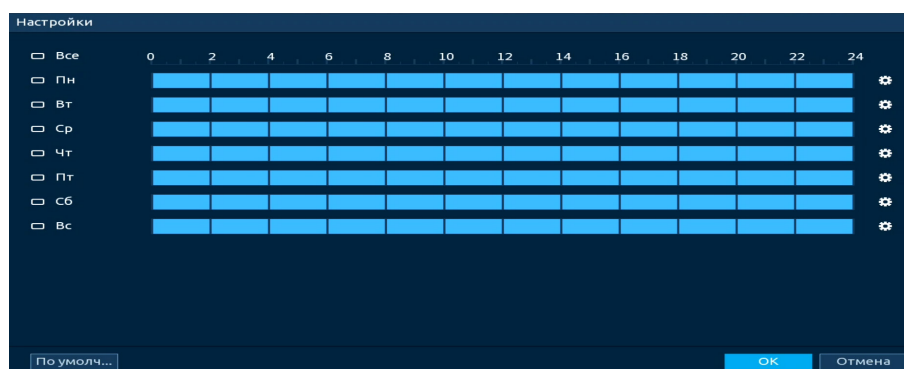
Рисунок 18.38 – Расписание
