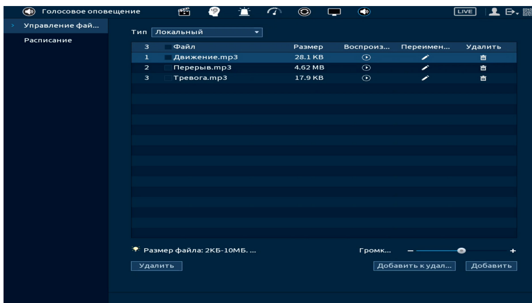
Рисунок 22.1 – Управление файлами
