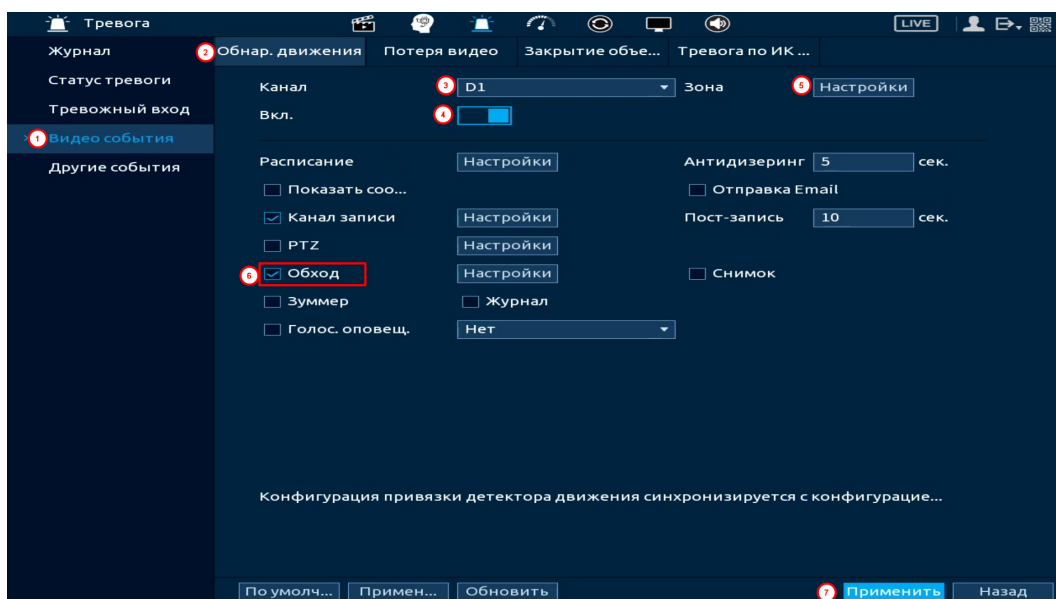
Рисунок 21.4 – Пример настройки
