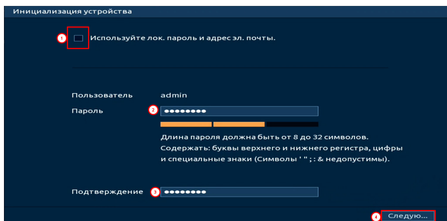
Рисунок 10.11 – Инициализация
