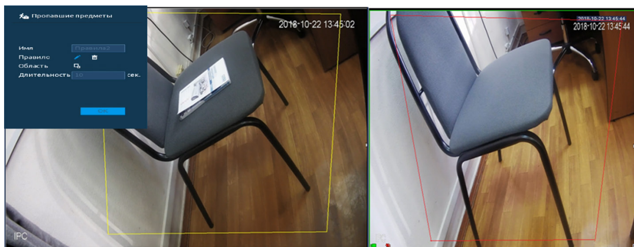
Рисунок 18.24 – Настройка функции
