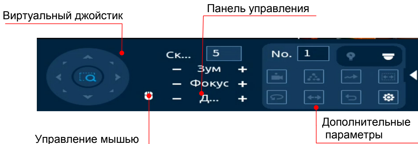
Рисунок 8.2 – Панель PTZ-управления
