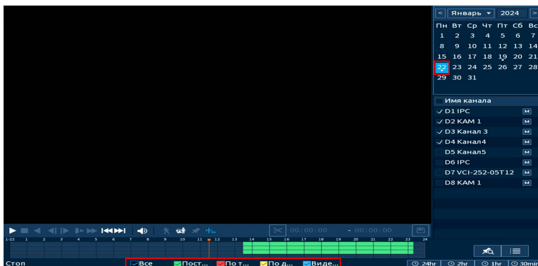
Рисунок 16.4 – Шкала времени
