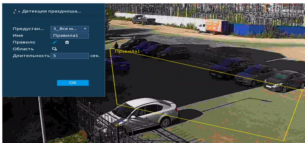
Рисунок 18.48 – Настройка правила
