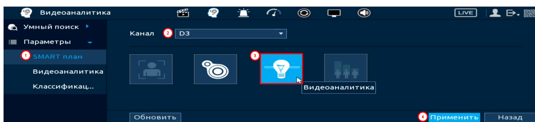
Рисунок 18.28 – Настройка
