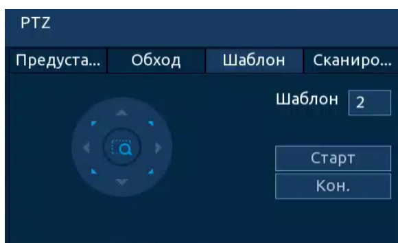
Рисунок 8.9 – Интерфейс «Шаблон»
