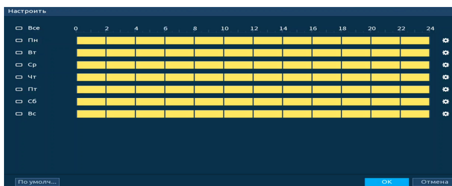
Рисунок 17.10 – Расписание
