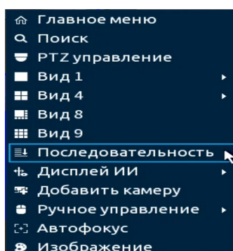
Рисунок 7.3 – Контекстное меню
