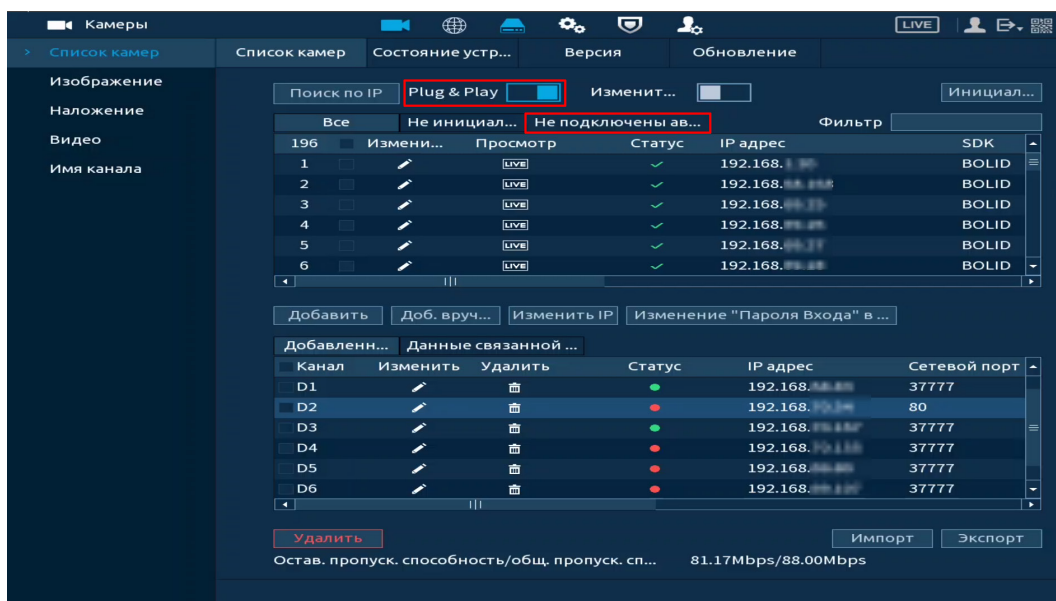
Рисунок 10.5 – Plug&amp;Play
