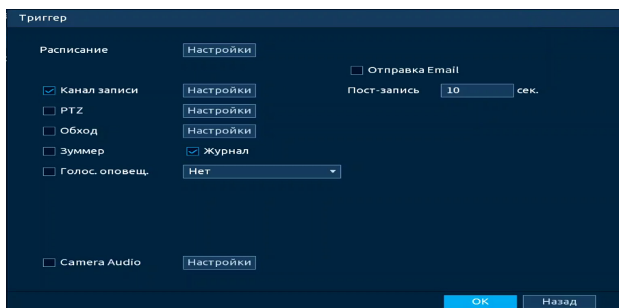
Рисунок 18.7 – Настройка параметров
