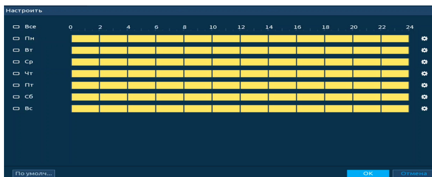
Рисунок 17.14 – Панель расписания
