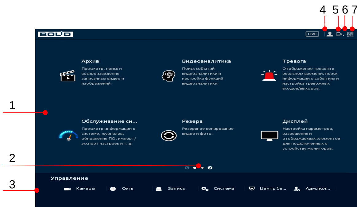
Рисунок 9.1 – Главное меню
