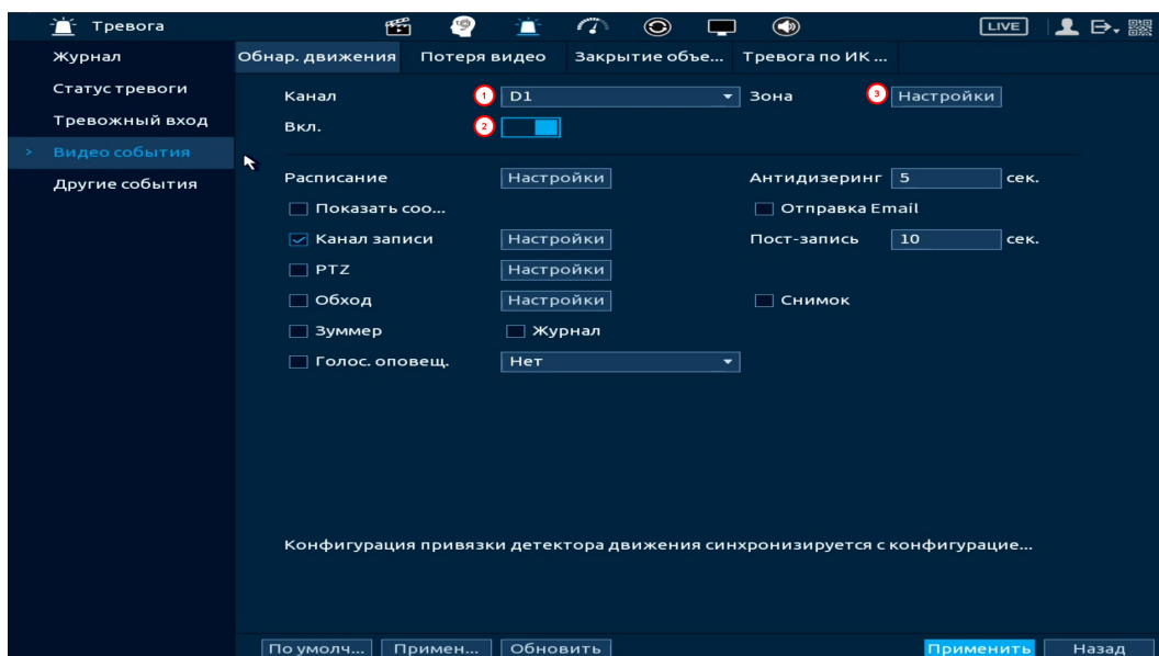
Рисунок 17.8 – Настройка события
