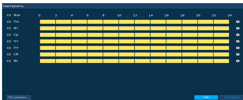
Рисунок 17.22 – Панель расписания
