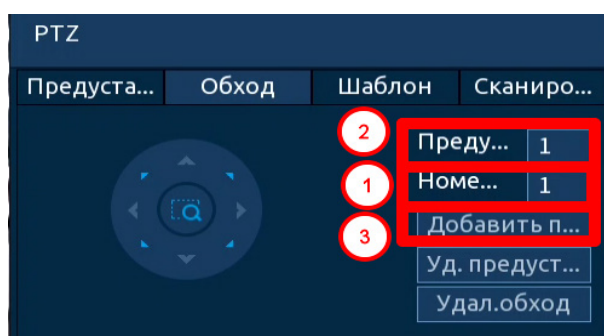
Рисунок 8.7 – Обход
