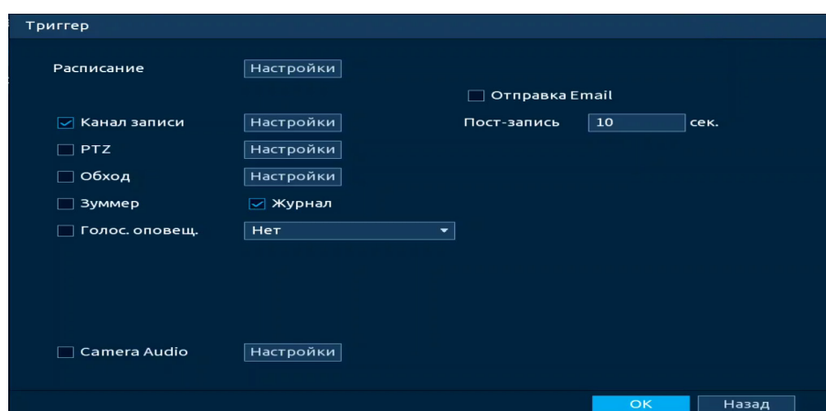
Рисунок 18.19 – Настройка параметров
