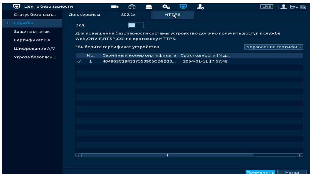
Рисунок 14.5 – HTTPS
