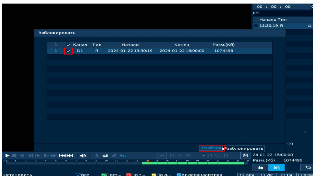
Рисунок 16.12 – Блокировка/Разблокировка файлов
