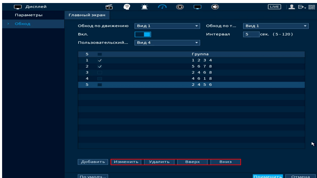
Рисунок 21.8 – Расположение групп
