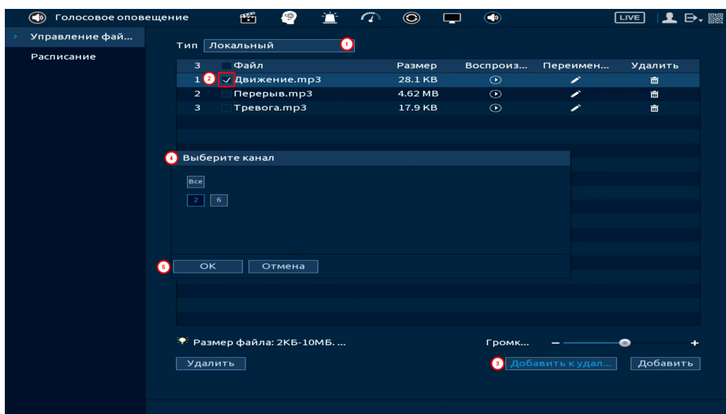
Рисунок 22.3 – Добавление
