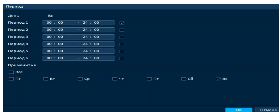
Рисунок 18.39 – Расписание
