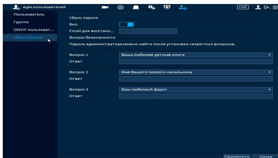
Рисунок 15.10 – Сброс пароля
