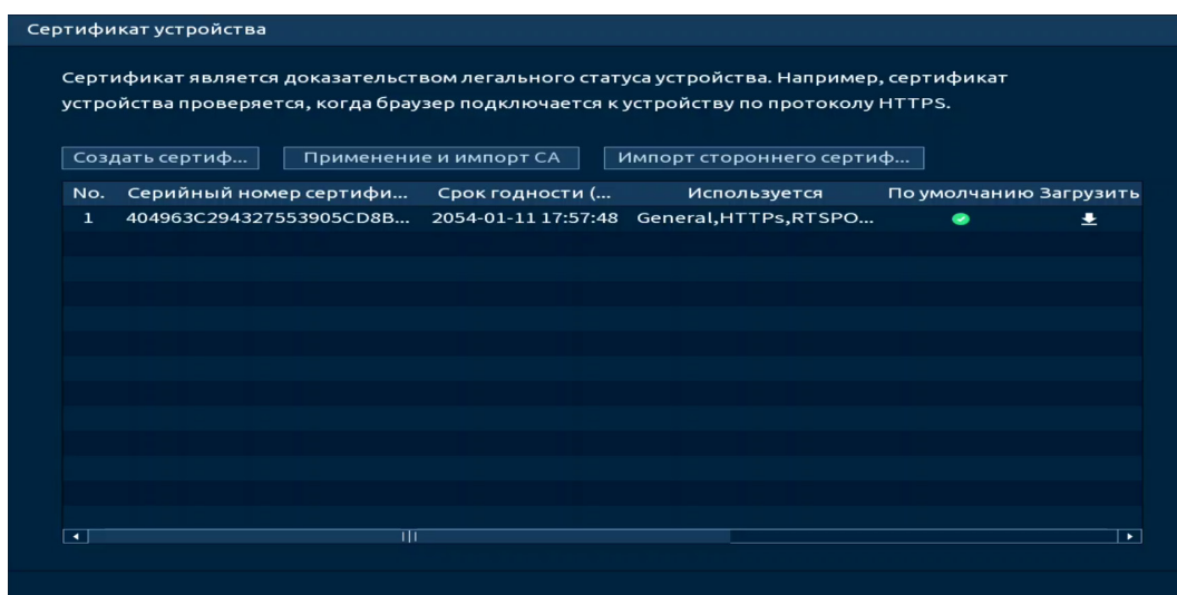
Рисунок 14.6 – Настройка
