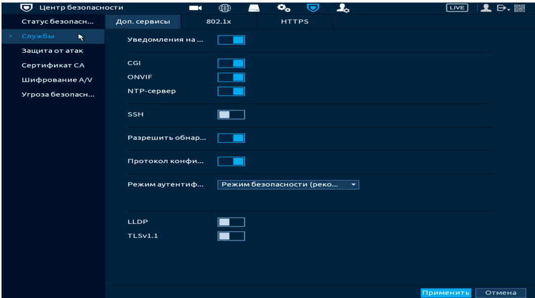
Рисунок 14.2 – Системное обслуживание
