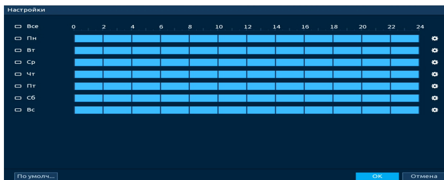
Рисунок 18.8 – Расписание
