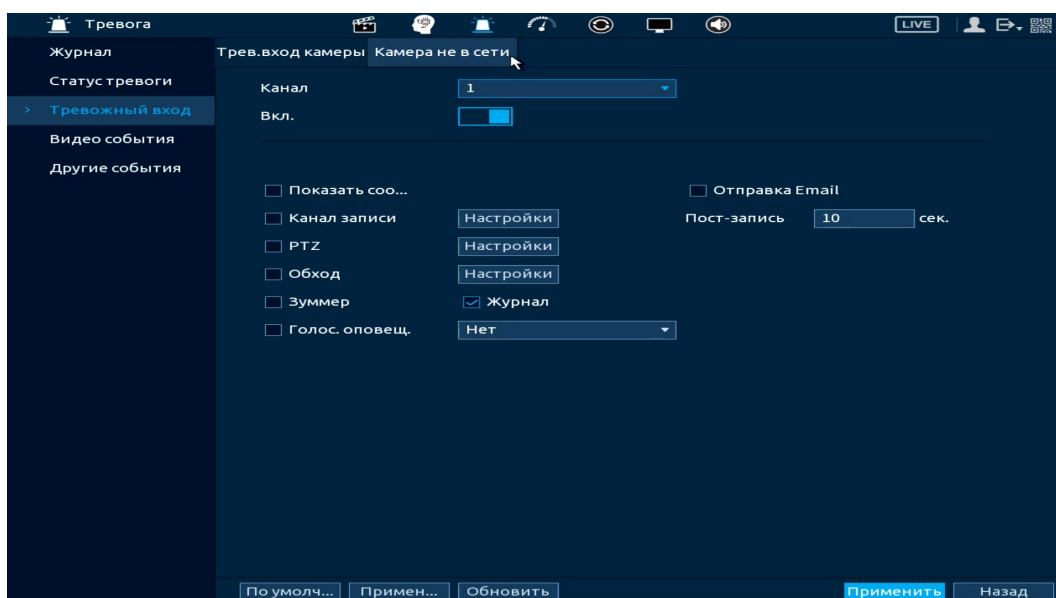
Рисунок 17.6 – Интерфейс настройки
