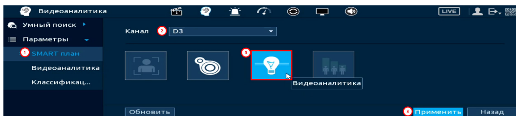
Рисунок 18.4 – Настройка
