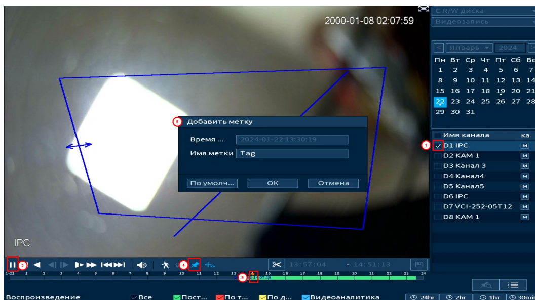
Рисунок 16.10 – Создание метки
