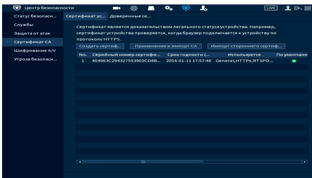
Рисунок 14.16 – Сертификат устройства
