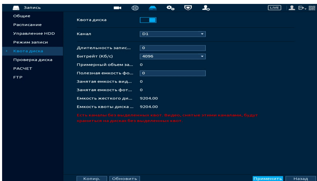
Рисунок 12.16 – Квота диска
