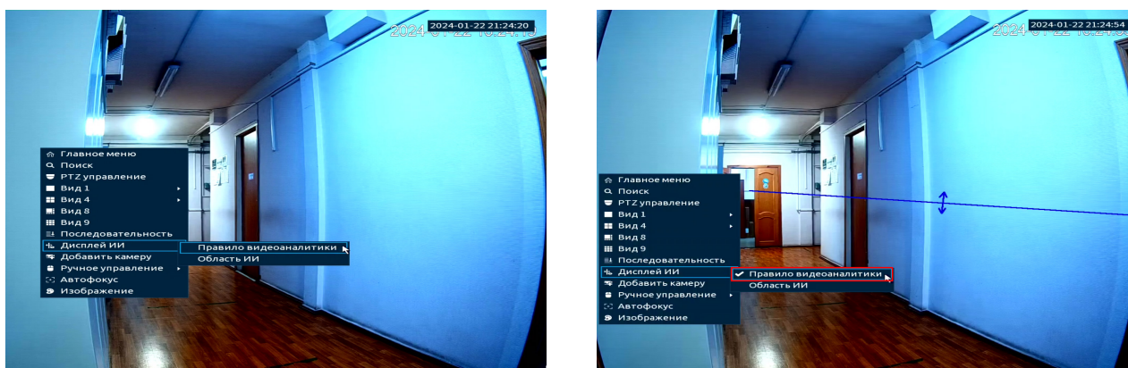
Рисунок 7.7 – Отображение видеонаналитики
