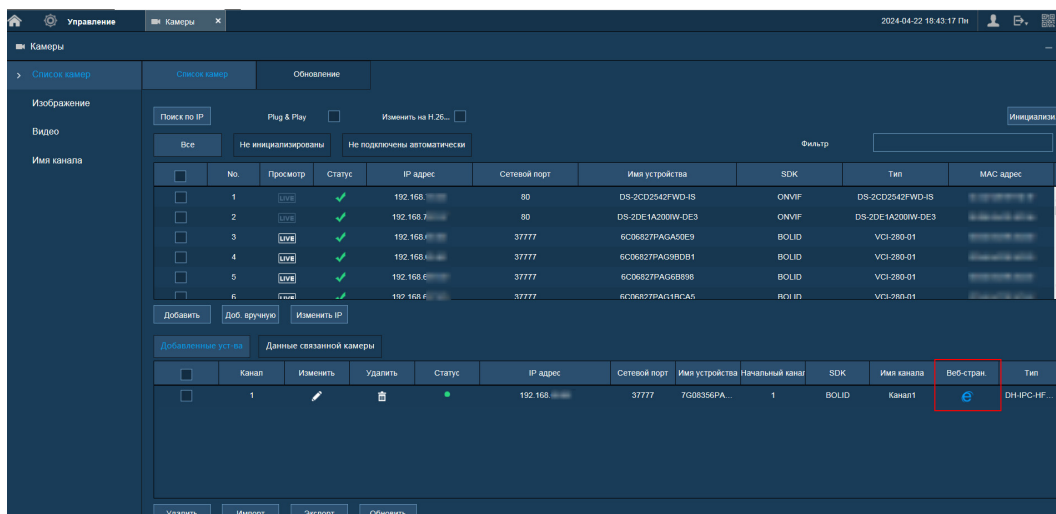
Рисунок 24.5 – Список камер
