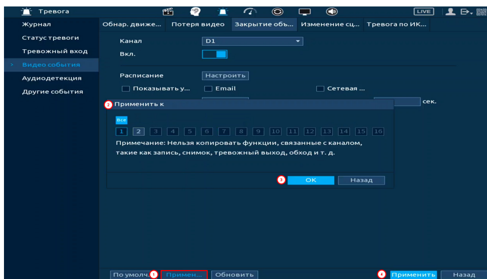
Рисунок 18.21 – Копирование настроек на другие каналы
