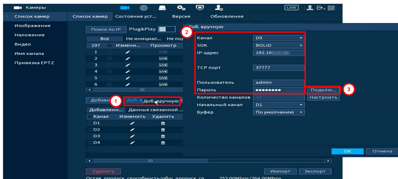
Рисунок 11.18 – Добавление видеопотока с другого регистратора
