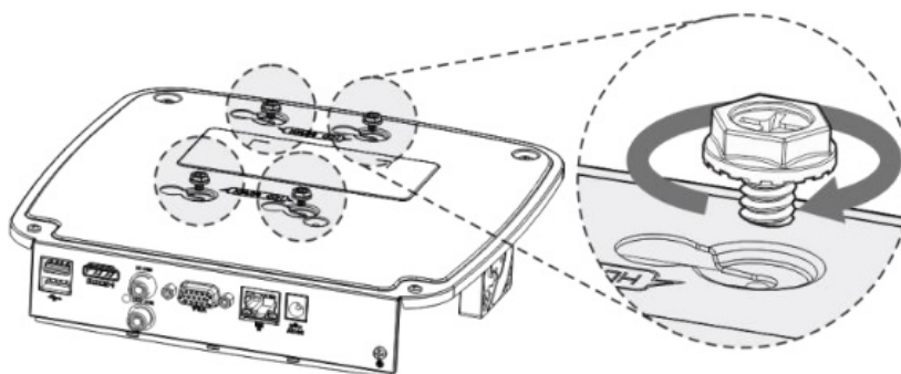
Рисунок 4.5 – Установка жёсткого диска
