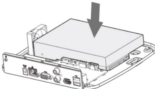
Рисунок 4.4 – Установка жёсткого диска
