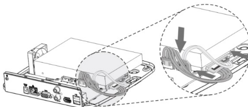
Рисунок 4.6 – Установка жёсткого диска
