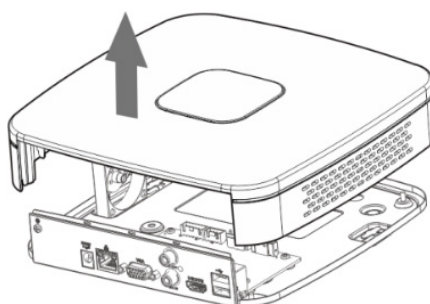
Рисунок 4.3 – Установка жёсткого диска
