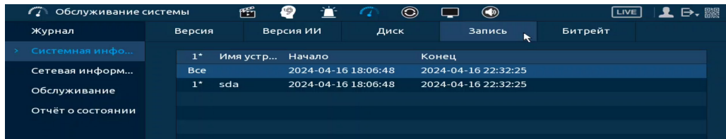
Рисунок 20.5 – Интерфейс просмотра
