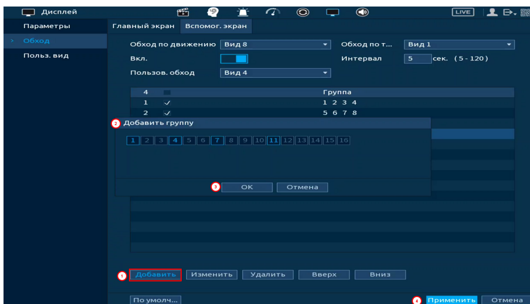
Рисунок 9.13 – Добавление группы
