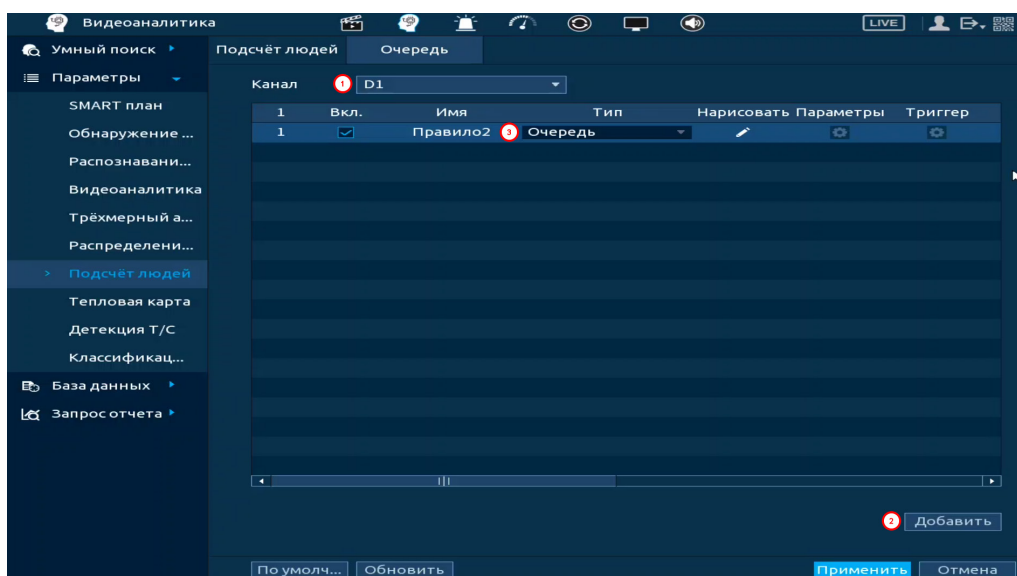
Рисунок 19.90 – Настройка
