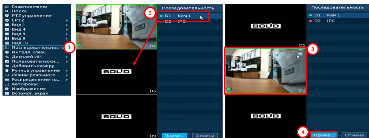
Рисунок 7.6 – Изменение раскладки
