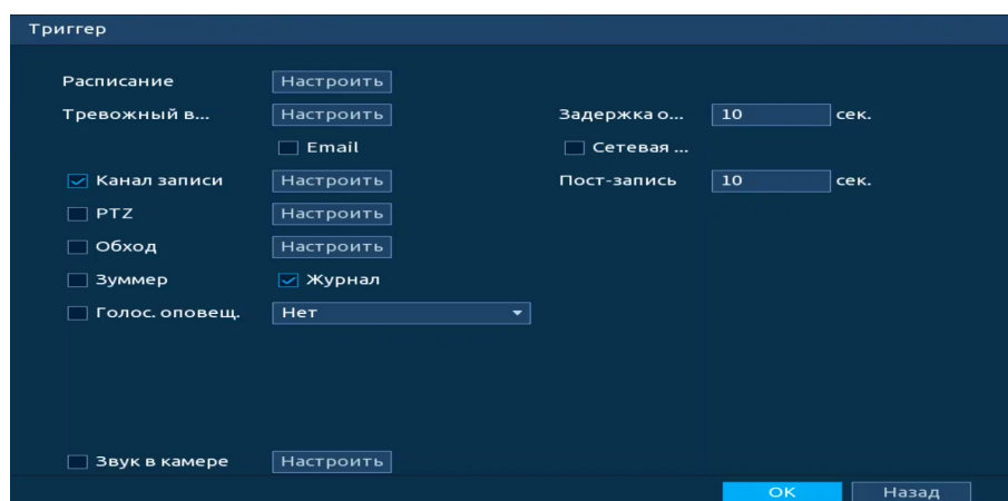
Рисунок 19.69 – Настройка параметров
