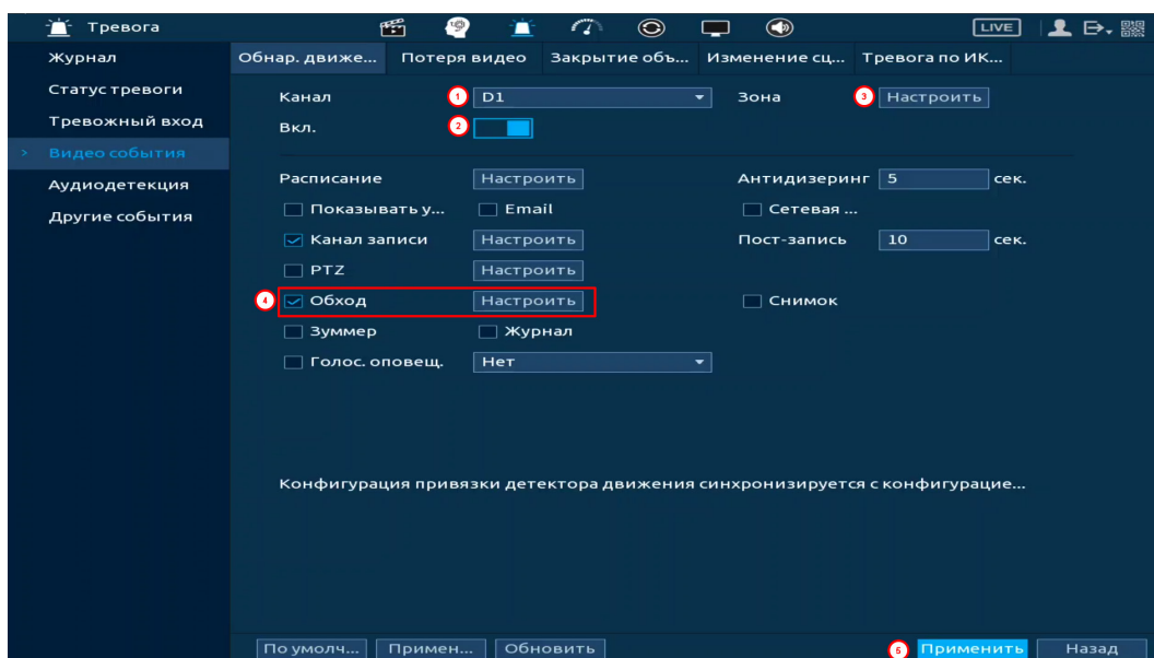
Рисунок 9.8 – Пример настройки
