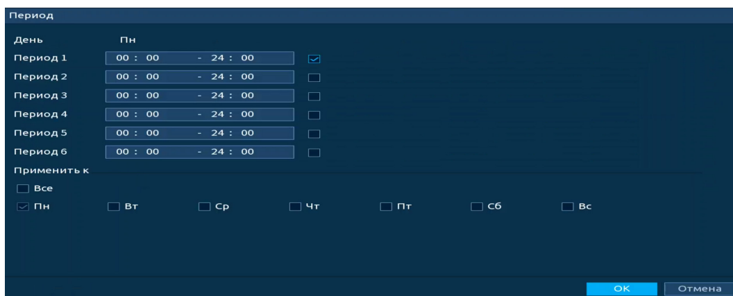
Рисунок 18.16 – Расписание
