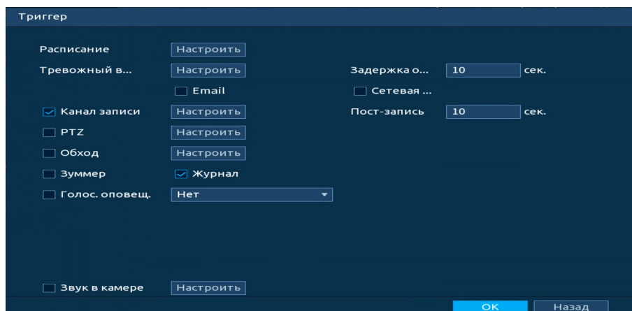
Рисунок 19.59 – Настройка параметров
