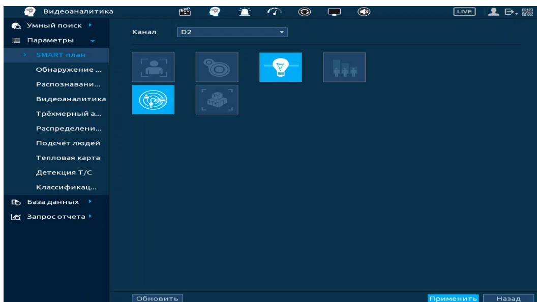
Рисунок 19.8 – Выбор функции
