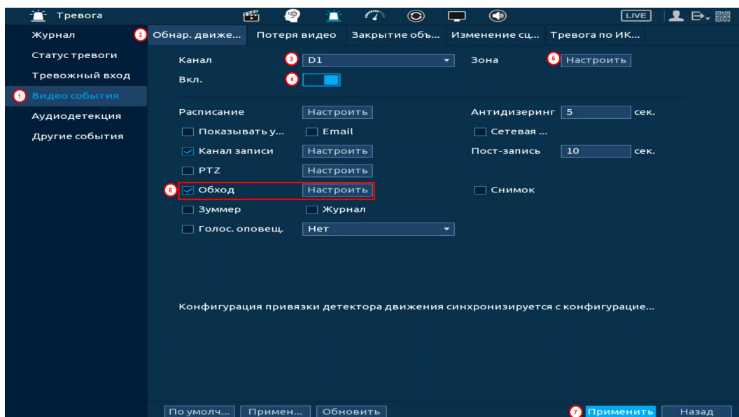
Рисунок 22.5 – Пример настройки
