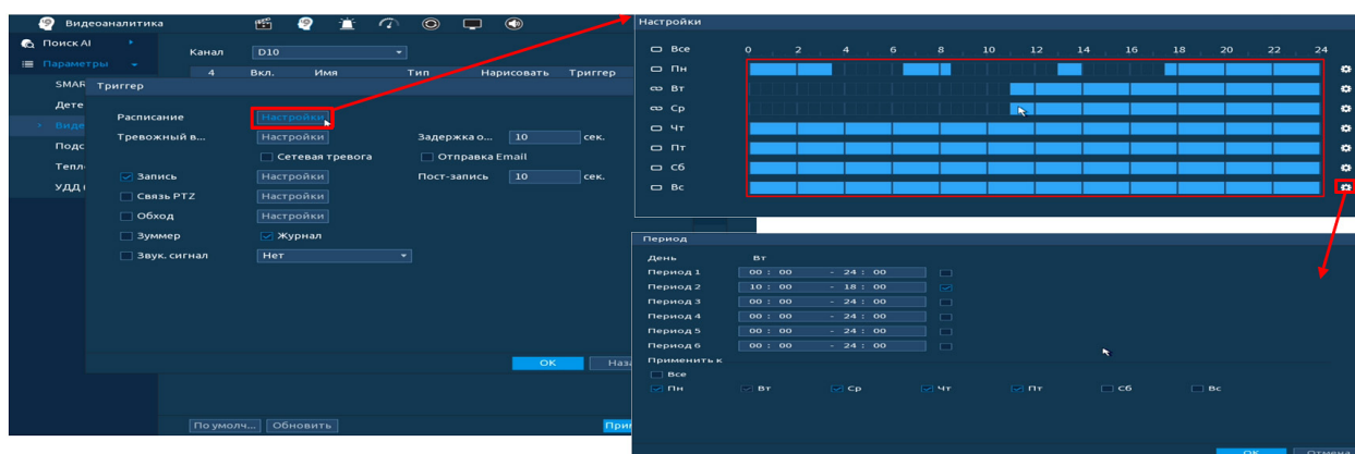
Рисунок 19.50 – Расписание
