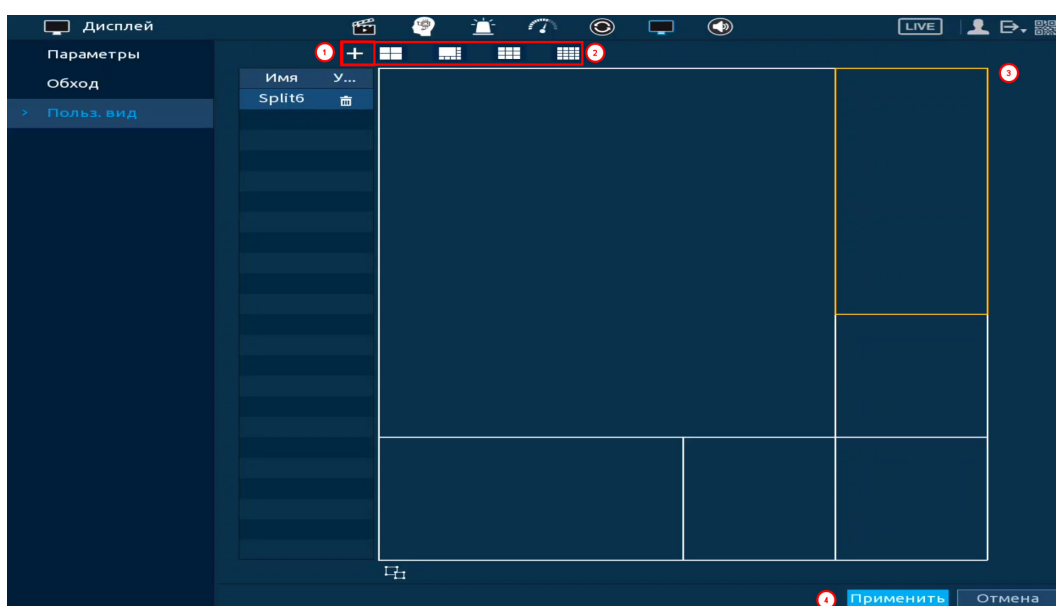
Рисунок 22.13 – Создание раскладки
