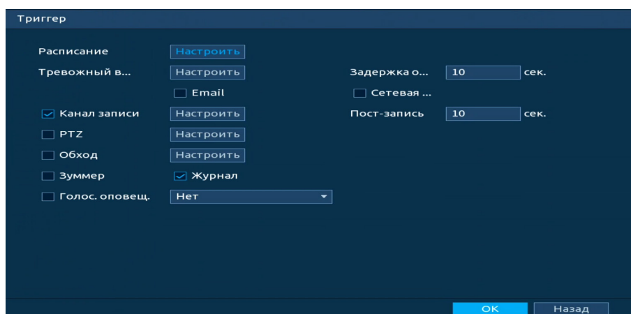
Рисунок 19.94 – Настройка параметров
