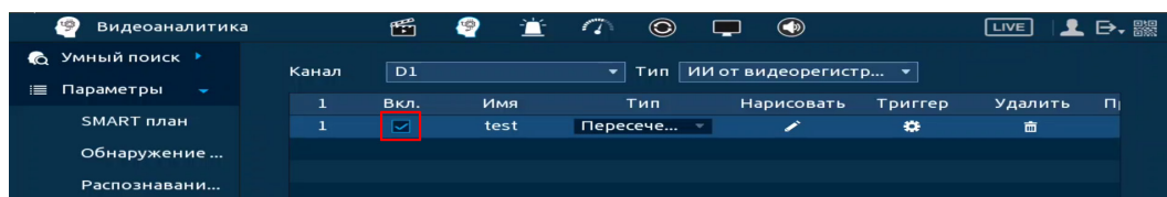
Рисунок 19.29 – Настройка
