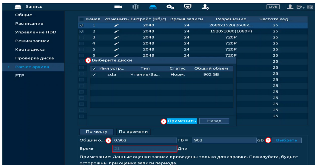
Рисунок 13.21 – Настройка
