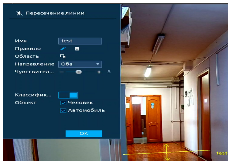
Рисунок 19.28 – Настройка правила
