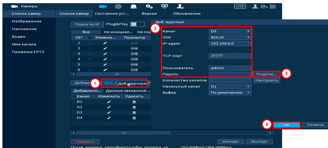
Рисунок 11.16 – Интерфейс ручного добавления удалённого устройства
