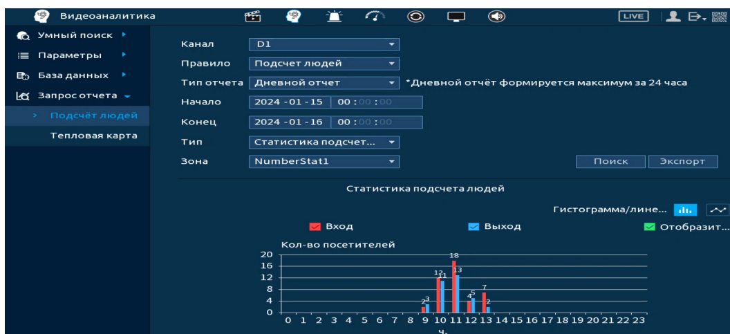
Рисунок 19.107 – Интерфейс просмотра подсчета людей
