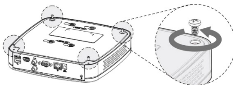
Рисунок 4.2 – Установка жёсткого диска
