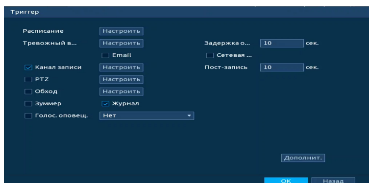
Рисунок 19.30 – Настройка
