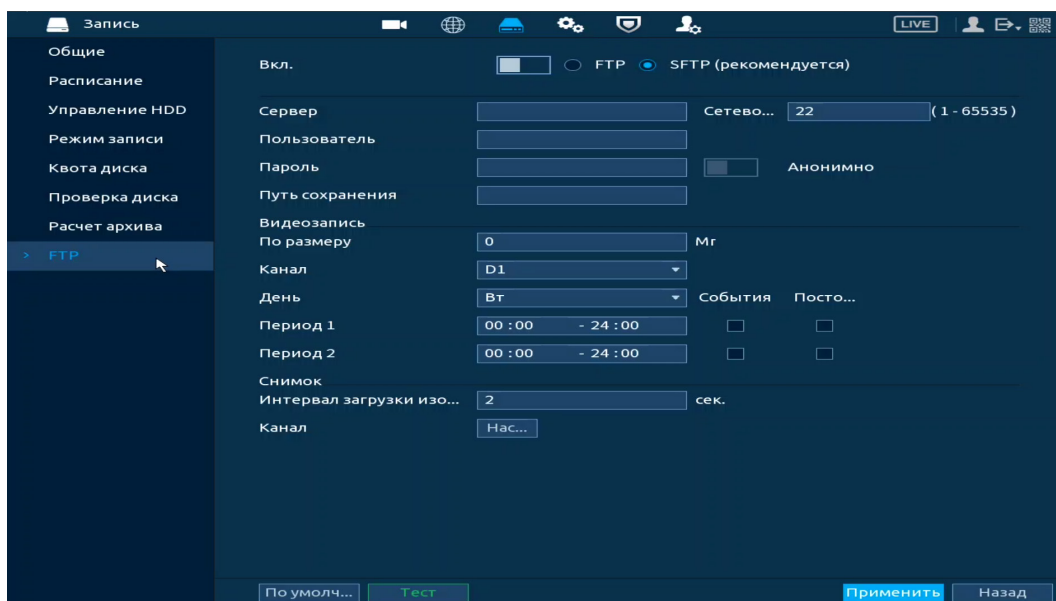
Рисунок 13.24 – Настройка FTP
