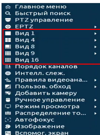
Рисунок 7.1 – Контекстное меню
