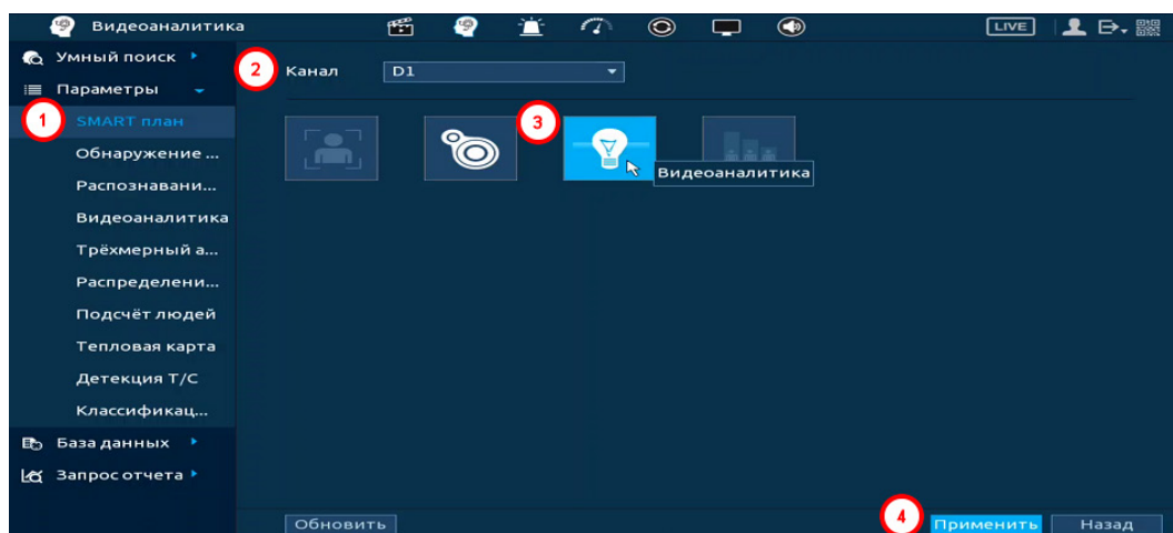
Рисунок 19.61 – Настройка
