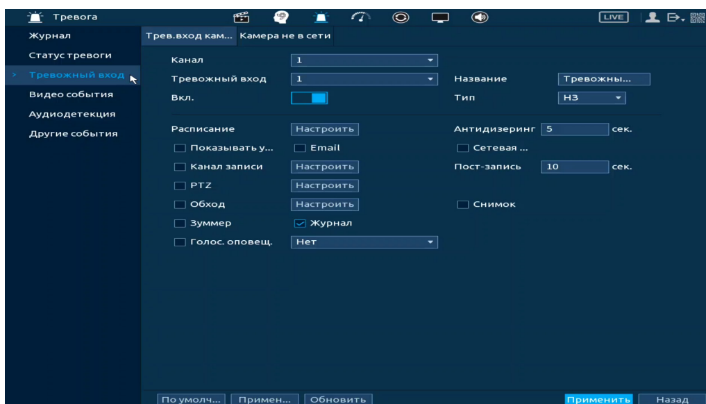
Рисунок 18.3 – Интерфейс настройки
