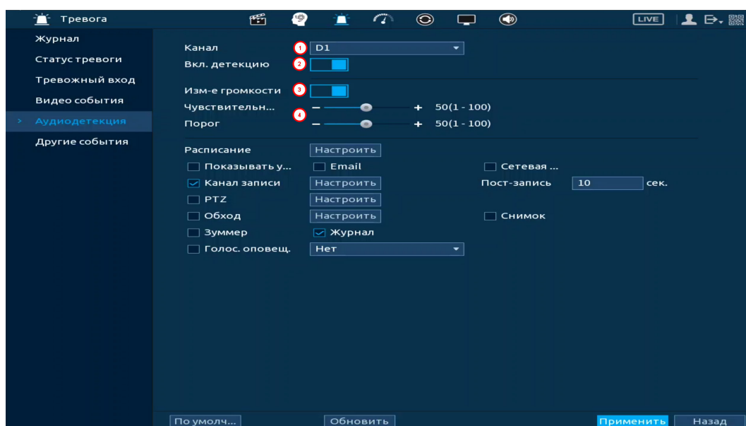
Рисунок 18.28 – Настройка аудиодетекции
