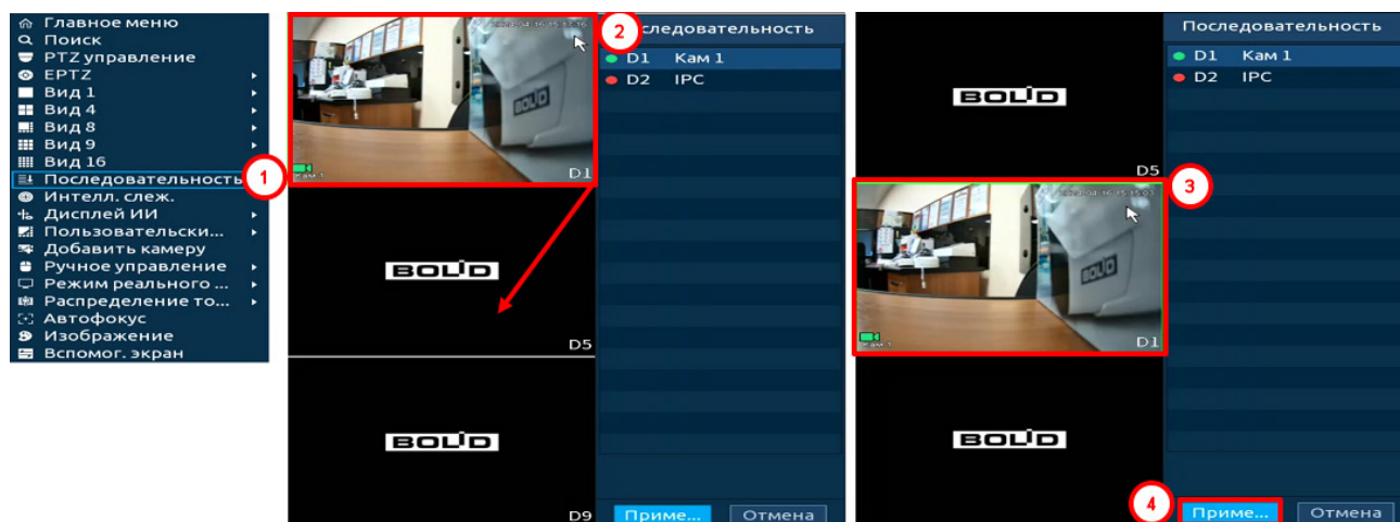
Рисунок 7.7 – Изменение раскладки
