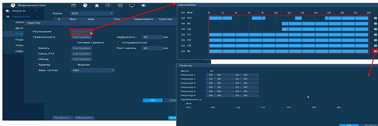
Рисунок 19.65 – Расписание
