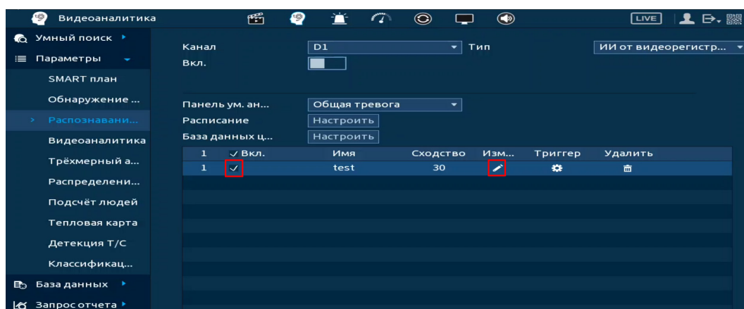
Рисунок 19.18 – Настройка
