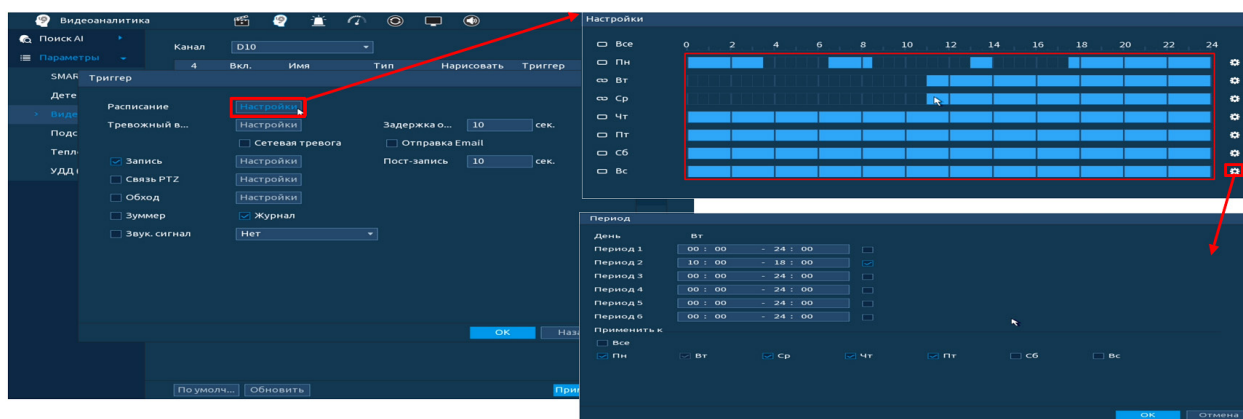
Рисунок 19.88 – Расписание
