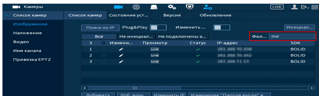
Рисунок 11.8 – Фильтр
