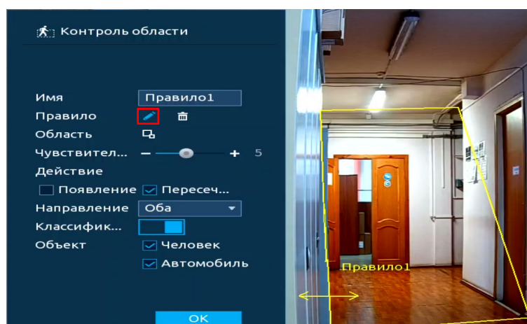
Рисунок 19.35 – Настройка
