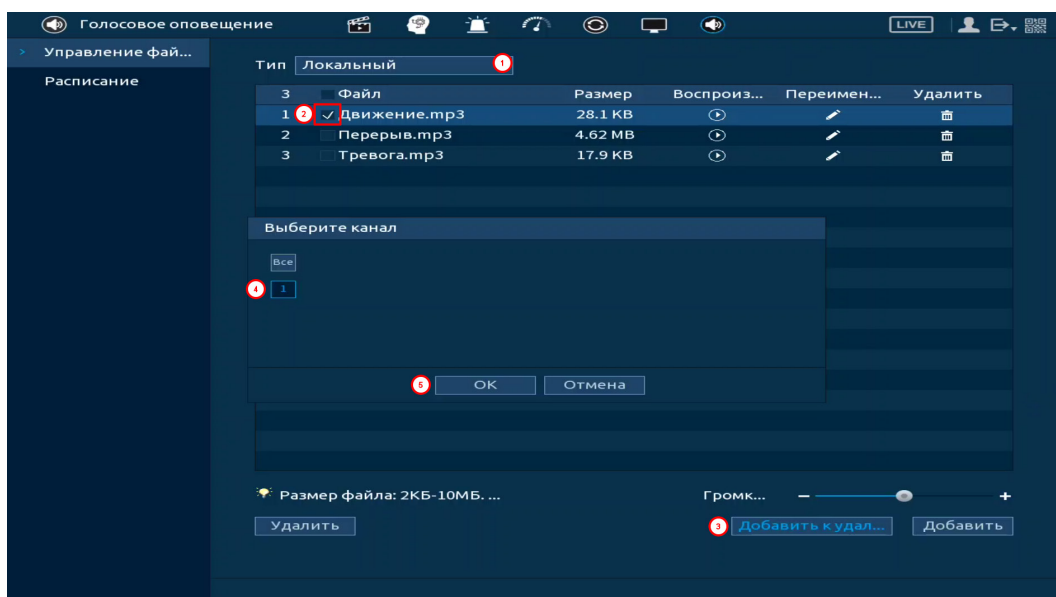
Рисунок 23.5 – Добавление
