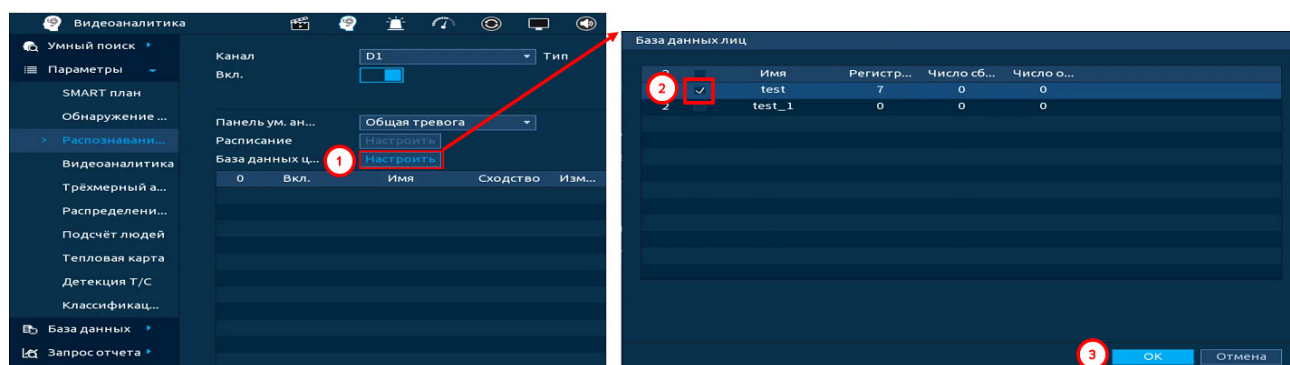
Рисунок 19.17 – Настройка
