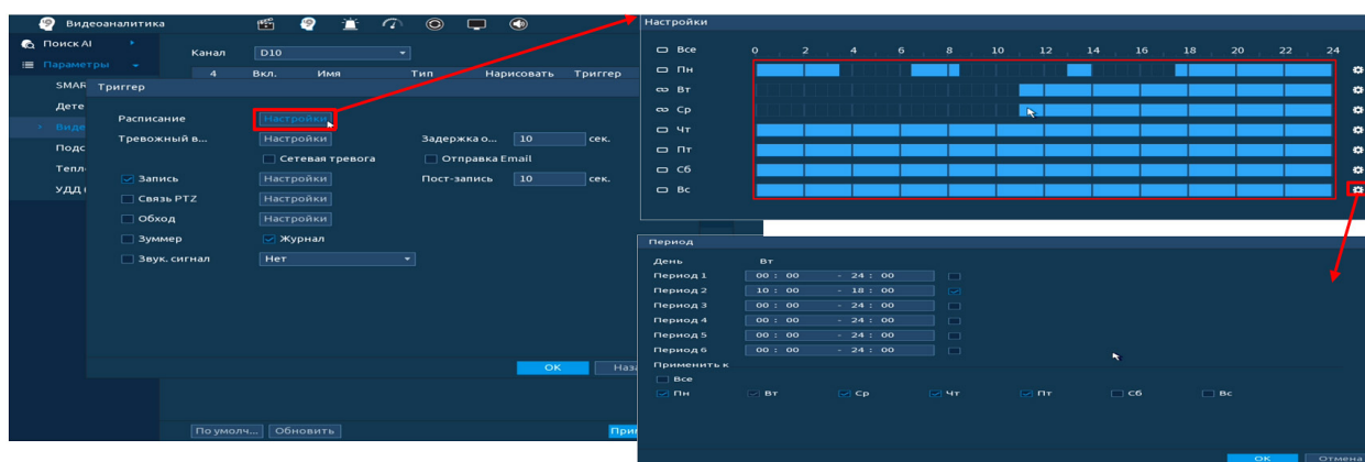
Рисунок 19.95 – Расписание
