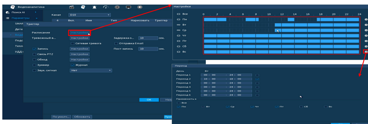
Рисунок 19.70 – Расписание
