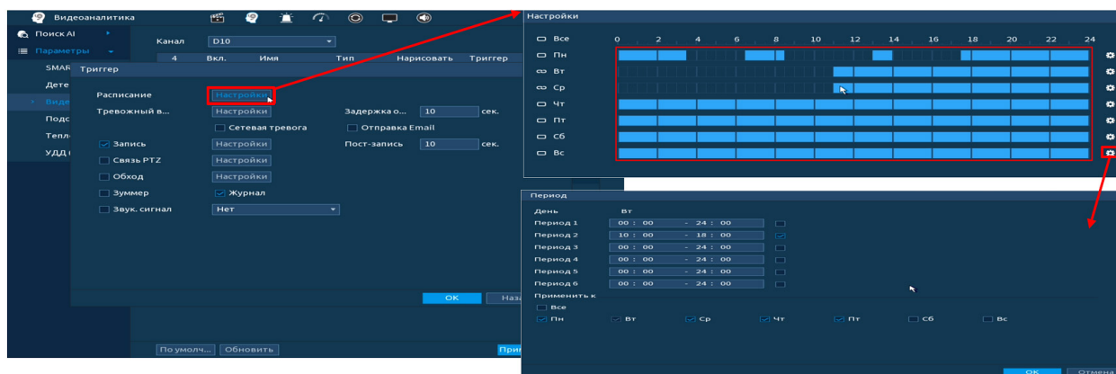
Рисунок 19.60 – Расписание
