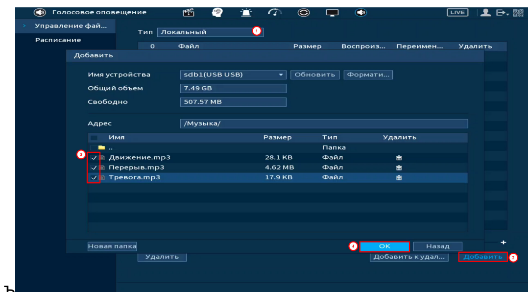
Рисунок 23.2 – Добавление
