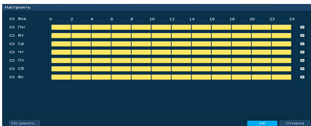
Рисунок 18.26 – Панель расписания
