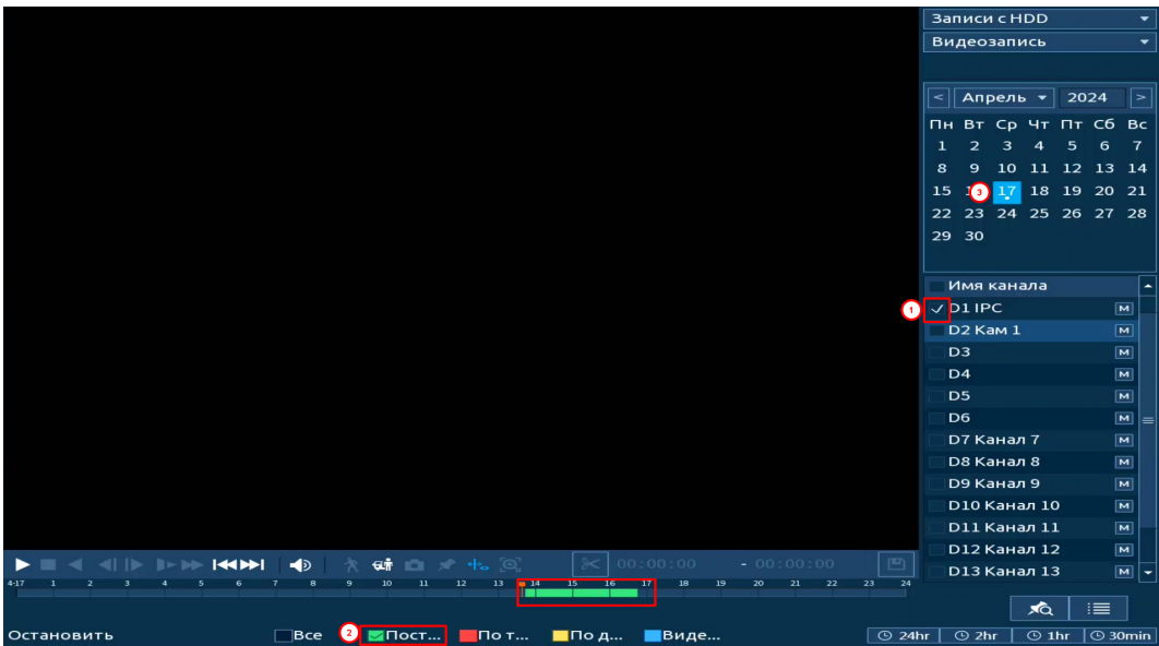
Рисунок 17.5 – Шкала времени
