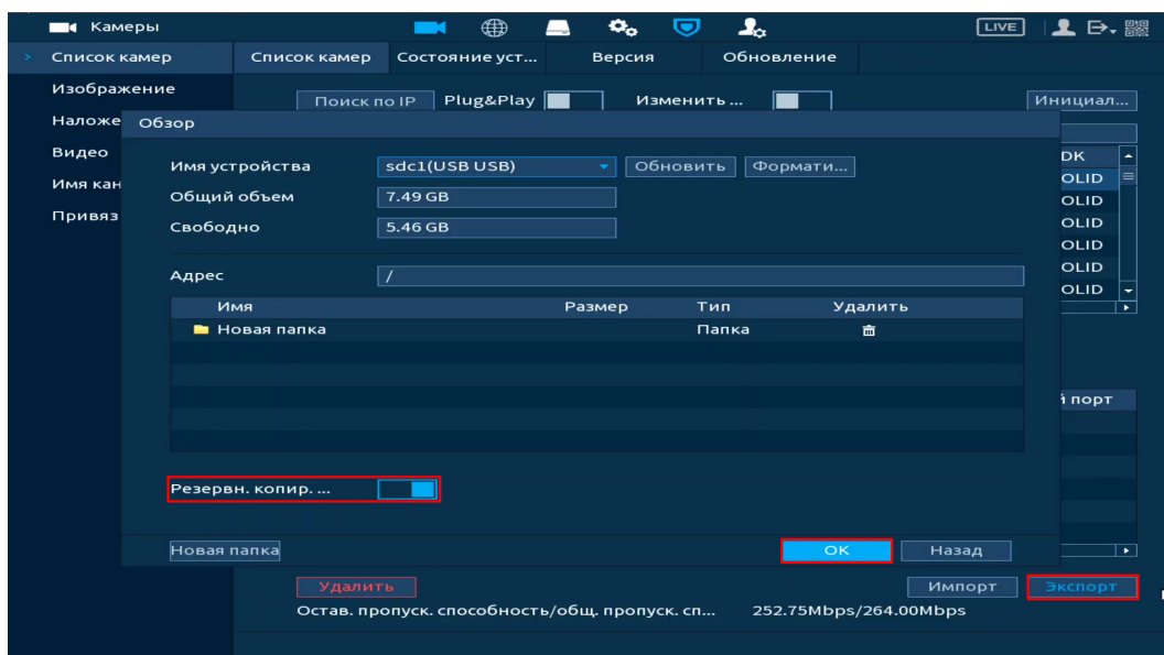
Рисунок 11.22 – Экспорт
