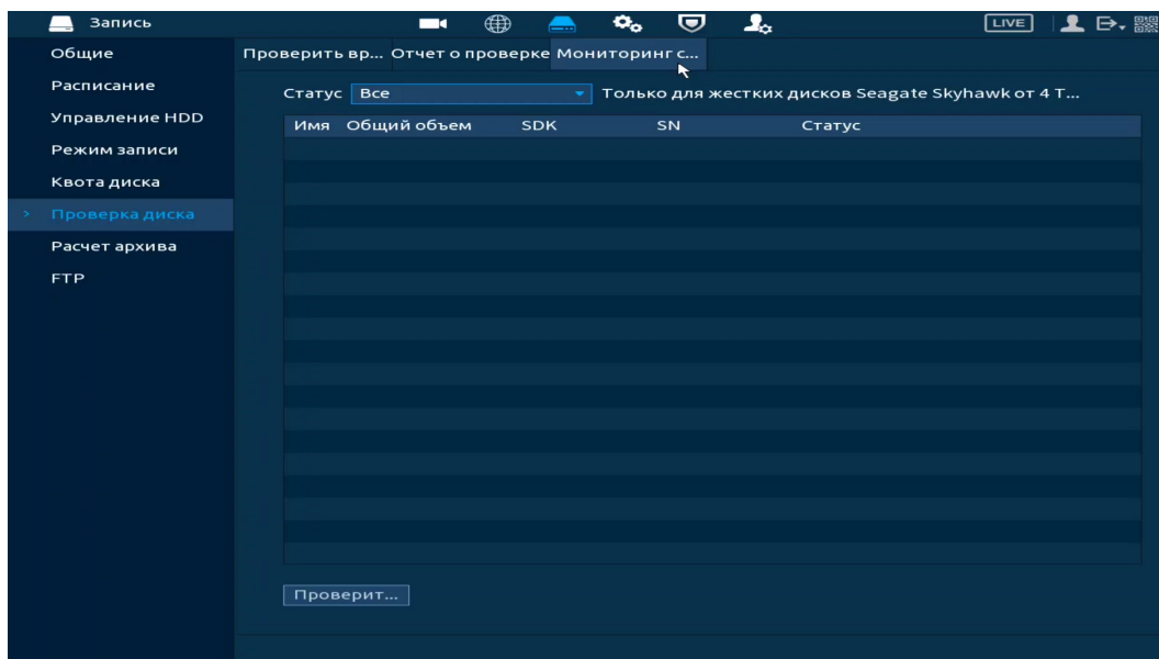
Рисунок 13.19 – Мониторинг состояния
