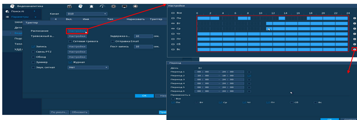
Рисунок 19.98 – Расписание
