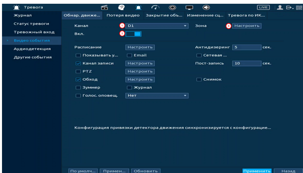
Рисунок 18.9 – Настройка события
