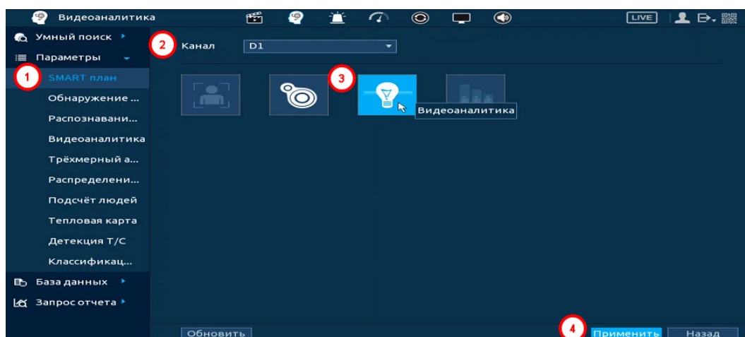
Рисунок 19.46 – Настройка
