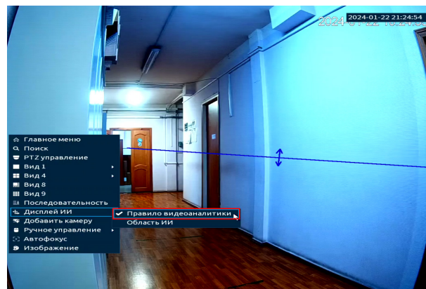
Рисунок 7.9 – Отображение видеоаналитики
