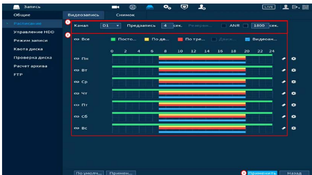
Рисунок 14.7 – Настройка расписания записи
