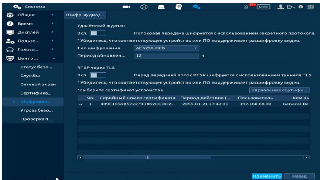
Рисунок 18.55 – Интерфейс шифрования аудио/видео
