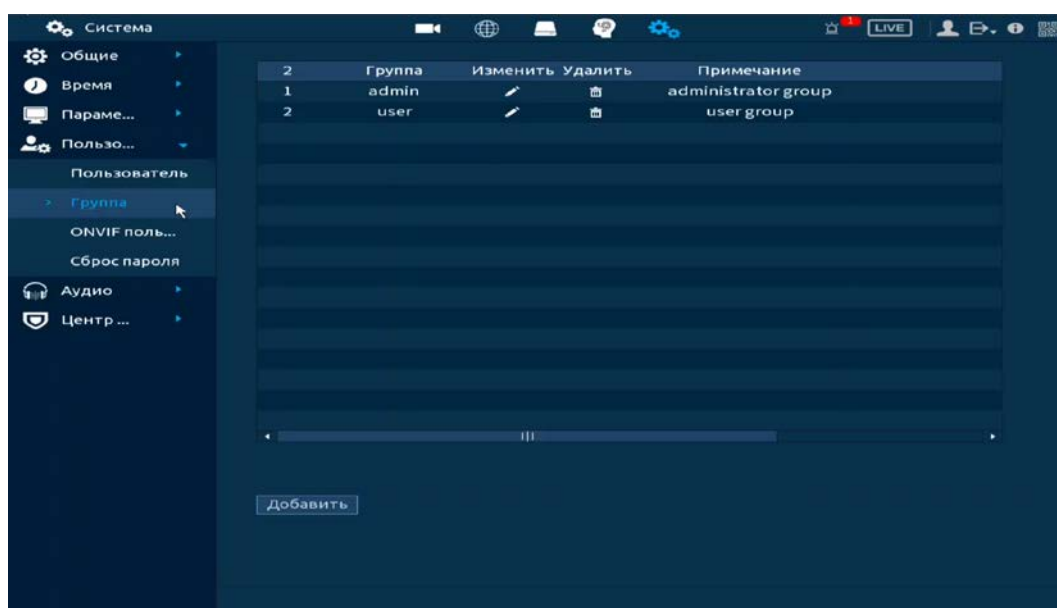
Рисунок 18.22 – Интерфейс добавления группы учётной записи
