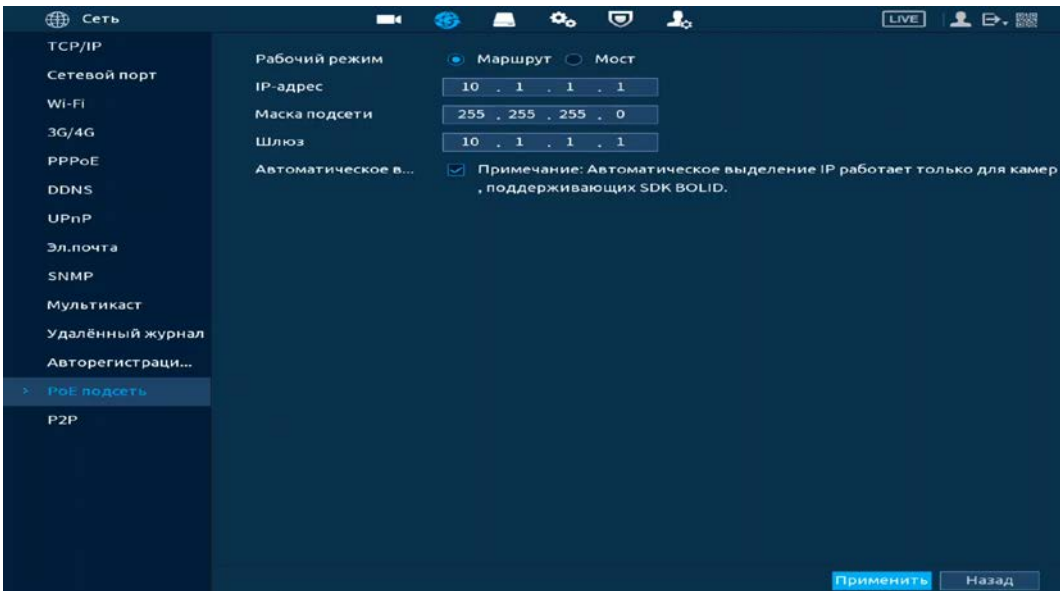
Рисунок 13.16 – Интерфейс настройки «PoE подсеть»
