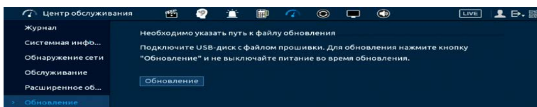
Рисунок 19.9 – Выбор файла для обновления
