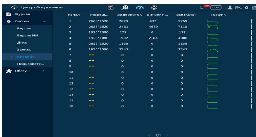
Рисунок 19.6 – Интерфейс просмотра битрейта
