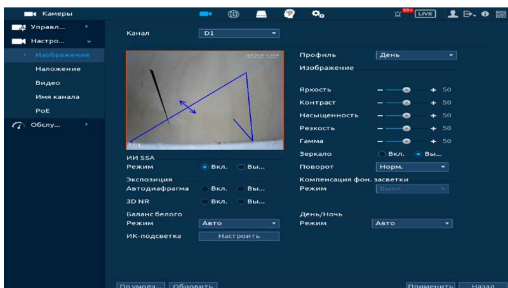
Рисунок 12.29 – Интерфейс настройки изображения
