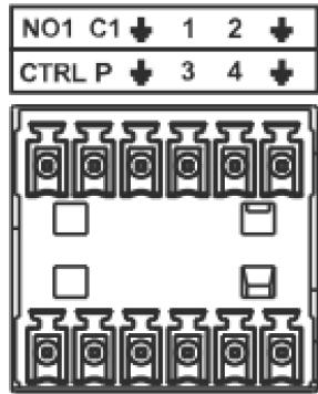
Рисунок 3.3 – Тревожный вход/выход
