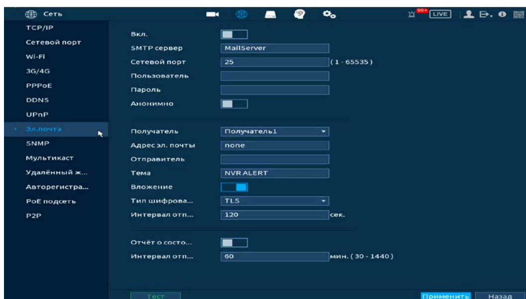
Рисунок 13.10 – Интерфейс настройки «Электронная почта»
