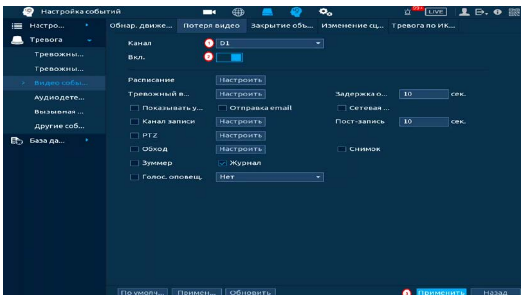
Рисунок 15.24 – Интерфейс настройки потери видео
