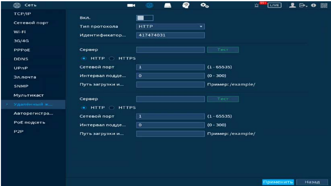
Рисунок 13.13 – Интерфейс настройки «HTTP»
