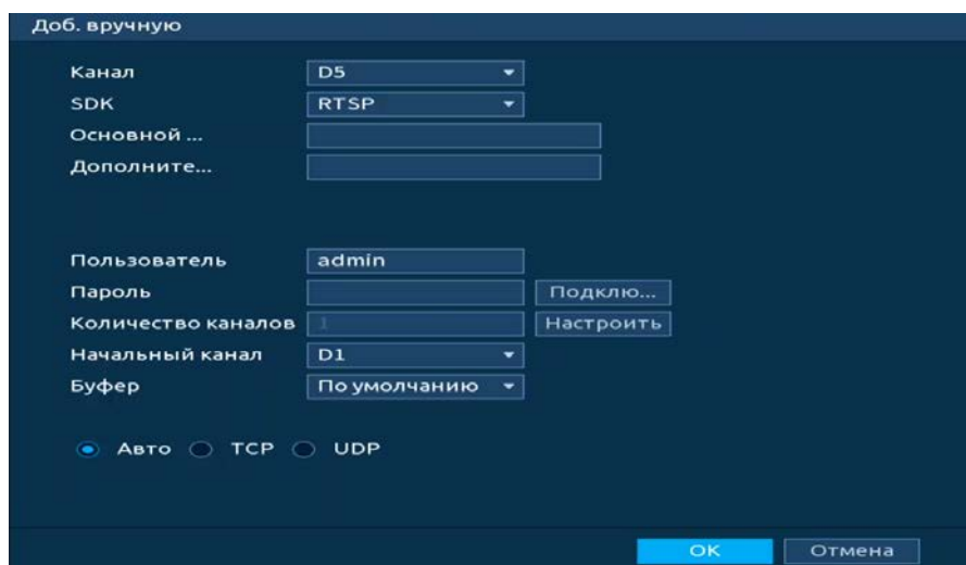
Рисунок 12.19 – Работа со сторонними клиентами по протоколу RTSP
