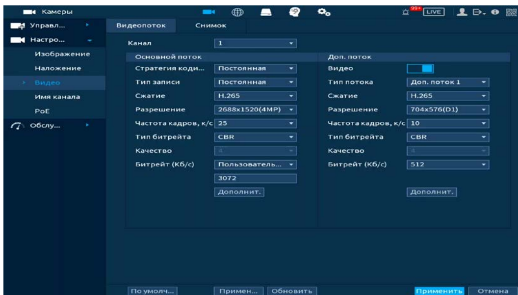
Рисунок 12.36 – Интерфейс настройки видеопотоков
