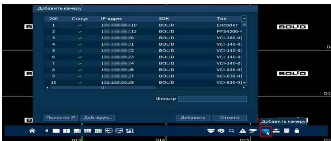
Рисунок 12.3 – Добавление через панель навигации
