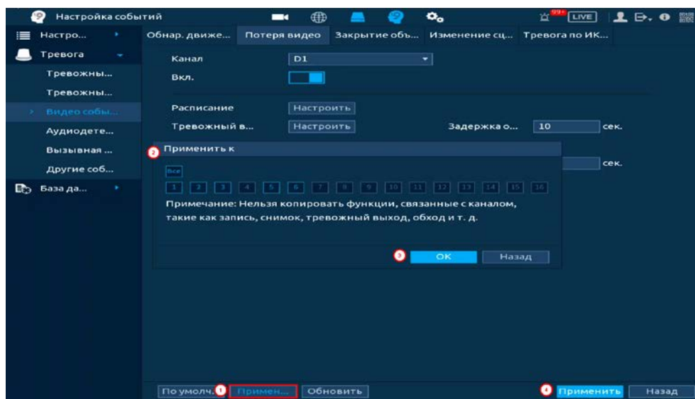
Рисунок 15.27 – Копирование настроек на другие каналы
