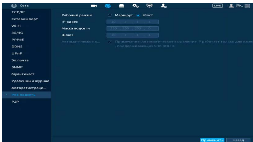
Рисунок 13.17 – Интерфейс настройки «PoE подсеть»
