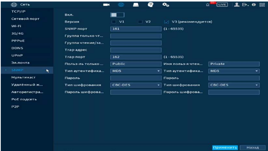
Рисунок 13.11 – Интерфейс настройки «SNMP»
