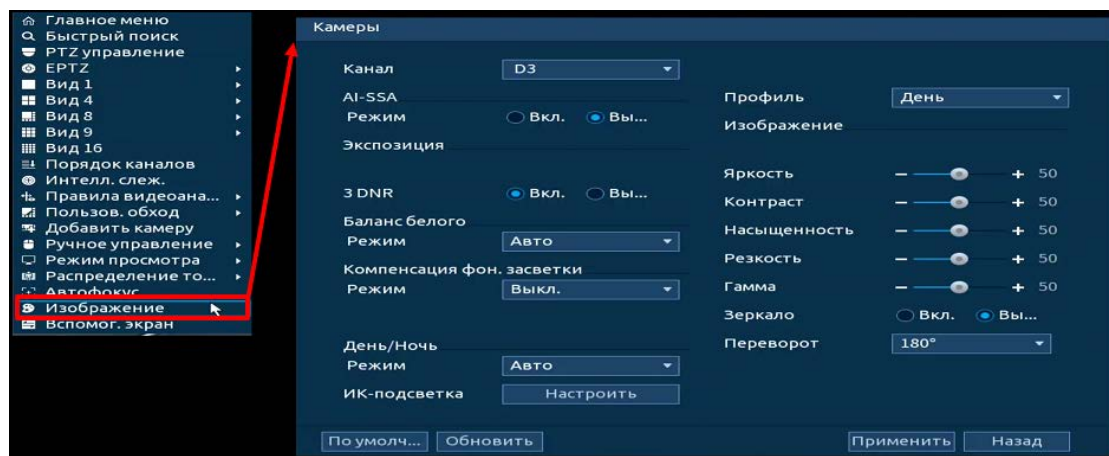
Рисунок 12.31 – Переход в меню редактирования изображения через контекстное меню
