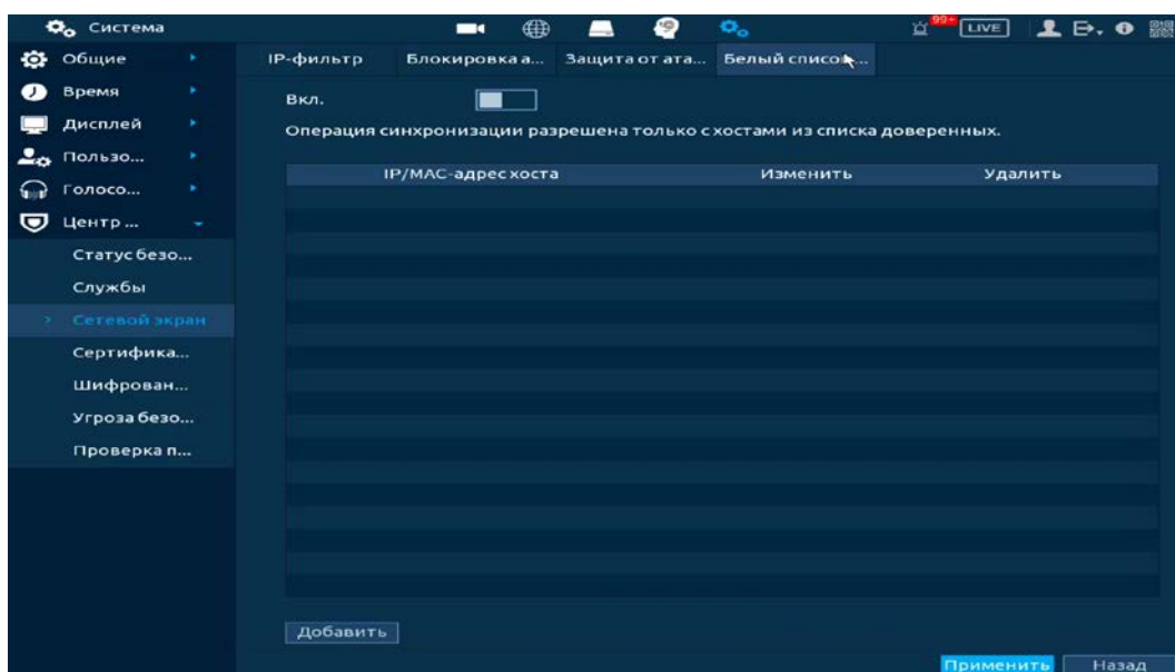
Рисунок 18.49 – Белый список NTP-серверов
