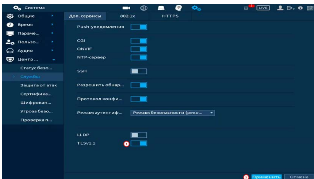
Рисунок 18.41 – Настройка. Доп. сервисы
