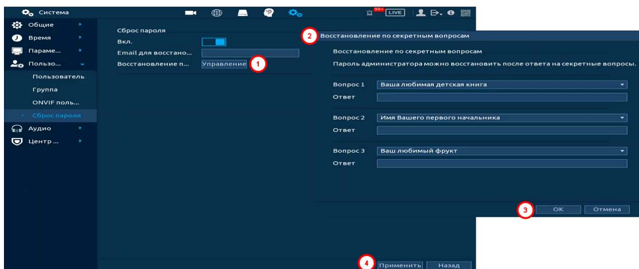
Рисунок 18.28 – Восстановление по секретным вопросам
