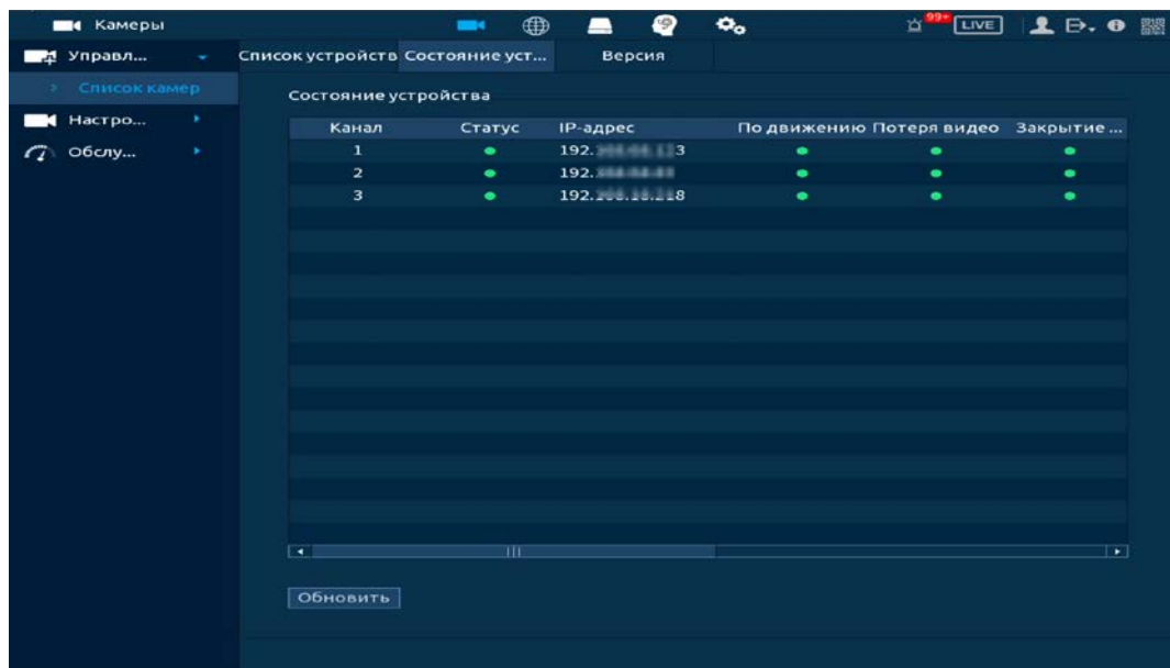
Рисунок 12.27 – Интерфейс просмотра состояния подключенных устройств
