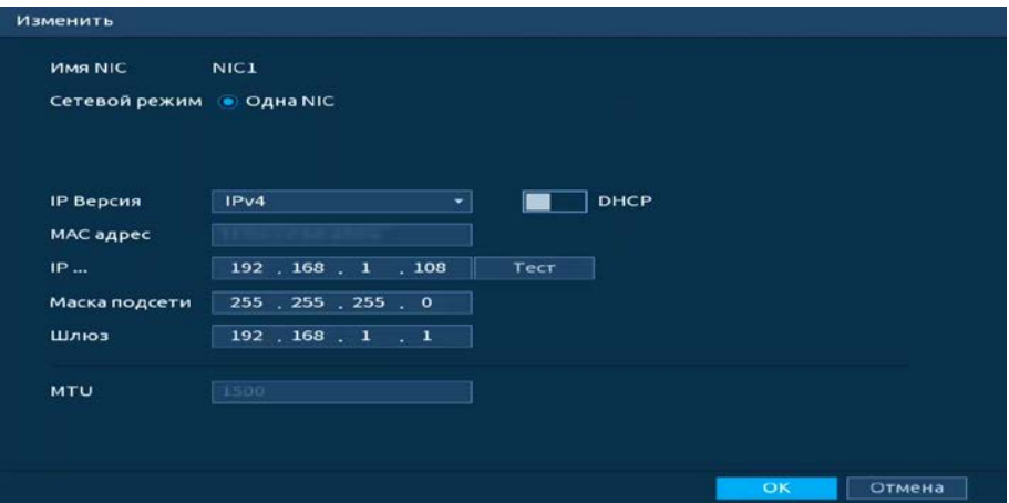
Рисунок 6.8 – Интерфейс меню быстрой настройки «Сеть»
