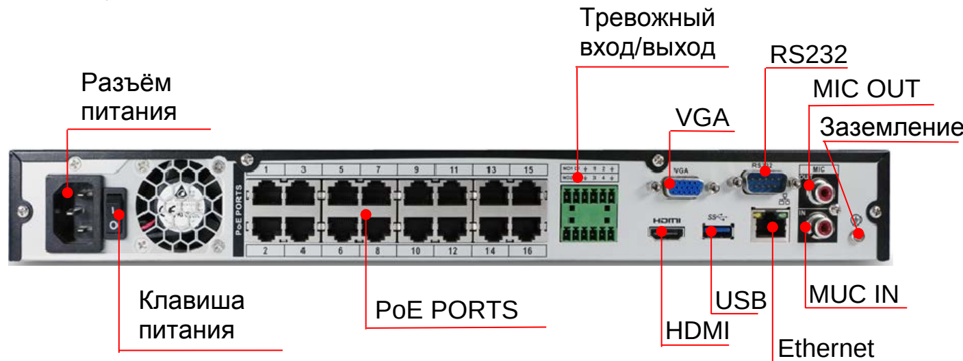
Рисунок 3.2 – Внешний вид задней панели
