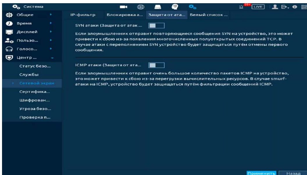
Рисунок 18.48 – Включение защиты от DoS атак
