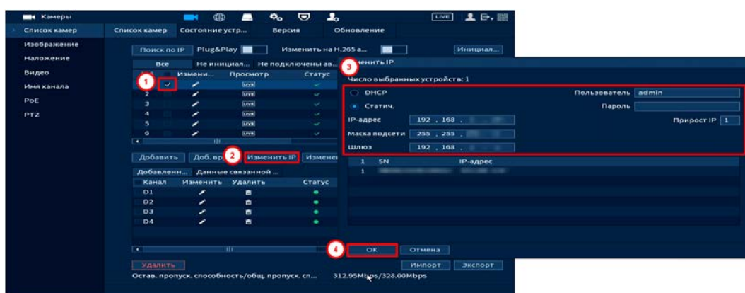
Рисунок 11.21 – Изменения сетевых настроек IP-камер через видеорегистратор
