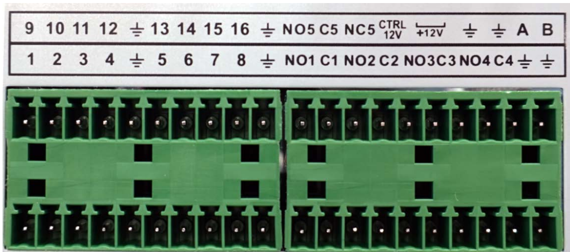
Рисунок 3.3 – Тревожный вход/выход, RS-485
