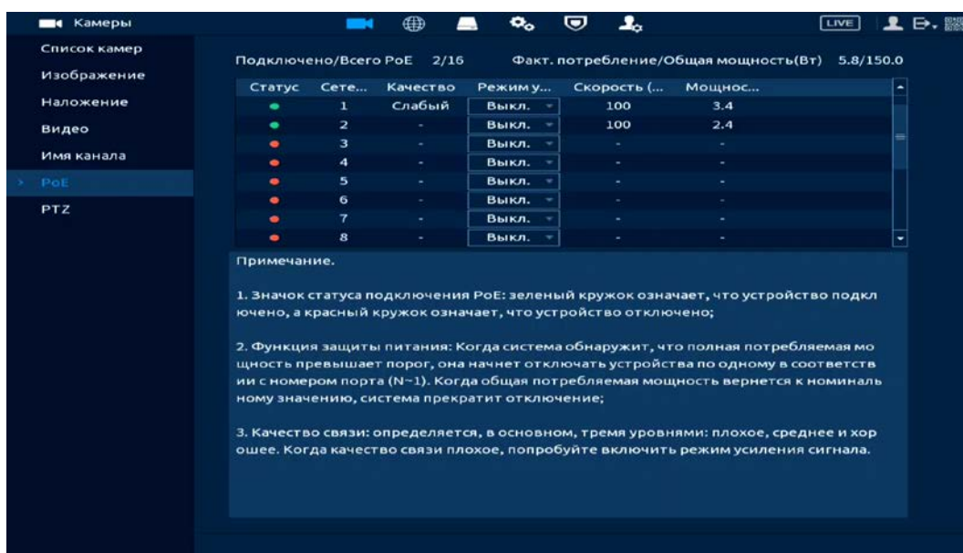
Рисунок 11.26 – Интерфейс просмотра подключенных устройств (PoE)
