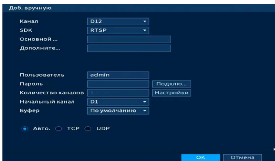
Рисунок 11.17 – Подключение к стороннему RTSP потоку
