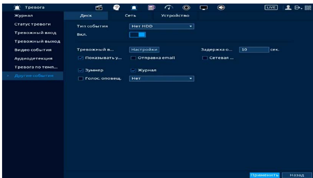
Рисунок 18.44 – Интерфейс настройки оповещения об ошибках HDD
