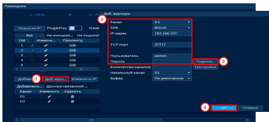
Рисунок 6.12 – Ручной режим добавления
