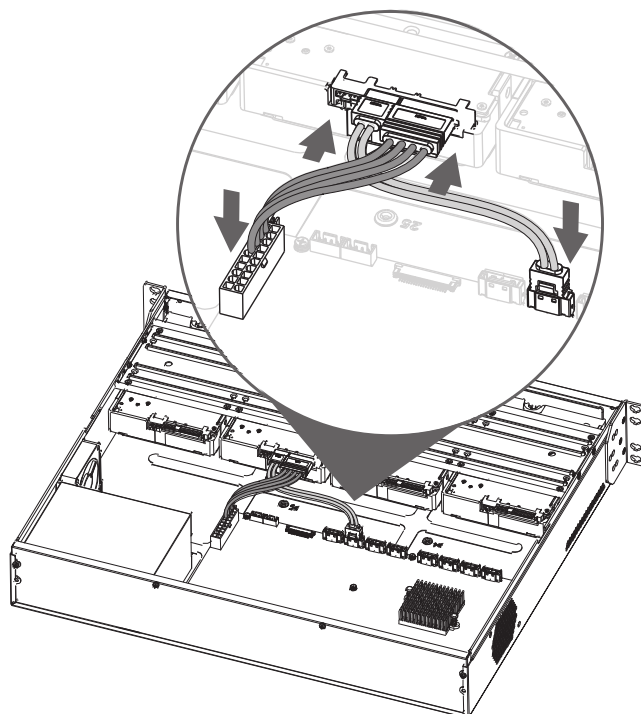
Рисунок 4.7 – Установка жёсткого диска
