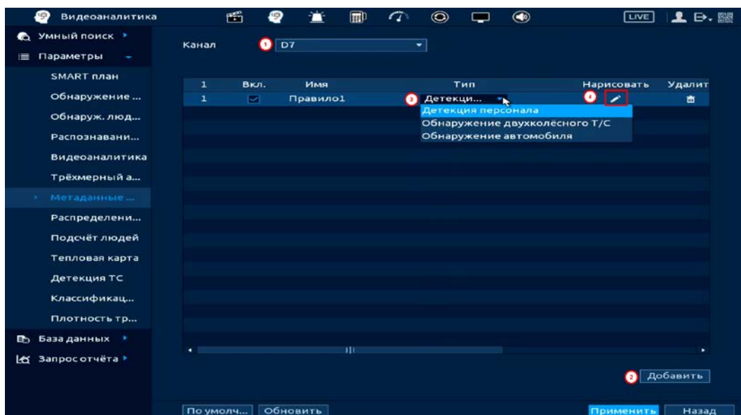
Рисунок 19.72 – Функция «Метаданные видео»
