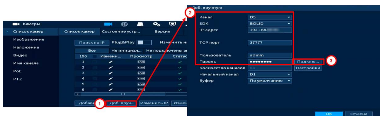
Рисунок 11.18 – Добавление видеопотока с другого регистратора
