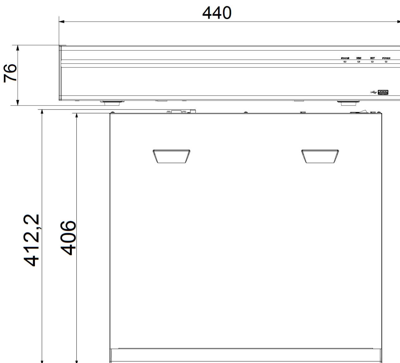
Рисунок 4.1 – Габаритные размеры видеорегистратора
