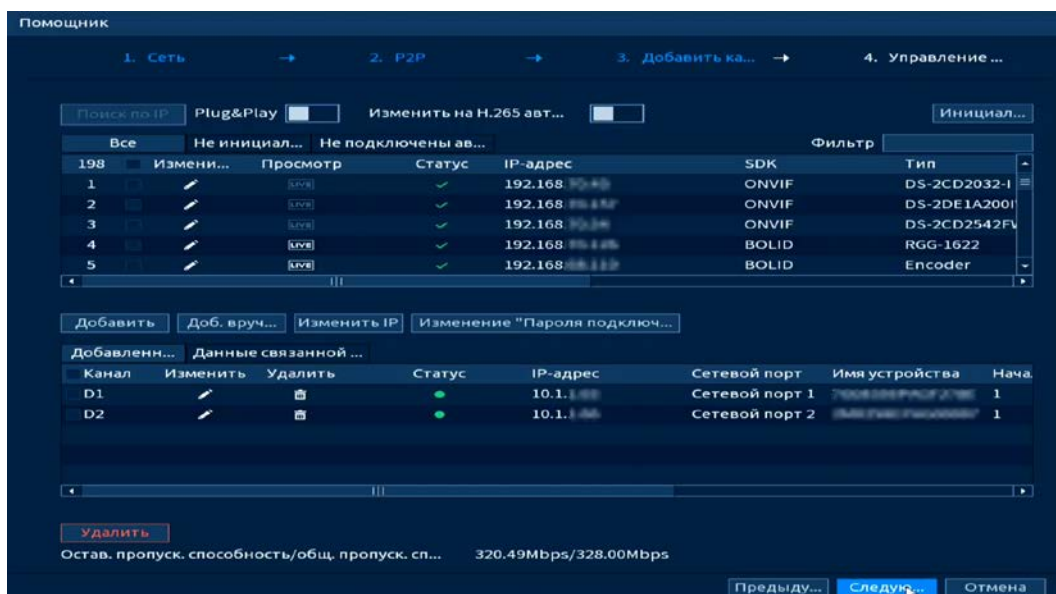
Рисунок 6.10 – Интерфейс меню быстрой настройки «Добавление камер»
