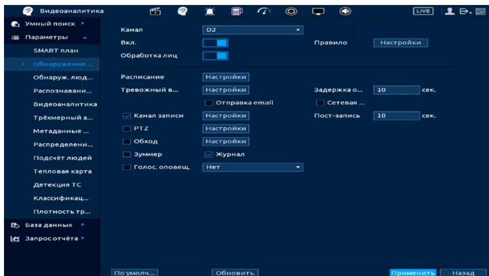
Рисунок 19.9 – Интерфейс настройки обнаружения лиц
