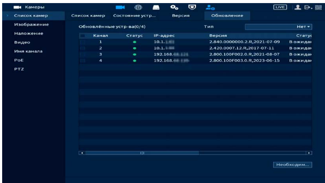
Рисунок 11.25 – Интерфейс обновления ПО камер
