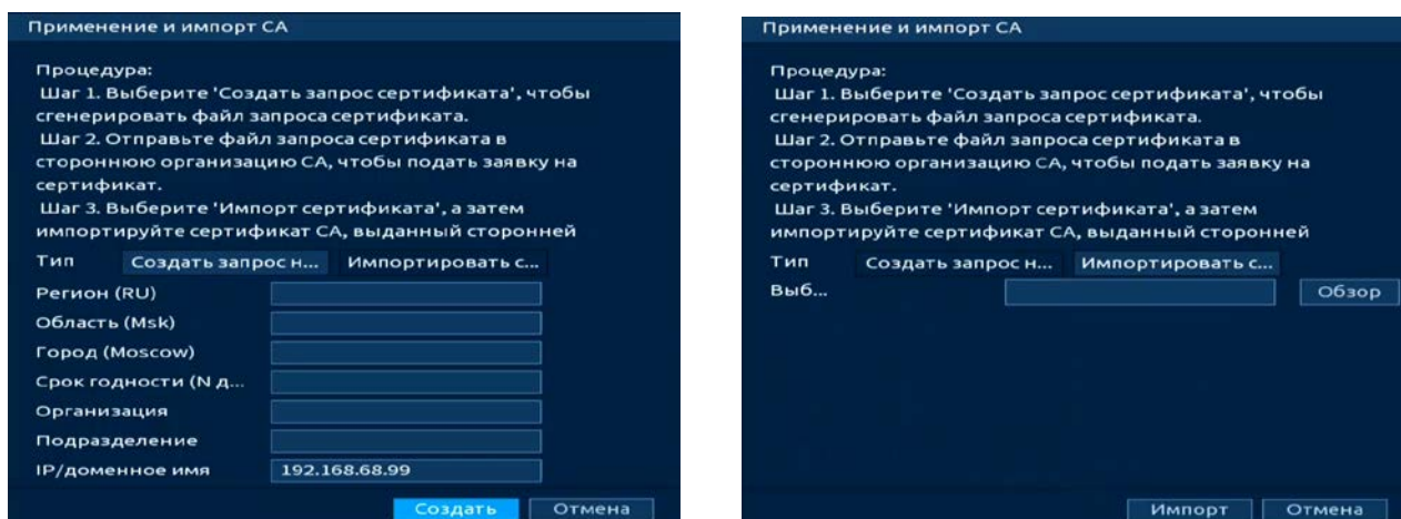
Рисунок 15.17 – Создание и импорт доверенного сертификата
