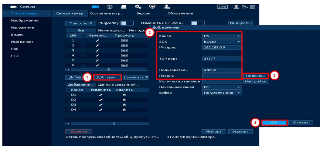
Рисунок 11.16 – Интерфейс ручного добавления удалённого устройства
