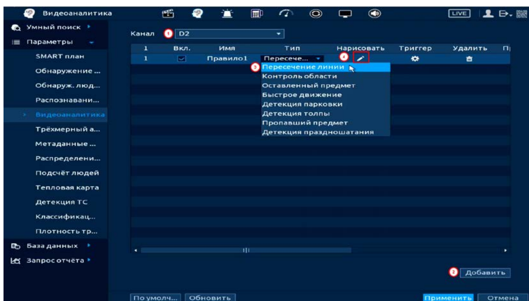
Рисунок 19.21 – Функция видеоаналитики «Пересечение линии»
