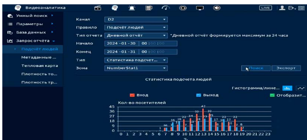
Рисунок 19.120 – Интерфейс просмотра подсчёта людей
