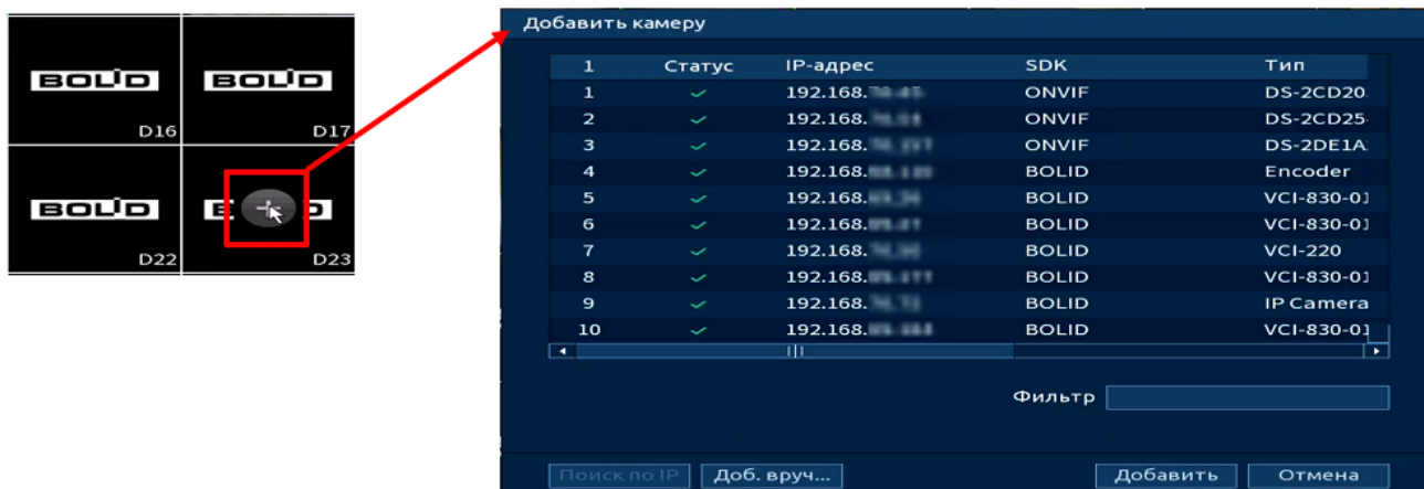
Рисунок 11.2 – Добавление в режиме просмотра
