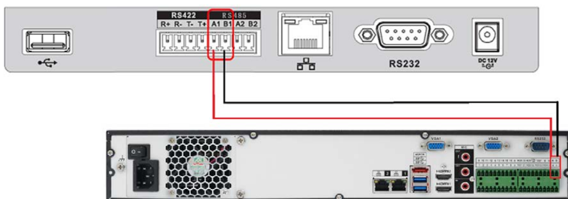
Рисунок 14.4 – Схема RS-485
