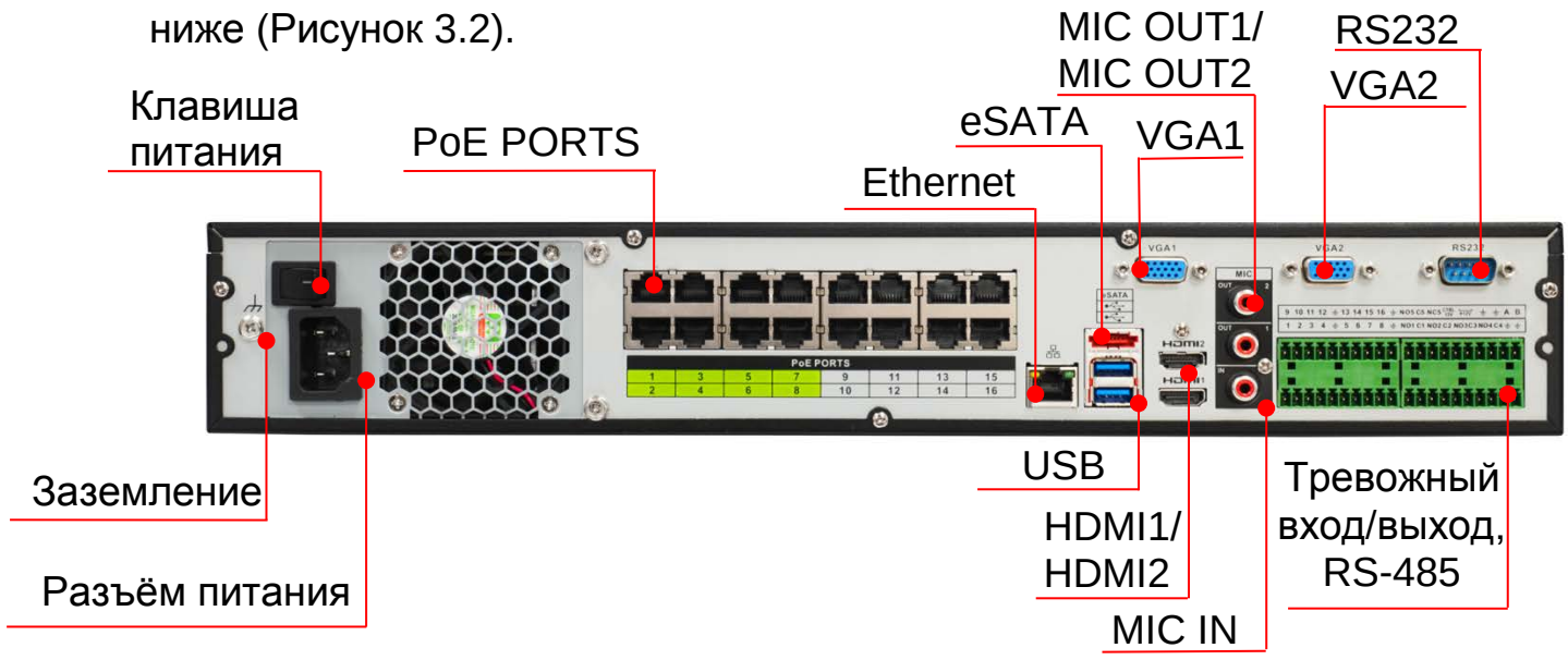
Рисунок 3.2 – Внешний вид задней панели
