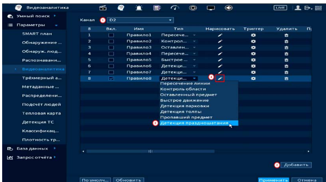
Рисунок 19.66 – Функция видеоаналитики «Детекция праздногошатания»
