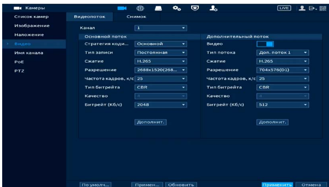
Рисунок 11.31 – Интерфейс настройки видеопотоков
