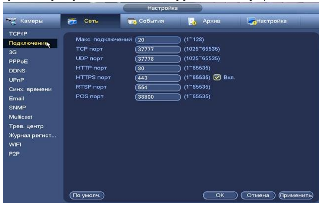
Рисунок 8.3.2.2.1 Интерфейс настройки «Подключение».
