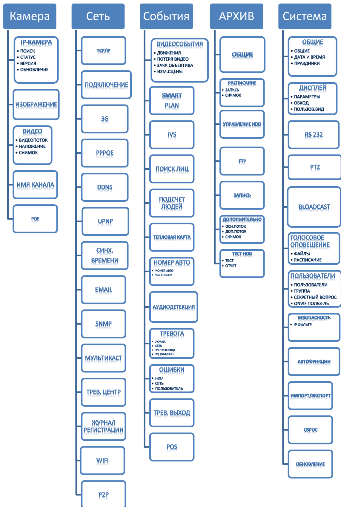
Рисунок 8.3.1 Схема меню «Настройка»
