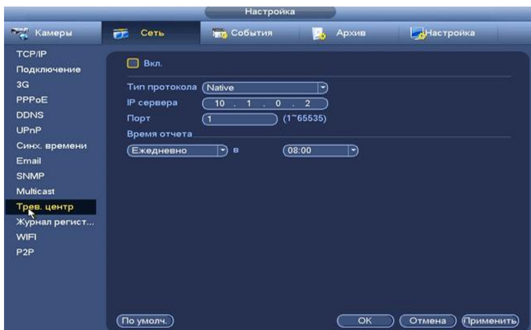
Рисунок 8.3.2.14.1 Интерфейс настройки «Трев. центр». Параметры и функции настройки описаны в таблице 8.16.
