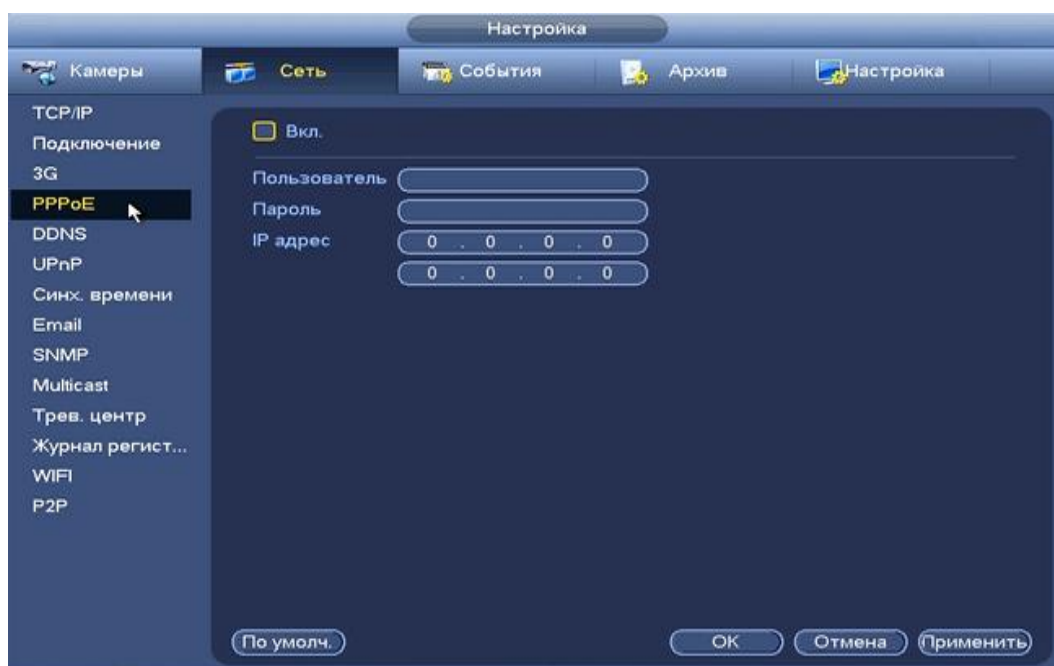
Рисунок 8.3.2.5.1 Интерфейс настройки «PPPoE».
