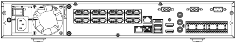
Рисунок 4.2.1 Схема обозначения портов.
