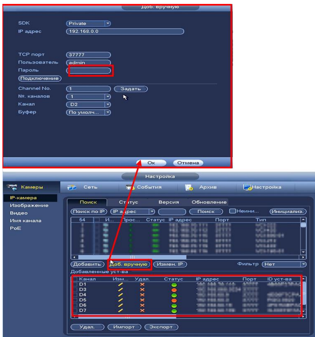
Рисунок 8.3.1.1.3 Настройка ручного добавления камер.
