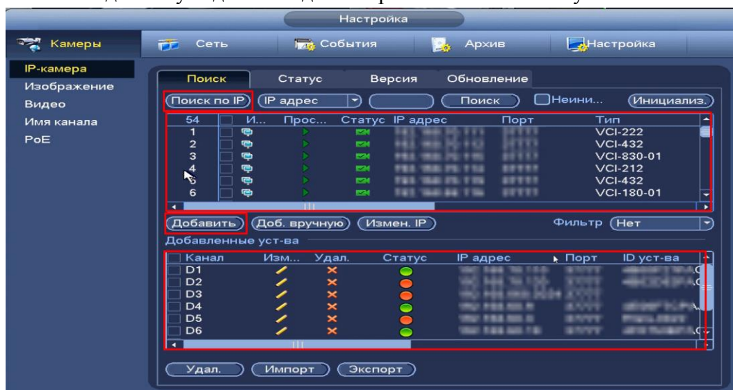
Рисунок 8.3.1.1.1.2 Настройка добавления камер по поиску в сети.
