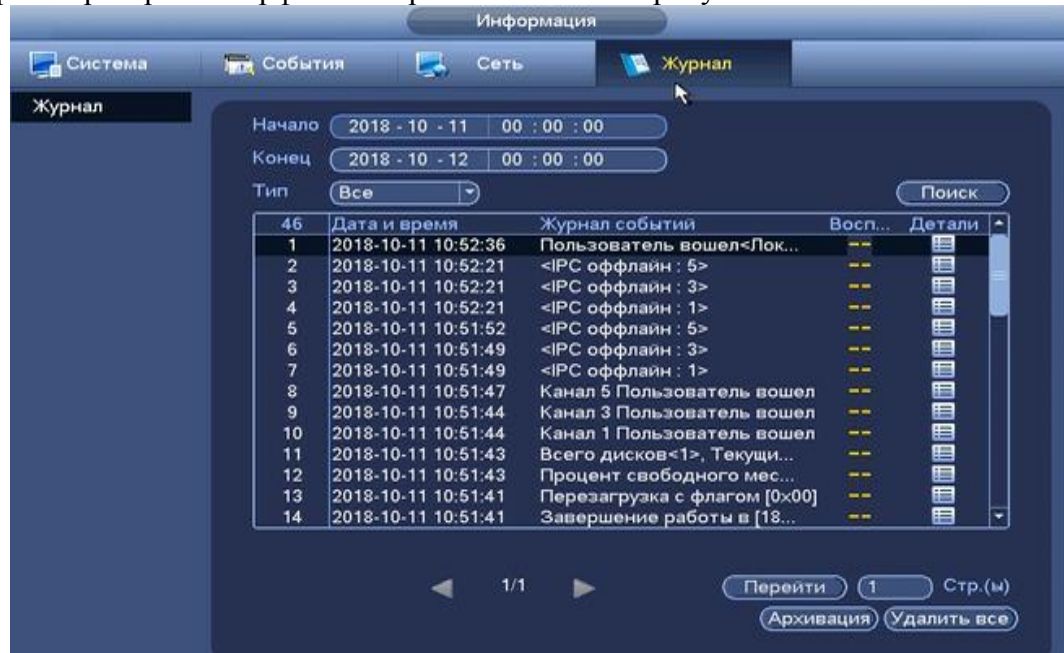
Рисунок 8.2.4.1 Интерфейс просмотра журнала
