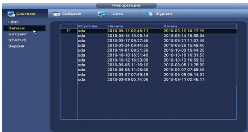
Рисунок 8.2.1.2.1.- Интерфейс просмотра информации о записи.
