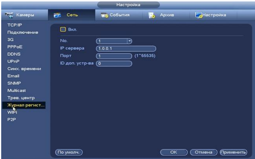
Рисунок 8.3.2.15.1 Интерфейс настройки журнала регистра. Параметры и функции настройки описаны в таблице 8.17.
