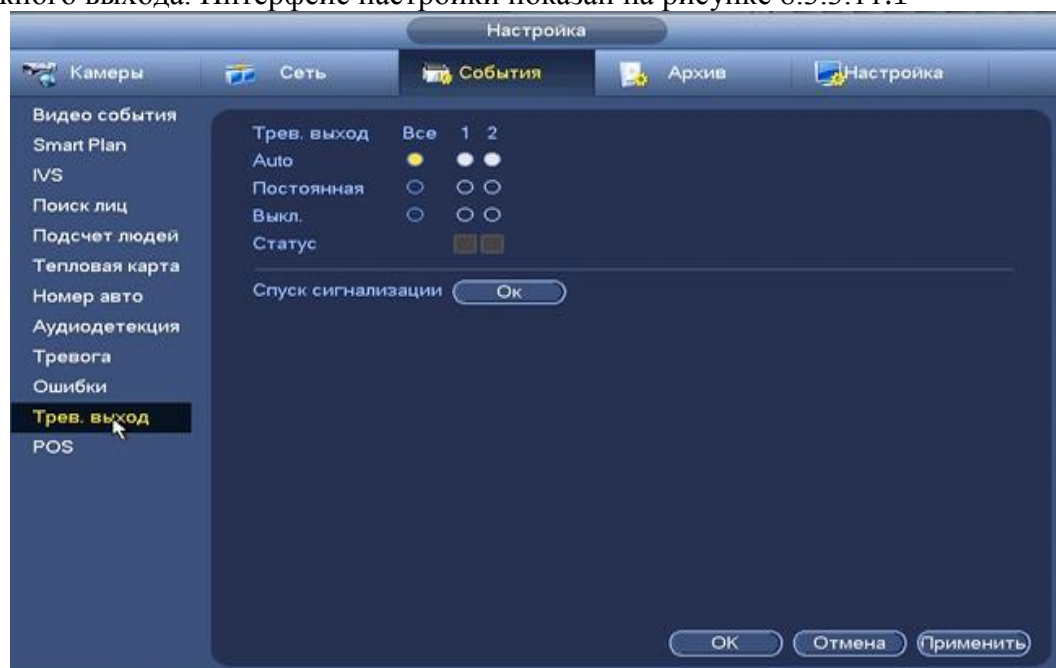
Рисунок 8.3.3.11.1 Интерфейс настройки тревожного выхода.
