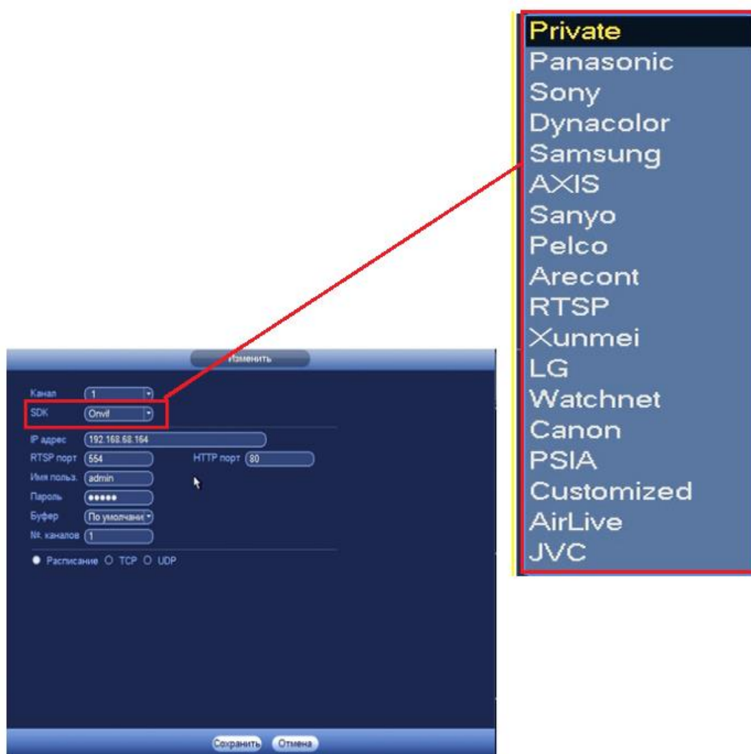
Рисунок 6.2.6.4 Настройка добавления камер сторонних производителей.
