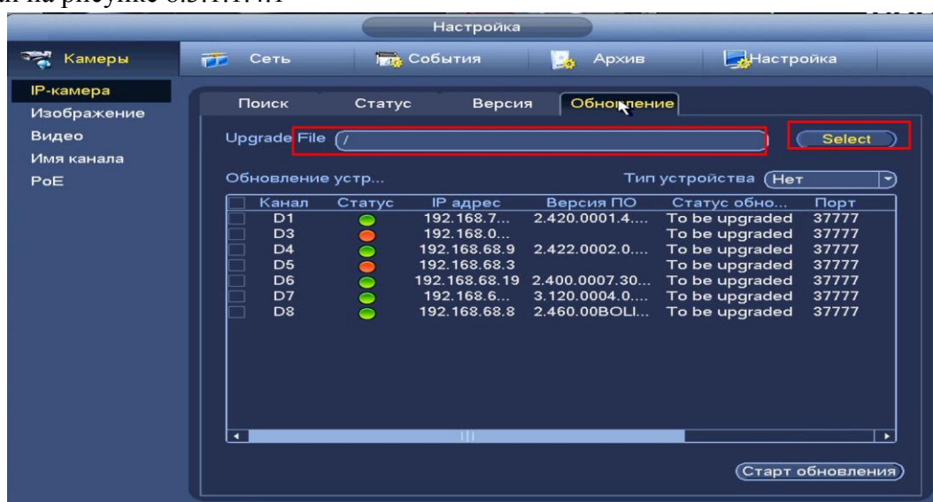
Рисунок 8.3.1.1.4.1 Интерфейс обновления ПО устройств.
