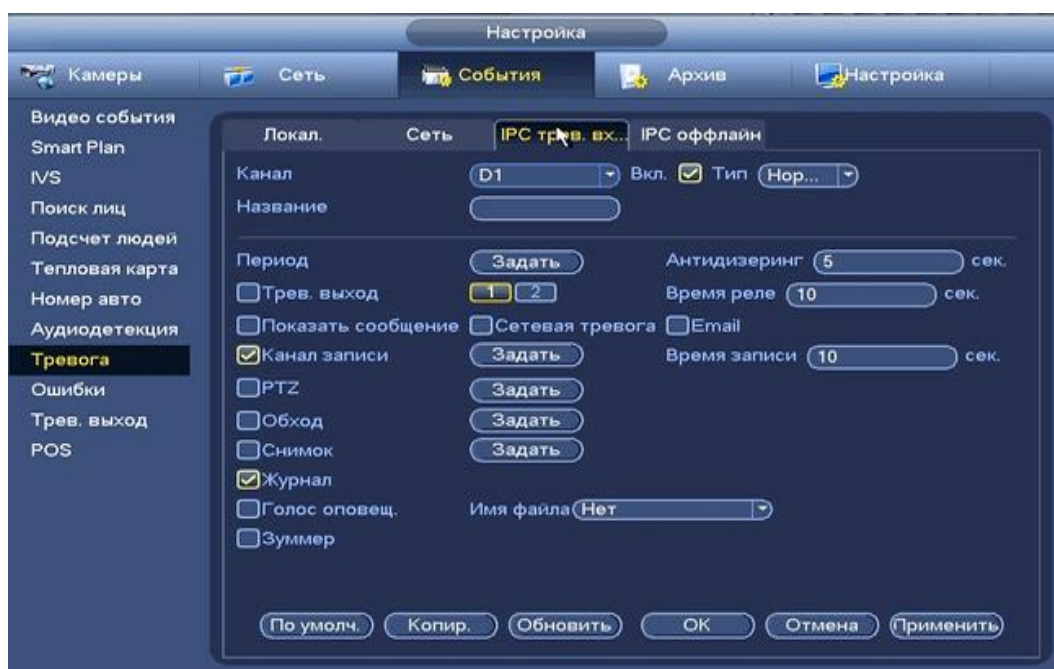
Рисунок 8.3.3.9.3.1 Интерфейс настройки IPC трев.вход.
