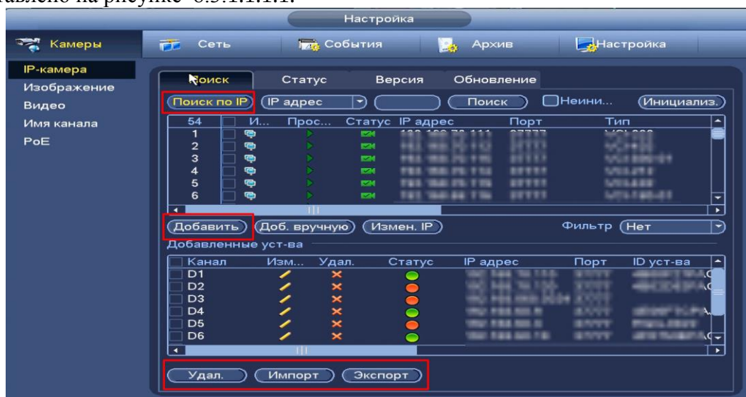
Рисунок 8.3.1.1.1.1 Интерфейс добавления камер к устройству.
