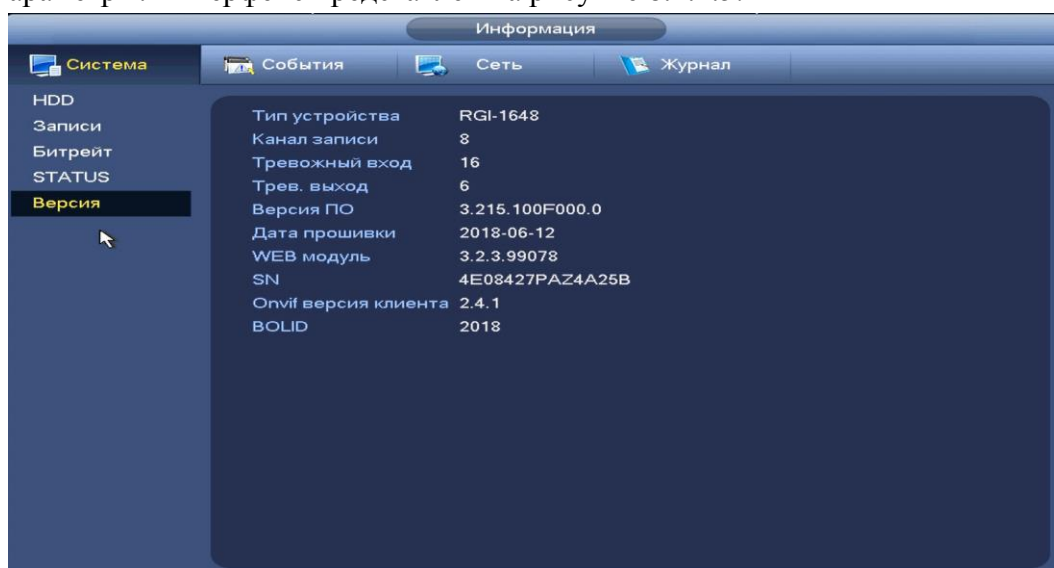
Рисунок 8.2.1.5.1 Интерфейс просмотра информации о версии.
