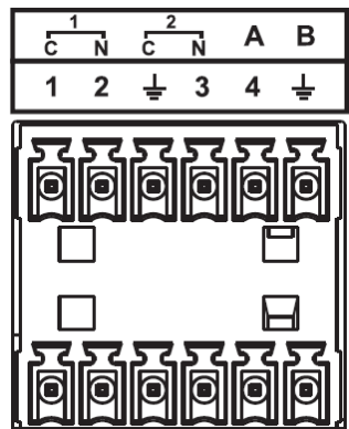
Рисунок 3.3 – Тревожный вход/выход, RS-485
