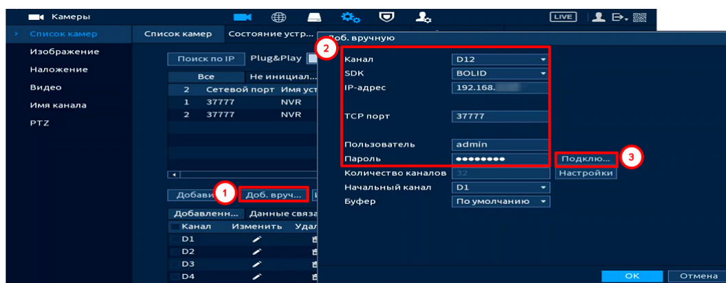
Рисунок 11.18 – Добавление видеопотока с другого регистратора
