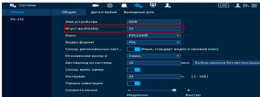
Рисунок 14.6 – Интерфейс установки номера устройства
