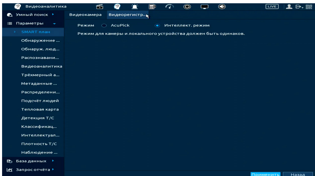
Рисунок 19.11 – Режим работы видеорегистратора «Интеллект. режим»
