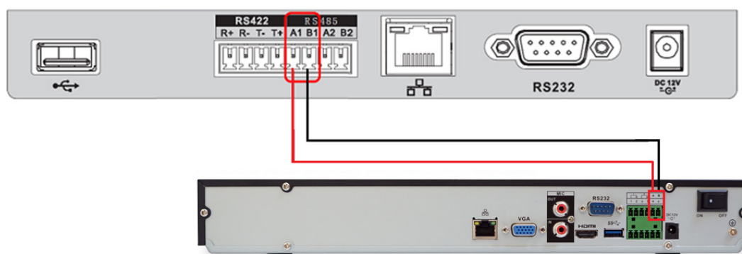
Рисунок 14.4 – Схема RS-485
