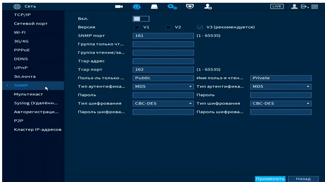
Рисунок 12.11 – Интерфейс настройки «SNMP»
