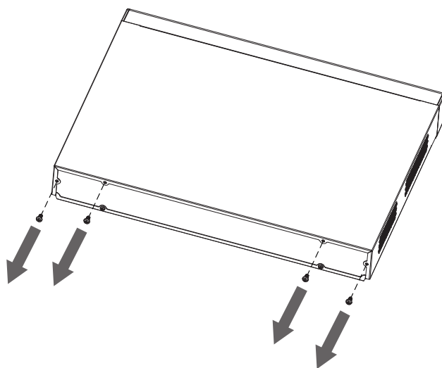
Рисунок 4.2 – Установка жесткого диска
