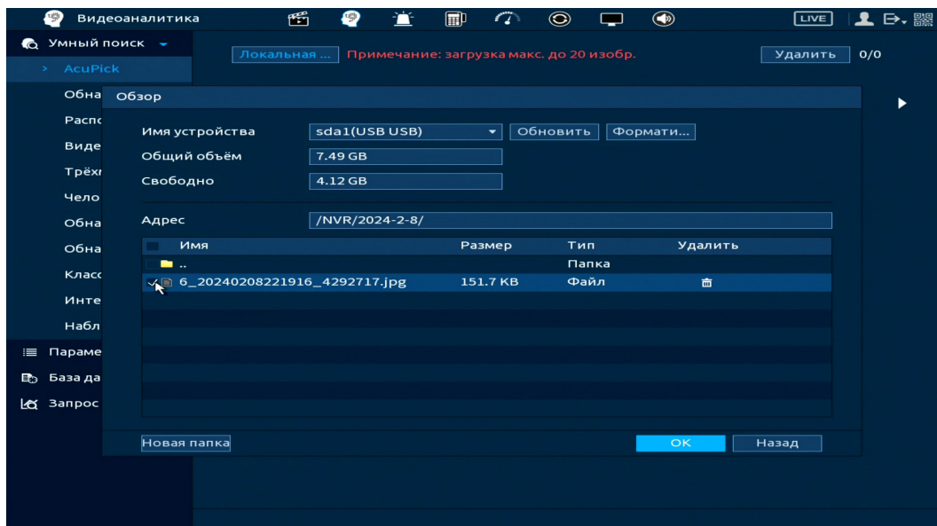
Рисунок 19.8 – АсуРиск. Подраздел «Умный поиск»
