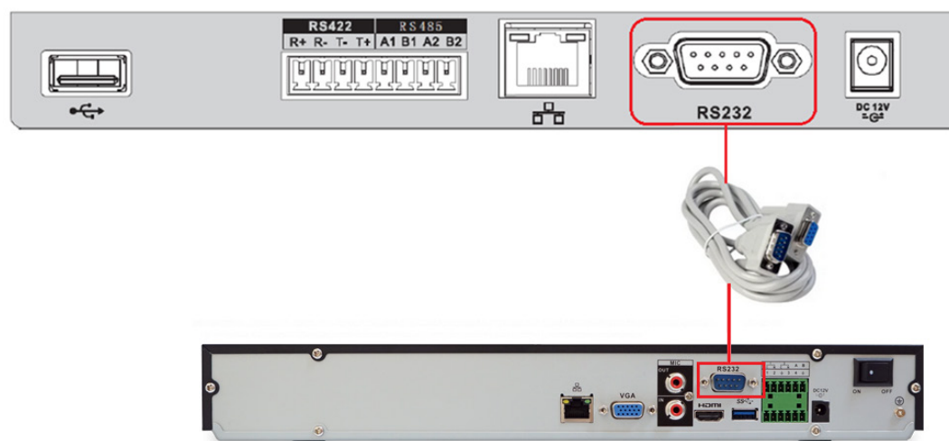
Рисунок 14.5 – Схема RS-232
