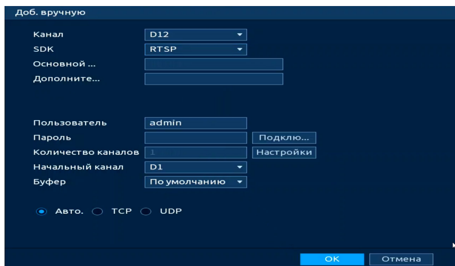
Рисунок 11.17 – Работа со сторонними клиентами по протоколу RTSP
