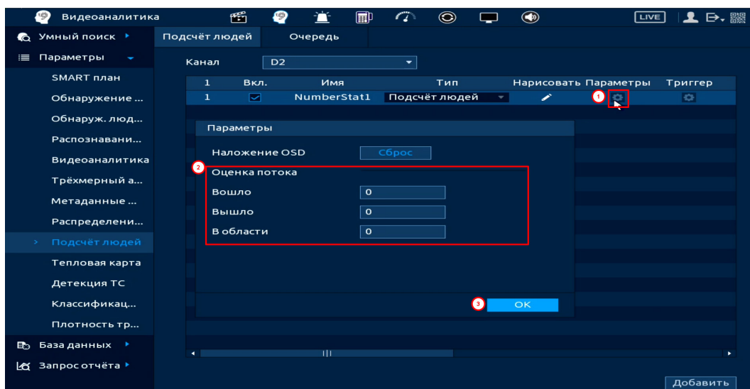
Рисунок 19.98 – Интерфейс настройки подсчёта посетителей
