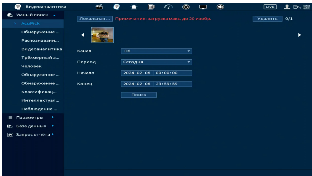
Рисунок 19.9 – AcuPick. Подраздел «Умный поиск»
