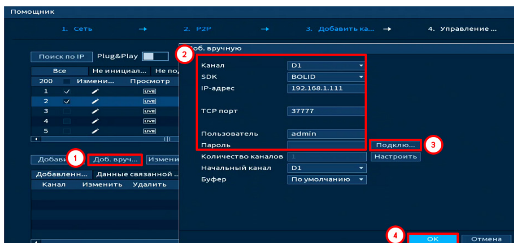
Рисунок 6.12 – Ручной режим добавления
