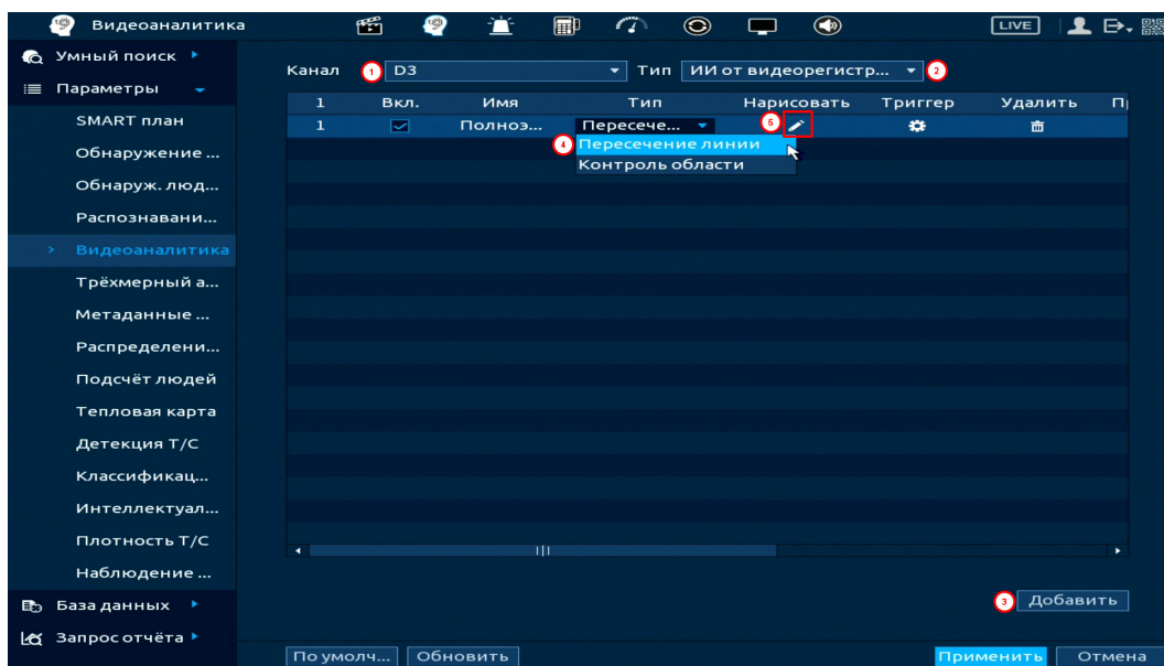
Рисунок 19.35 – Функция видеоаналитики «Пересечение линии»
