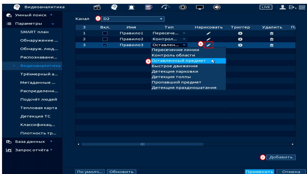
Рисунок 19.50 – Функция видеоаналитики «Оставленный предмет»
