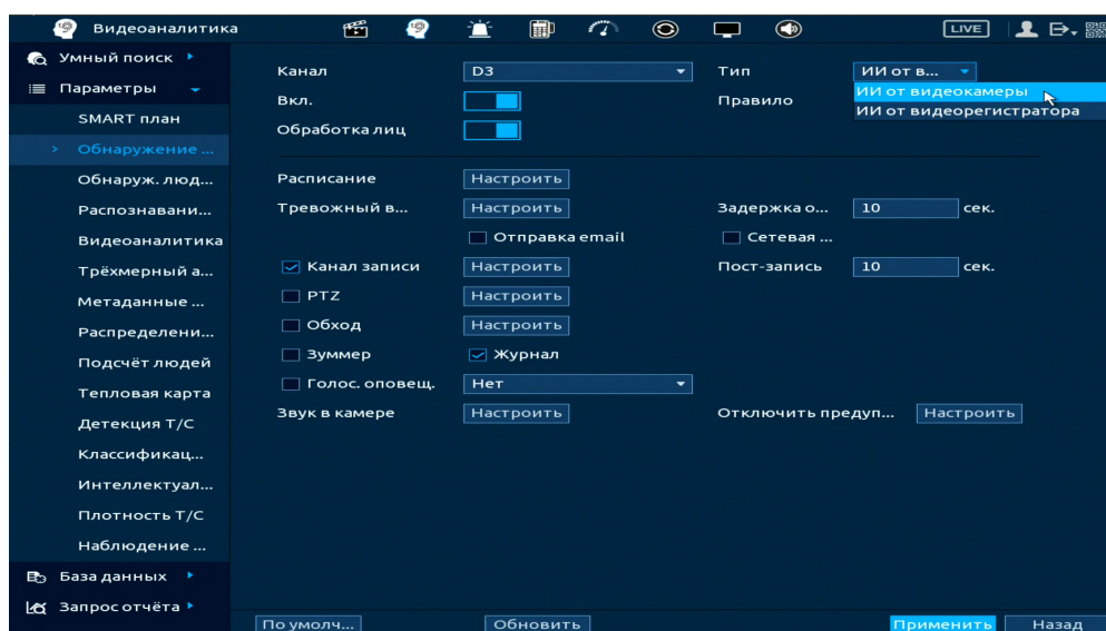
Рисунок 19.12 – Интерфейс настройки обнаружения лиц. ИИ от видеокамеры
