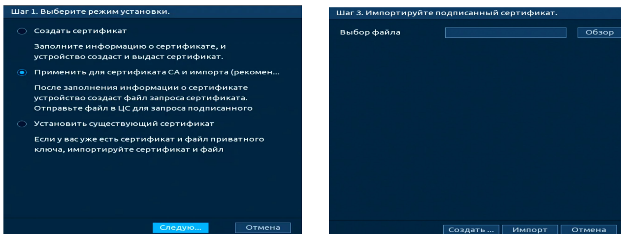
Рисунок 15.18 – Создание и импорт доверенного сертификата
