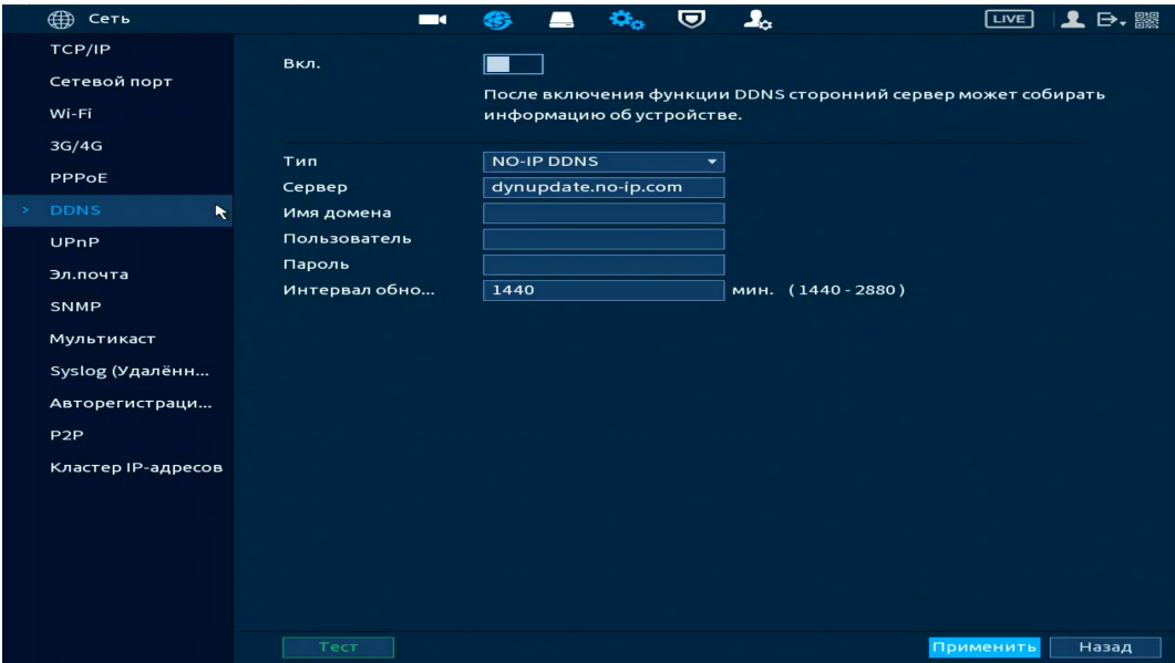
Рисунок 12.8 – Интерфейс настройки «DDNS»
