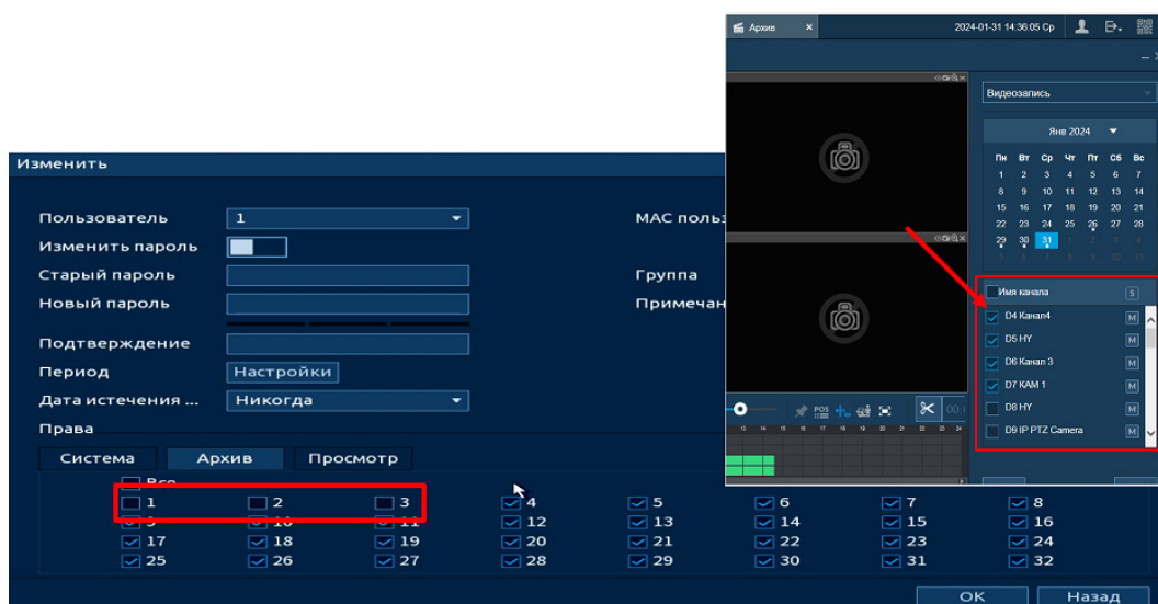
Рисунок 16.3 – Снят доступ для просмотра архива пользователем (каналы D1, D2 и D3)
