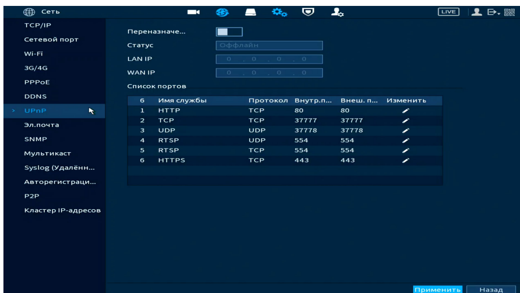
Рисунок 12.9 – Интерфейс настройки «UPnP»
