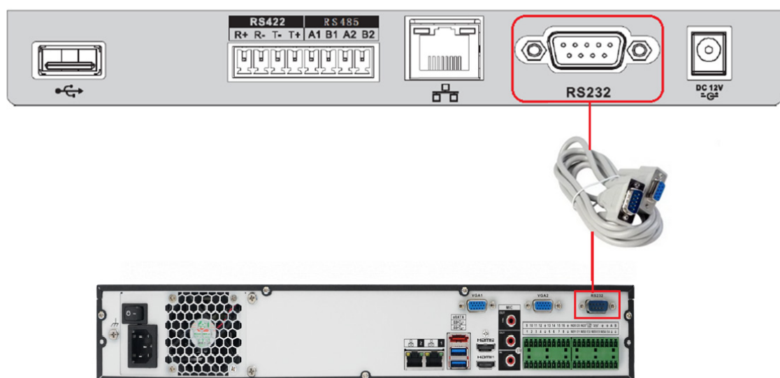
Рисунок 14.5 – Схема RS-232
