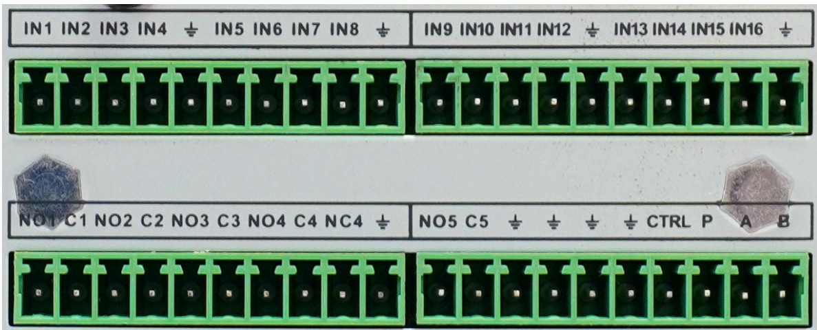
Рисунок 3.3 – Тревожный вход/выход, RS-485
