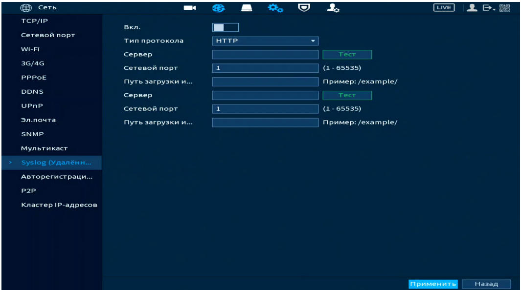
Рисунок 12.14 – Интерфейс настройки «HTTP»
