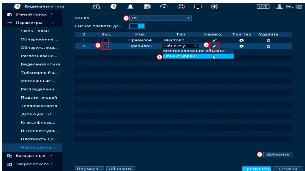
Рисунок 19.138 – Функция видеоаналитики «Пропавший предмет»
