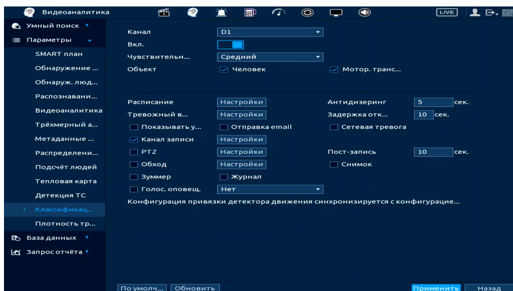
Рисунок 19.124 – Классификация объектов
