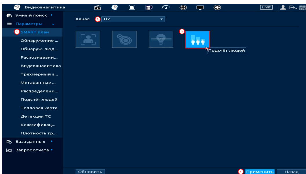
Рисунок 19.111 – Настройка
