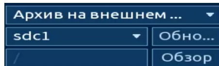
Рисунок 17.20 – Тип поиска
