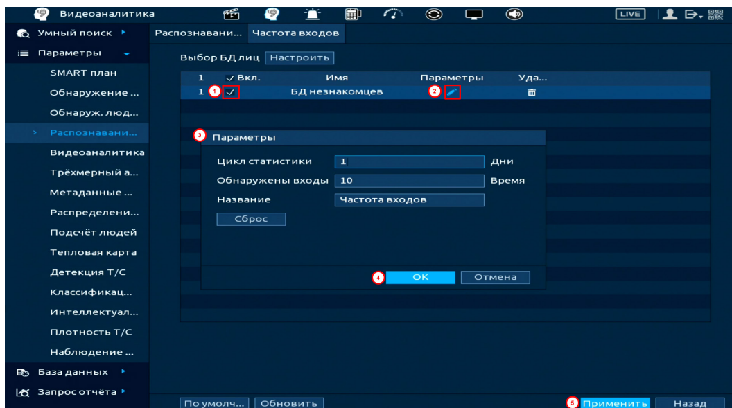
Рисунок 19.31 – Настройка
