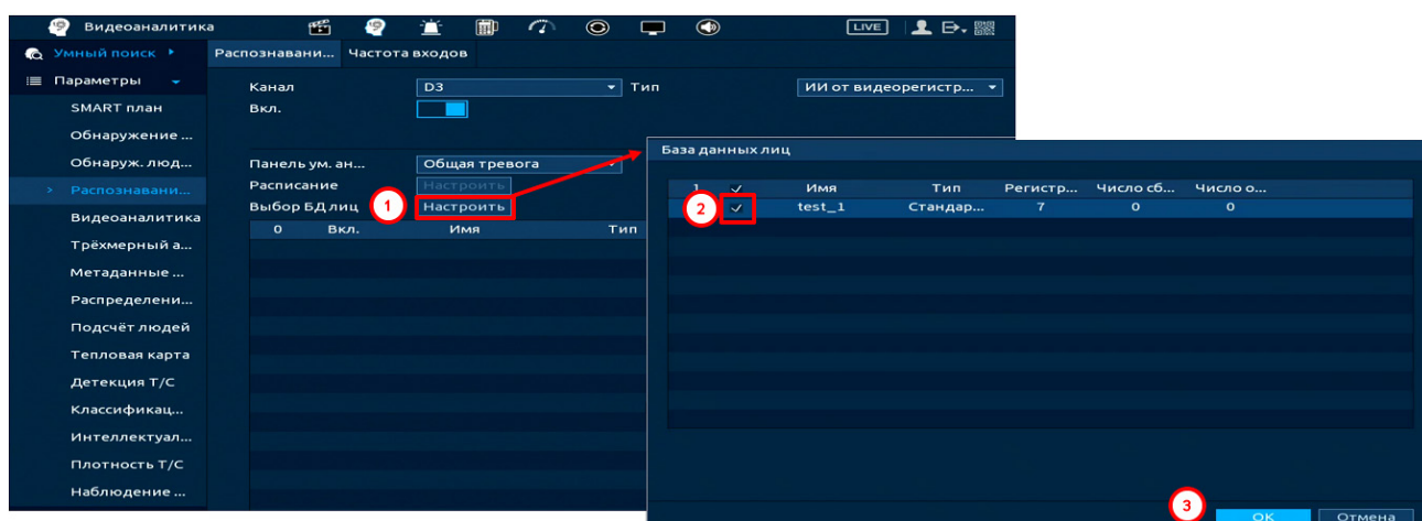
Рисунок 19.21 – Настройка
