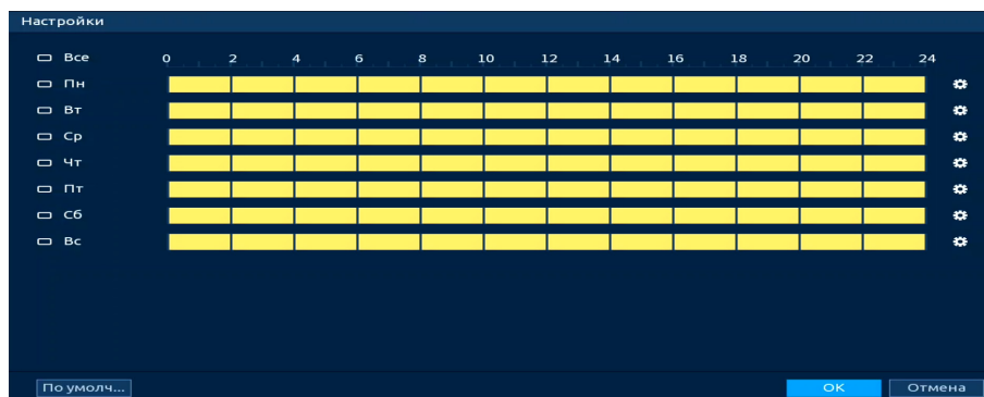
Рисунок 18.39 – Панель расписания
