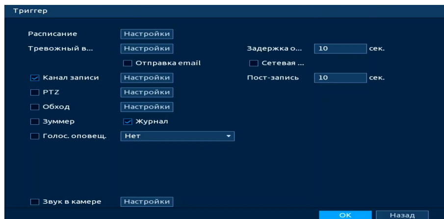
Рисунок 19.52 – Настройка
