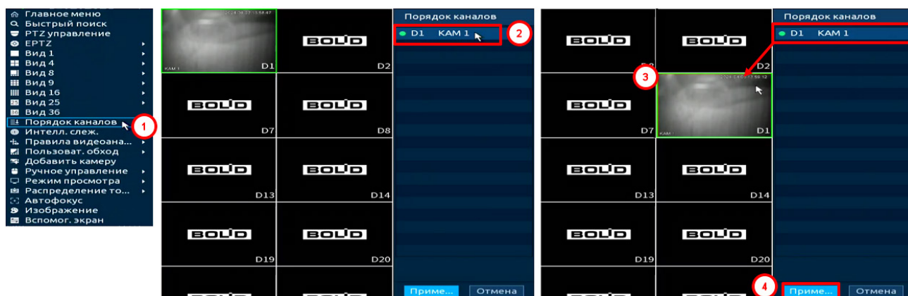
Рисунок 7.6 – Изменение раскладки
