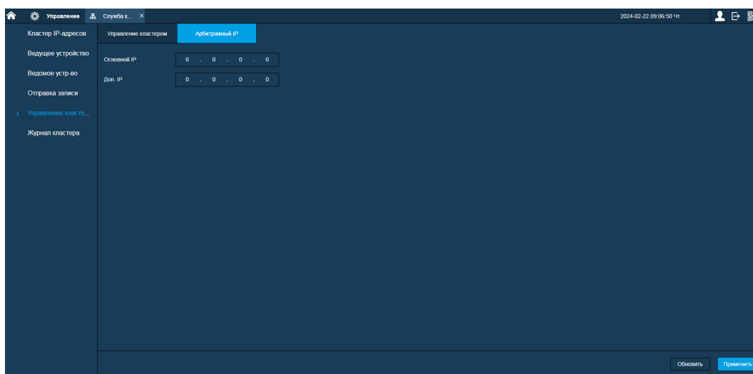
Рисунок 12.29 – Арбитражный IP-адрес
