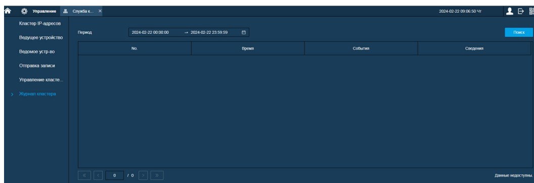
Рисунок 12.30 – Журнал кластера
