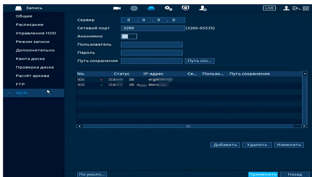
Рисунок 13.30 – Настройка iSCSI
