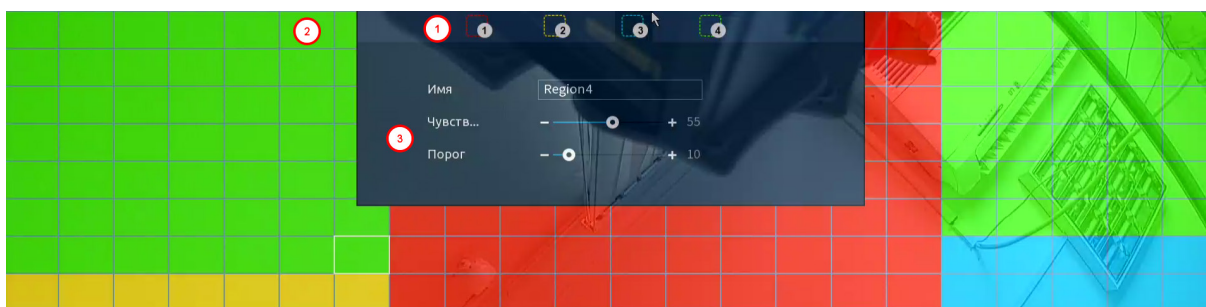
Рисунок 18.20 – Настройка области
