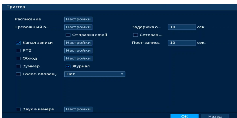
Рисунок 19.116 – Настройка
