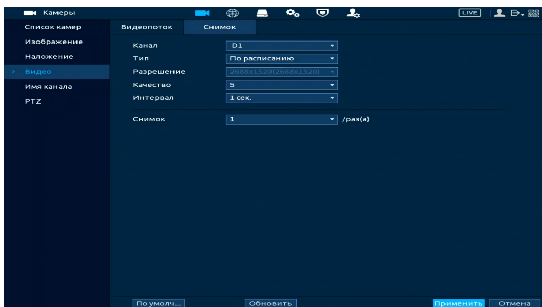
Рисунок 11.32 – Настройка снимка
