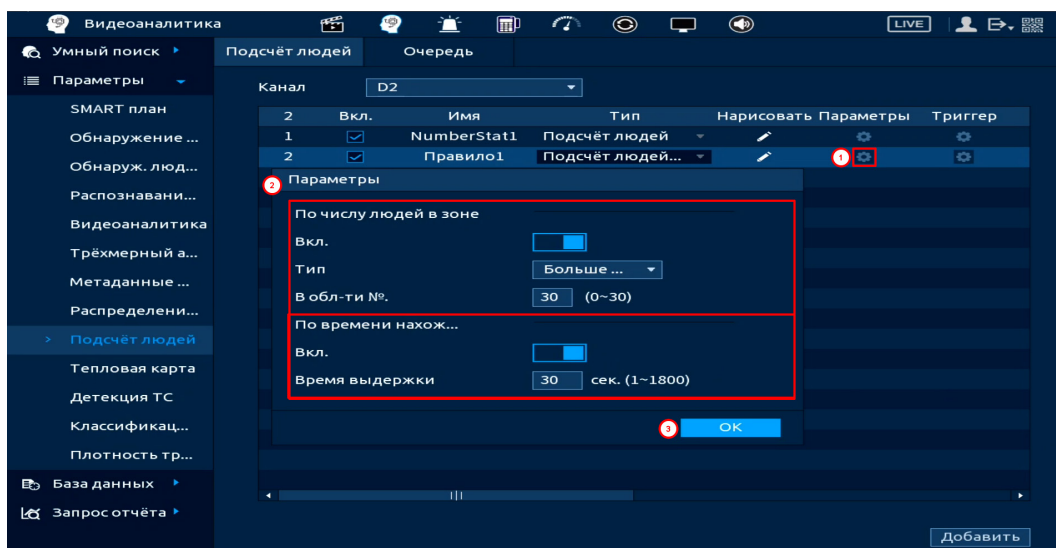
Рисунок 19.107 – Настройка параметров
