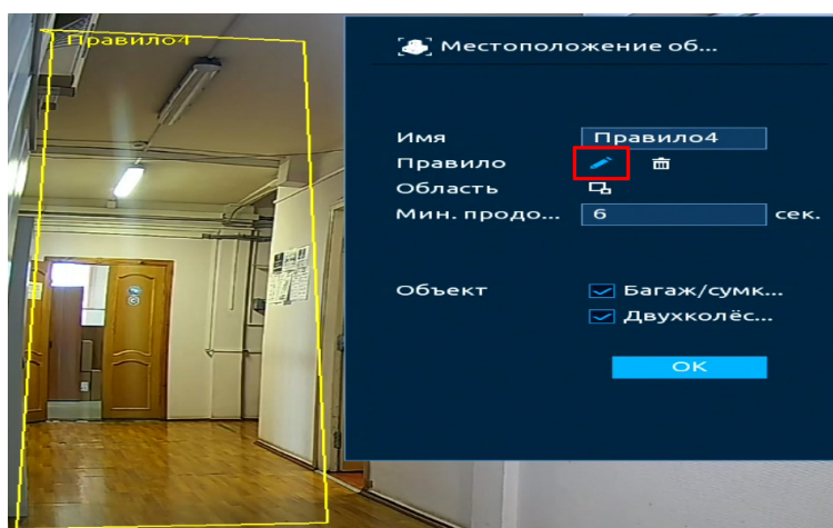
Рисунок 19.131 – Настройка
