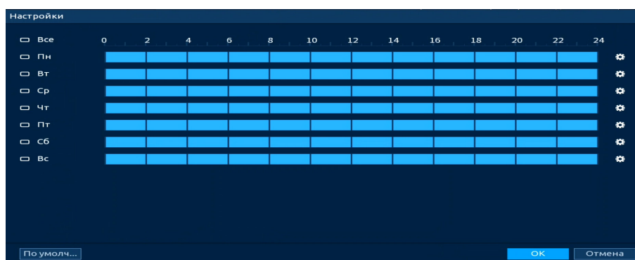
Рисунок 19.101 – Расписание
