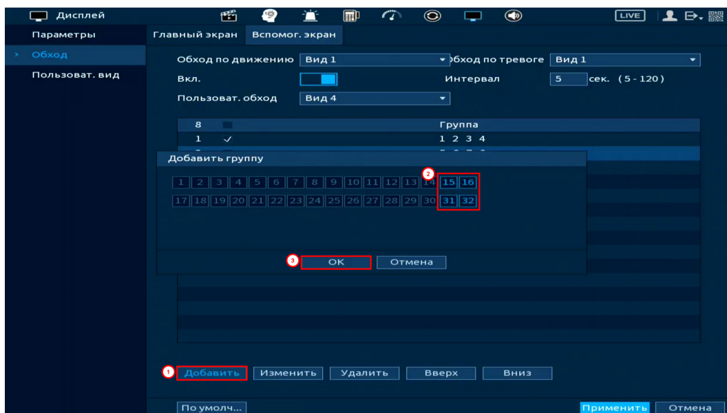
Рисунок 9.13 – Добавление группы
