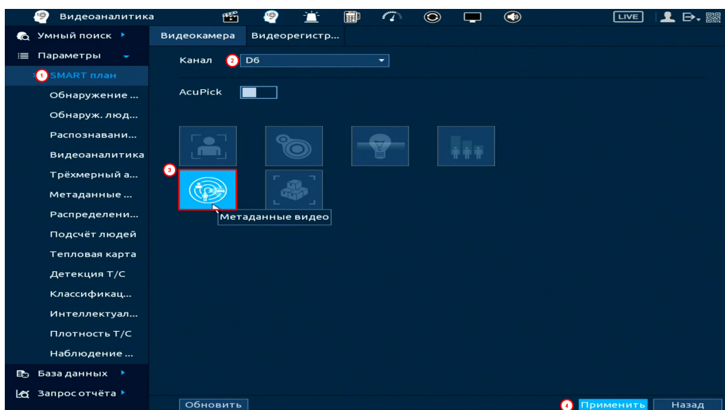
Рисунок 19.85 – Настройка
