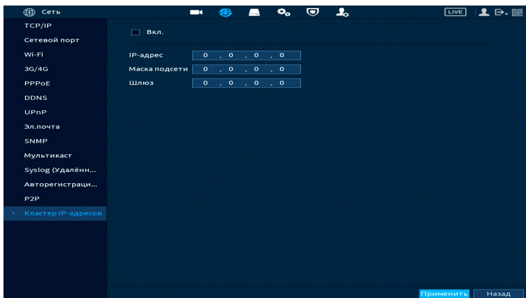
Рисунок 12.24 – Локальный интерфейс. Кластер IP-адресов
