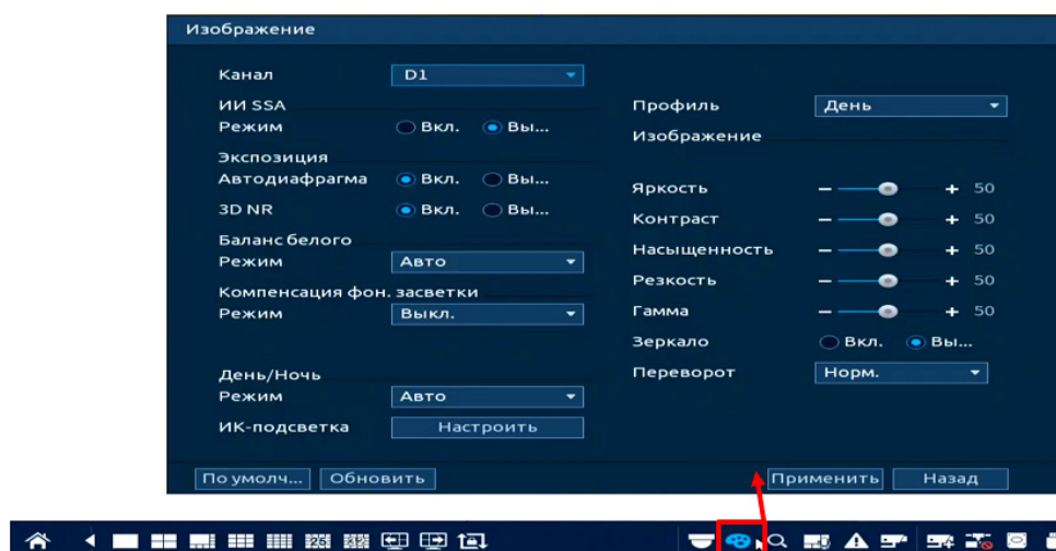
Рисунок 11.28 – Переход в меню редактирования изображения через панель навигации
