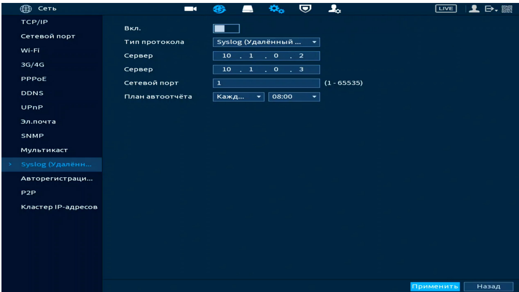
Рисунок 12.15 – Интерфейс настройки «Удалённый журнал»
