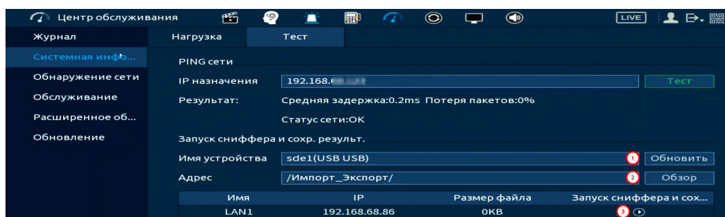
Рисунок 20.11 – Настройка пути сохранения данных
