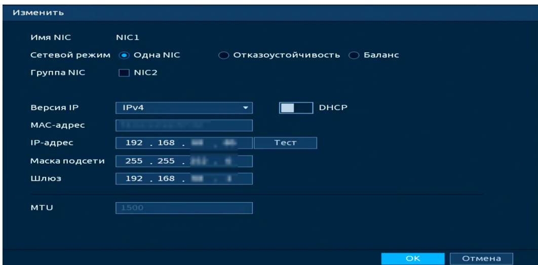
Рисунок 12.2 – Интерфейс настройки «Сеть»
