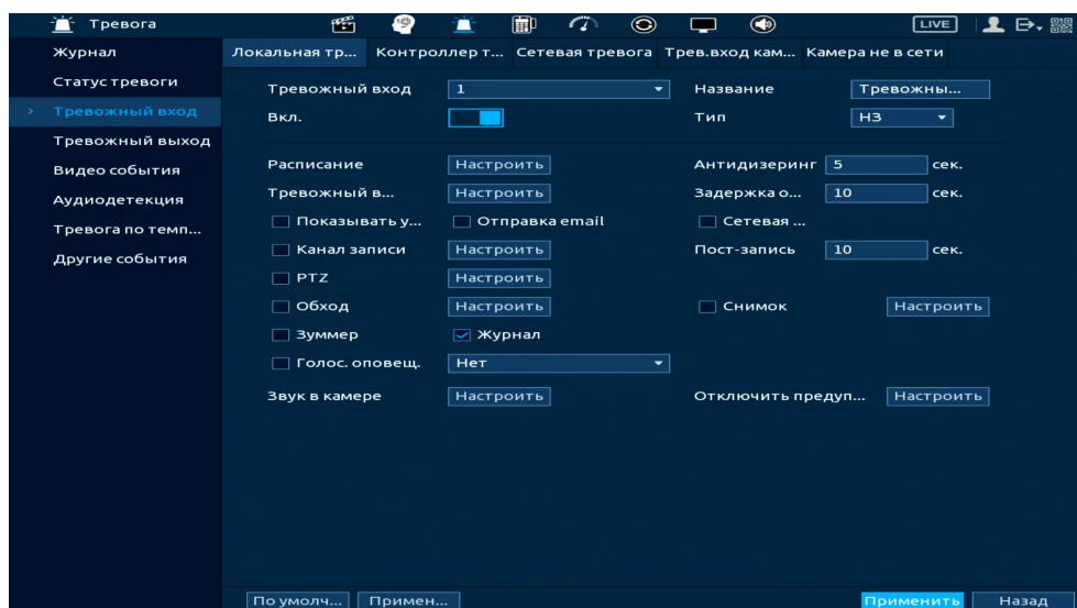
Рисунок 18.3 – Интерфейс настройки локальной тревоги
