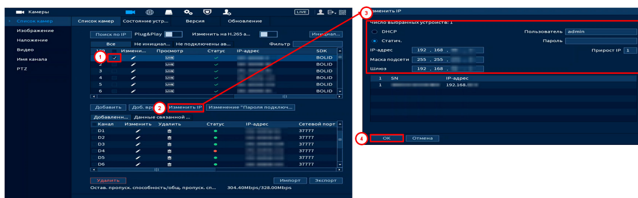
Рисунок 11.21 – Изменения сетевых настроек IP-камер через видеорегистратор
