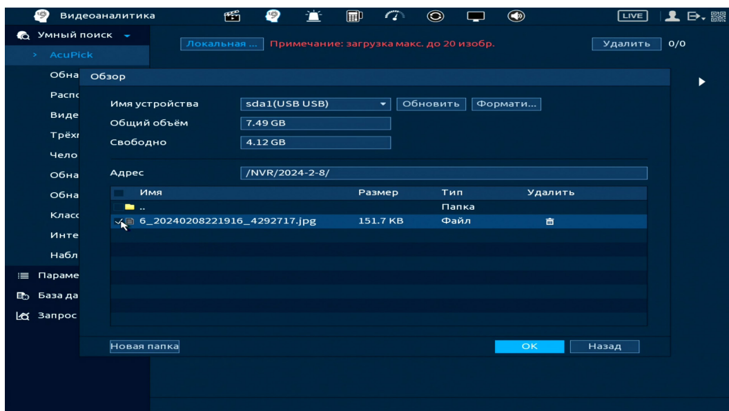
Рисунок 19.8 – AcuPick. Подраздел «Умный поиск»
