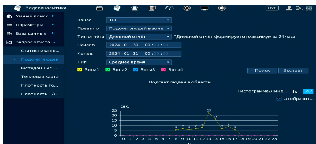
Рисунок 19.169 – Статистика по времени
