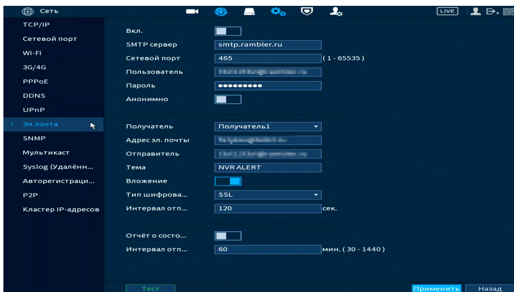
Рисунок 12.11 – Интерфейс настройки «Электронная почта»
