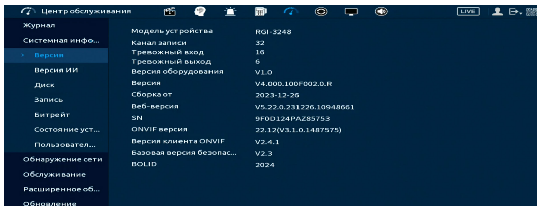
Рисунок 20.2 – Интерфейс просмотра информации о версии
