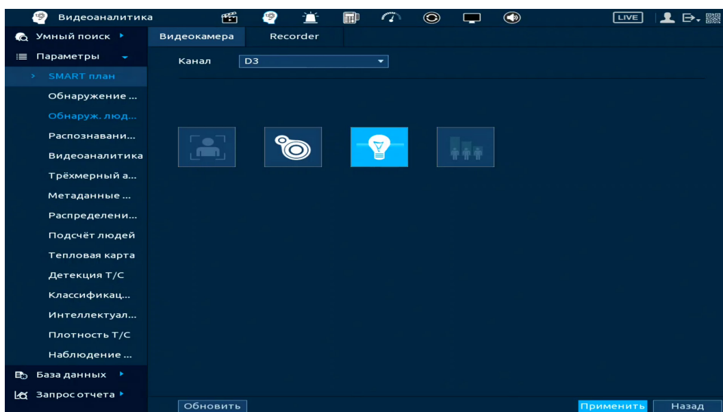
Рисунок 19.1 – Выбор ИИ с камеры
