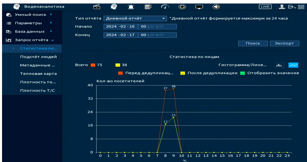
Рисунок 19.166 – Интерфейс просмотра собранной статистики по лицам
