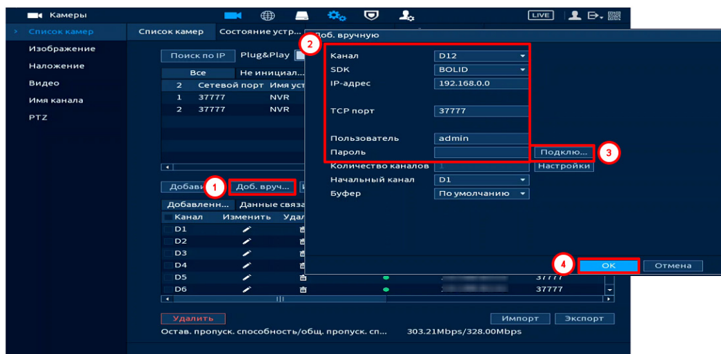
Рисунок 11.16 – Интерфейс ручного добавления удалённого устройства
