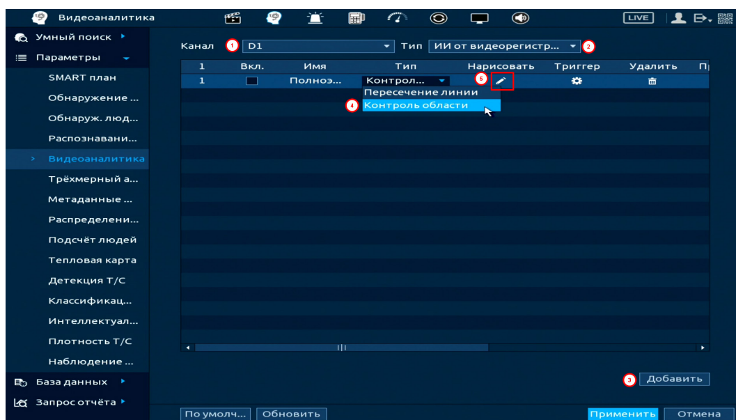
Рисунок 19.42 – Функция видеоаналитики «Контроль области»
