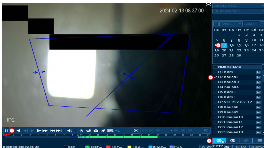
Рисунок 17.16 – Настройка EPTZ
