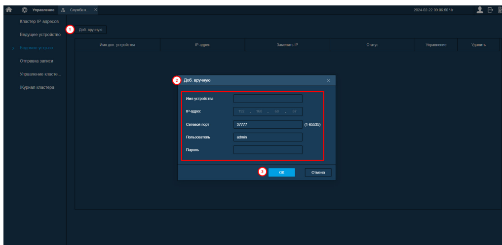
Рисунок 12.26 – Ведущее устройство
