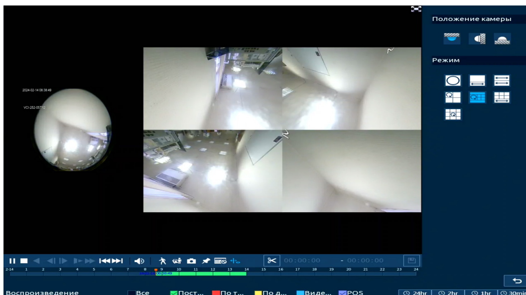
Рисунок 17.15 – Настройка FishEye
