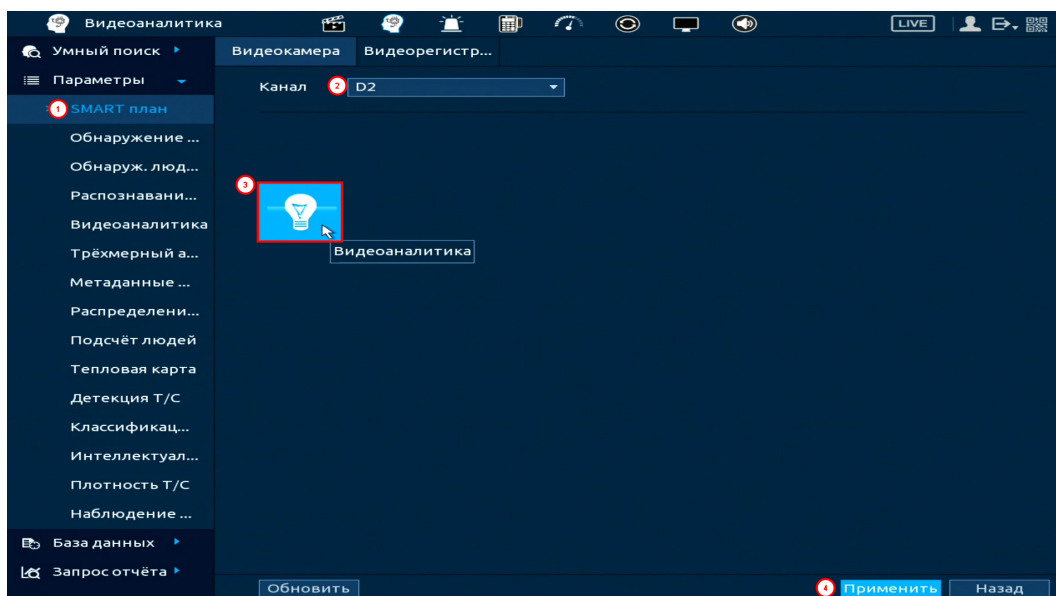
Рисунок 19.34 – Настройка
