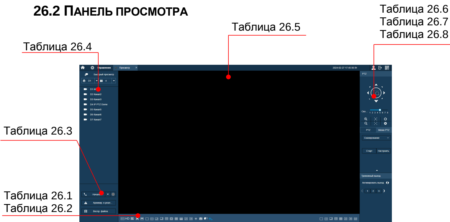
Рисунок 26.1 – Режим просмотра
