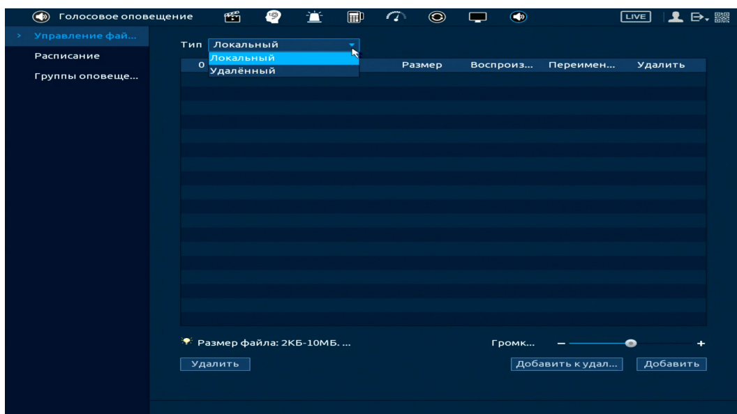
Рисунок 24.1 – Управление файлами
