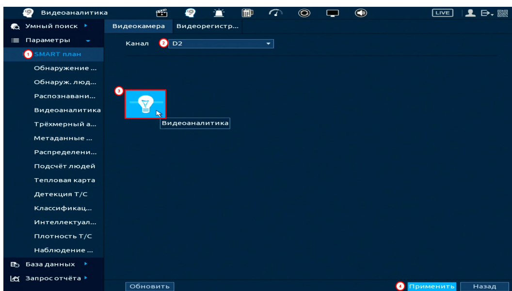
Рисунок 19.41 – Настройка
