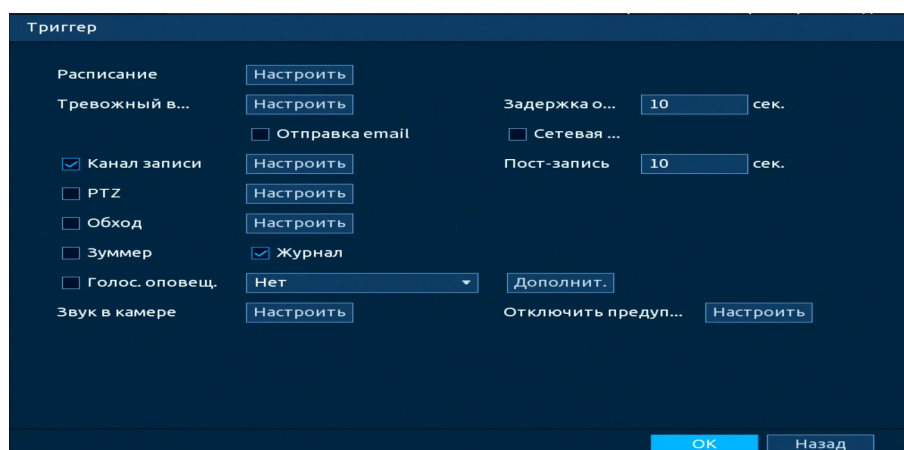
Рисунок 19.46 – Настройка
