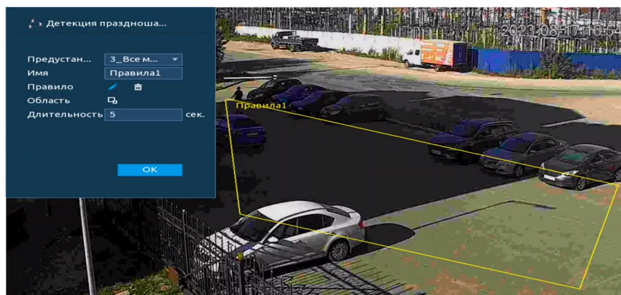
Рисунок 19.81 – Настройка правила
