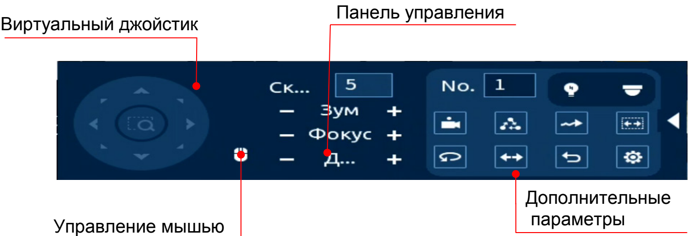
Рисунок 8.3 – Панель PTZ-управления
