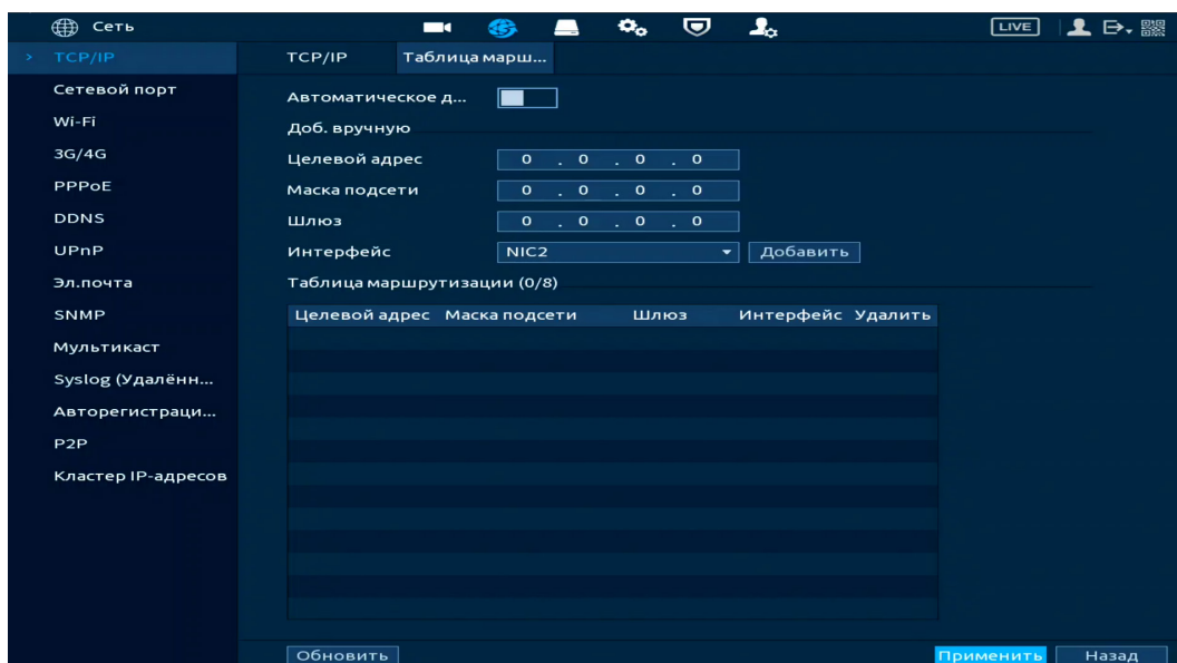
Рисунок 12.3 – Интерфейс настройки «Таблица маршрутизации»
