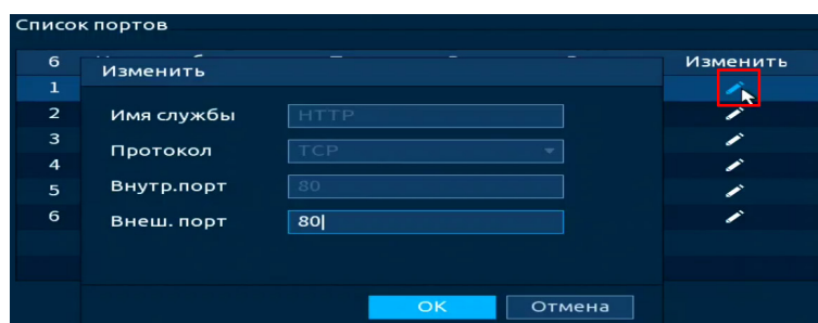
Рисунок 12.10 – Интерфейс настройки «UPnP»
