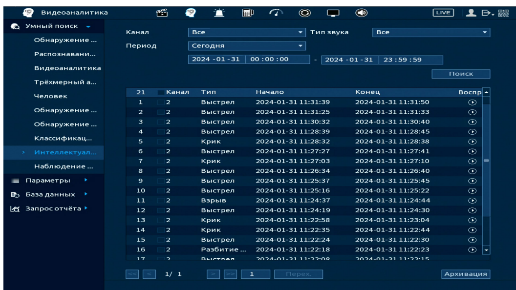
Рисунок 19.164 – Архив видеороликов «Интеллектуальное обнаружение звука»
