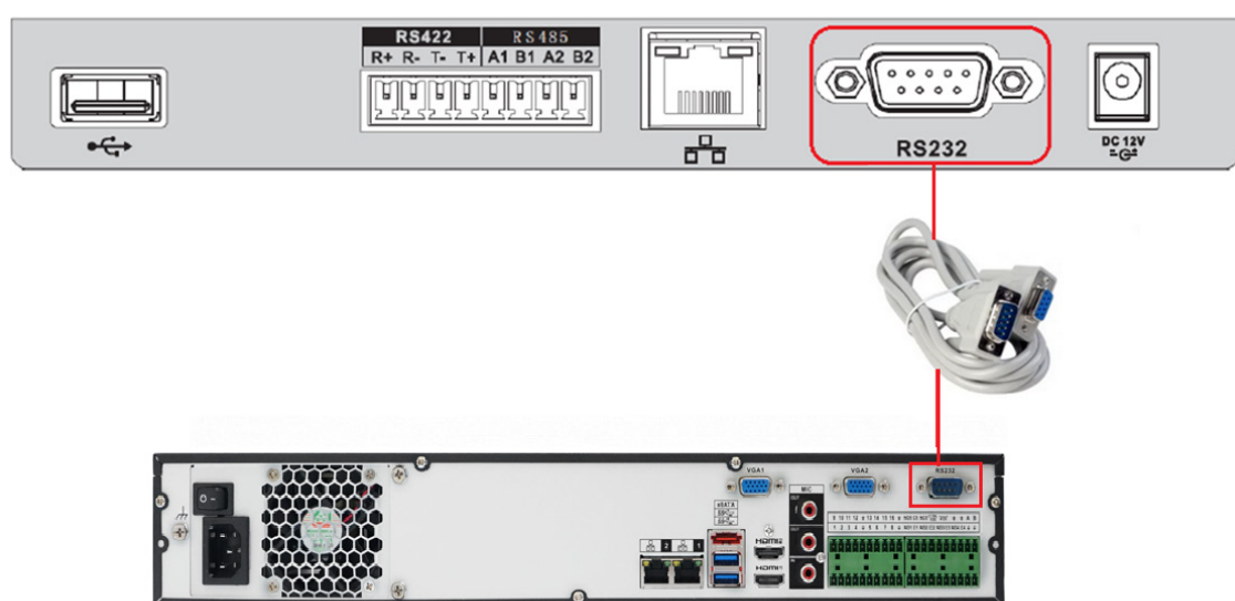
Рисунок 14.5 – Схема RS-232
