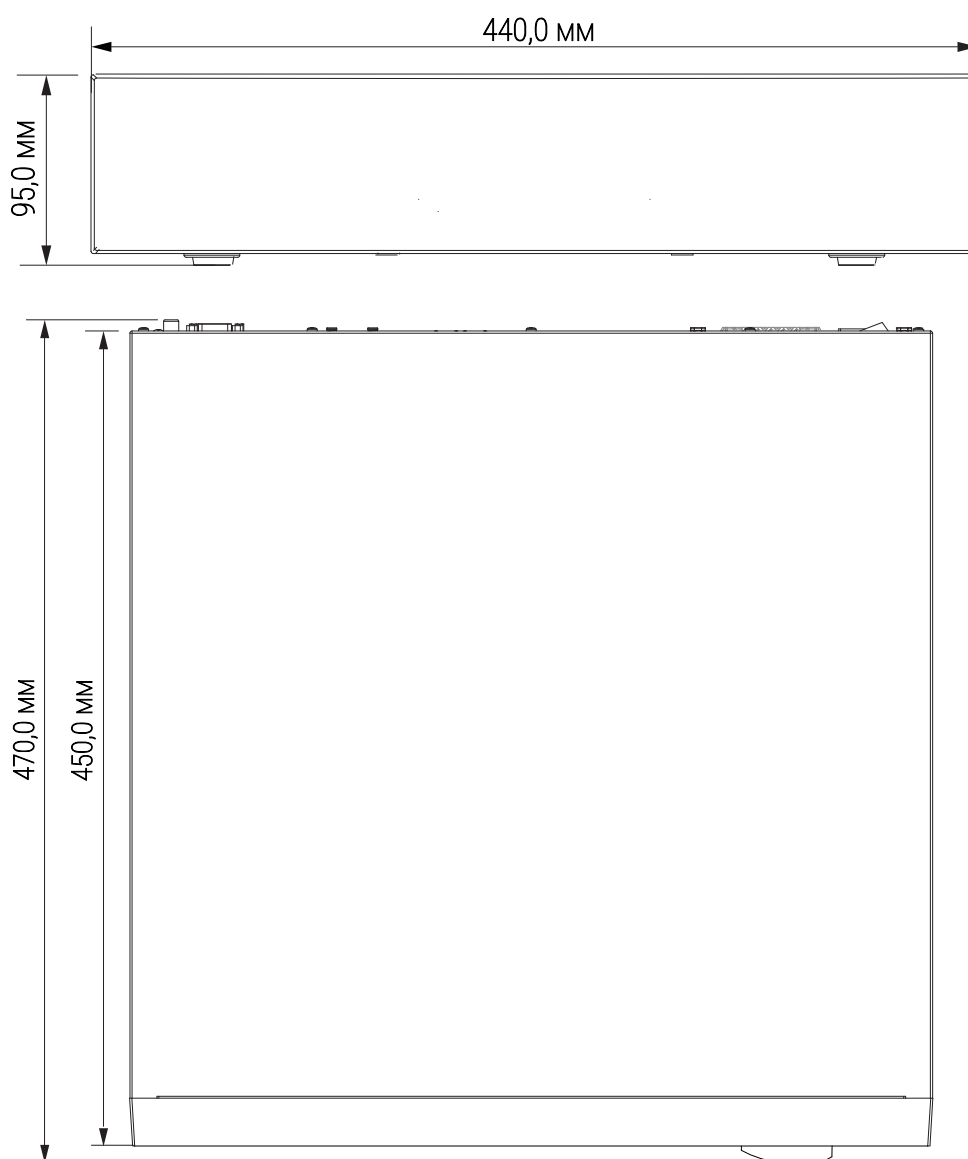
Рисунок 4.1 – Габаритные размеры видеорегистратора
