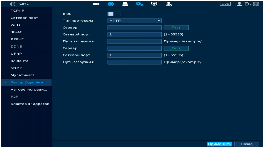
Рисунок 12.14 – Интерфейс настройки «HTTP»
