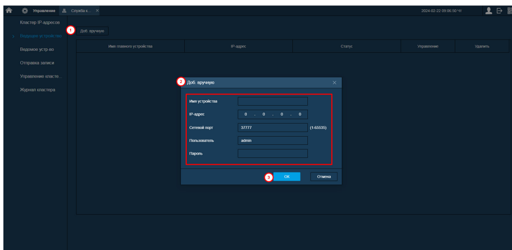
Рисунок 12.25 – Добавление «ведущего» устройства
