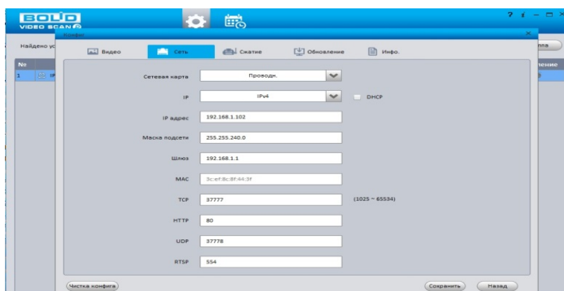
Рисунок 27.2 – Изменение IP-адреса с помощью утилиты «BOLID VideoScan»
