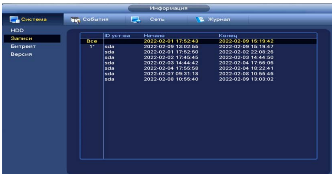
Рисунок 15.20 – Информационный пункт меню «Запись»
