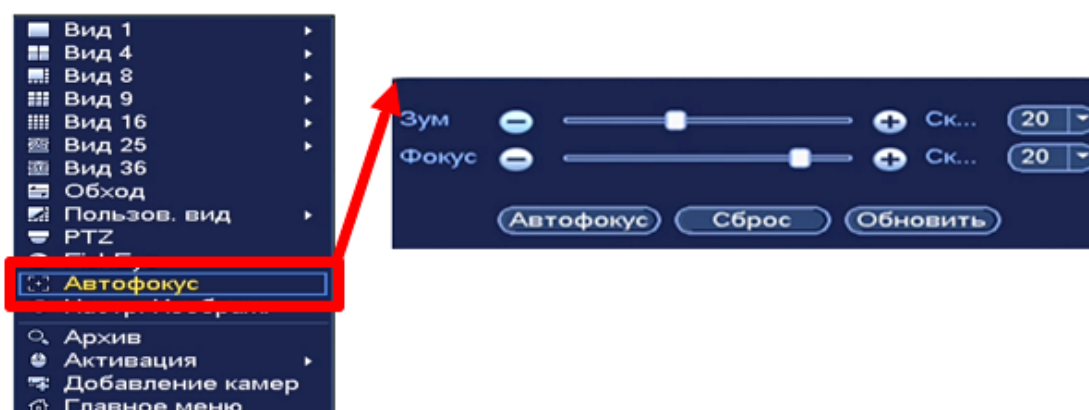
Рисунок 6.8 – Интерфейс настройки контекстного меню «Автофокус»
