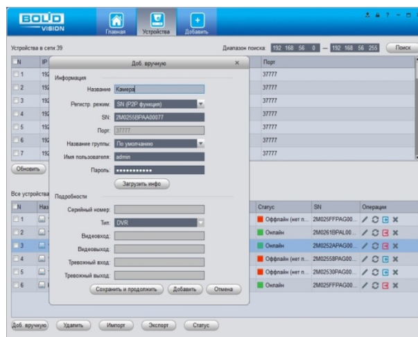
Рисунок 10.13 – Раздел «Устройства» программы «BOLID VISION»
