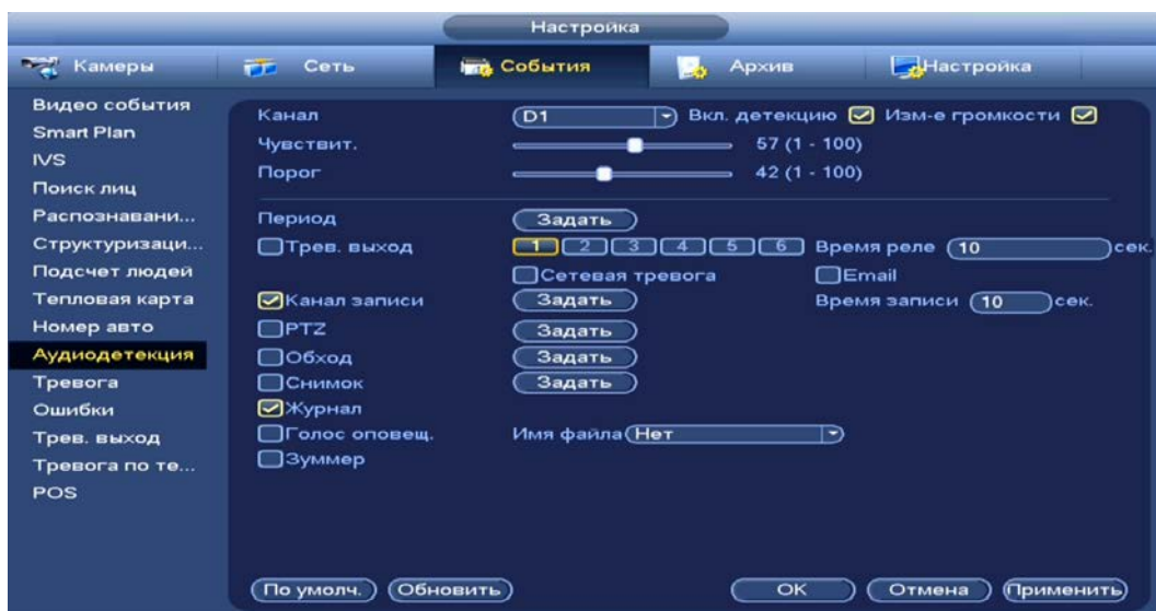
Рисунок 18.28 – Настройка аудиодетекция
