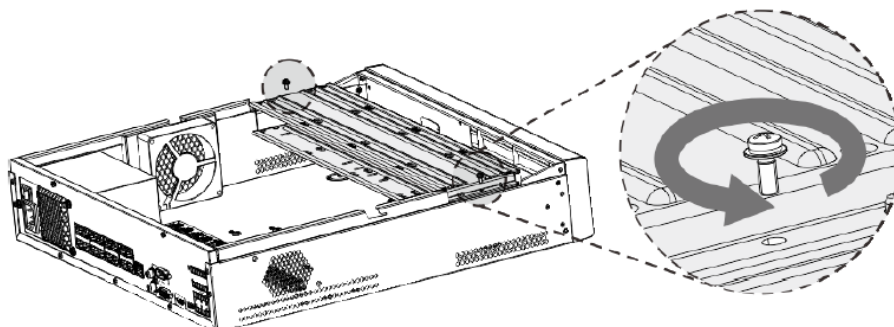
Рисунок 3.5 – Установка жесткого диска
