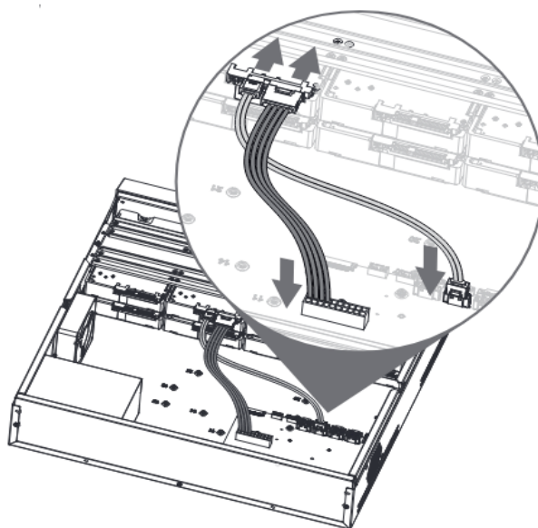
Рисунок 3.8 – Установка жесткого диска
