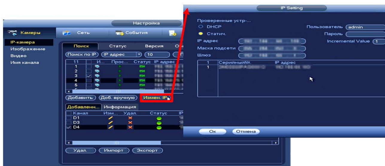
Рисунок 11.12 – Изменения сетевых настроек IP-камер через регистратор
