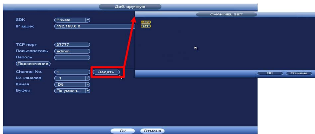
Рисунок 11.11 – Добавление видеопотока с другого регистратора
