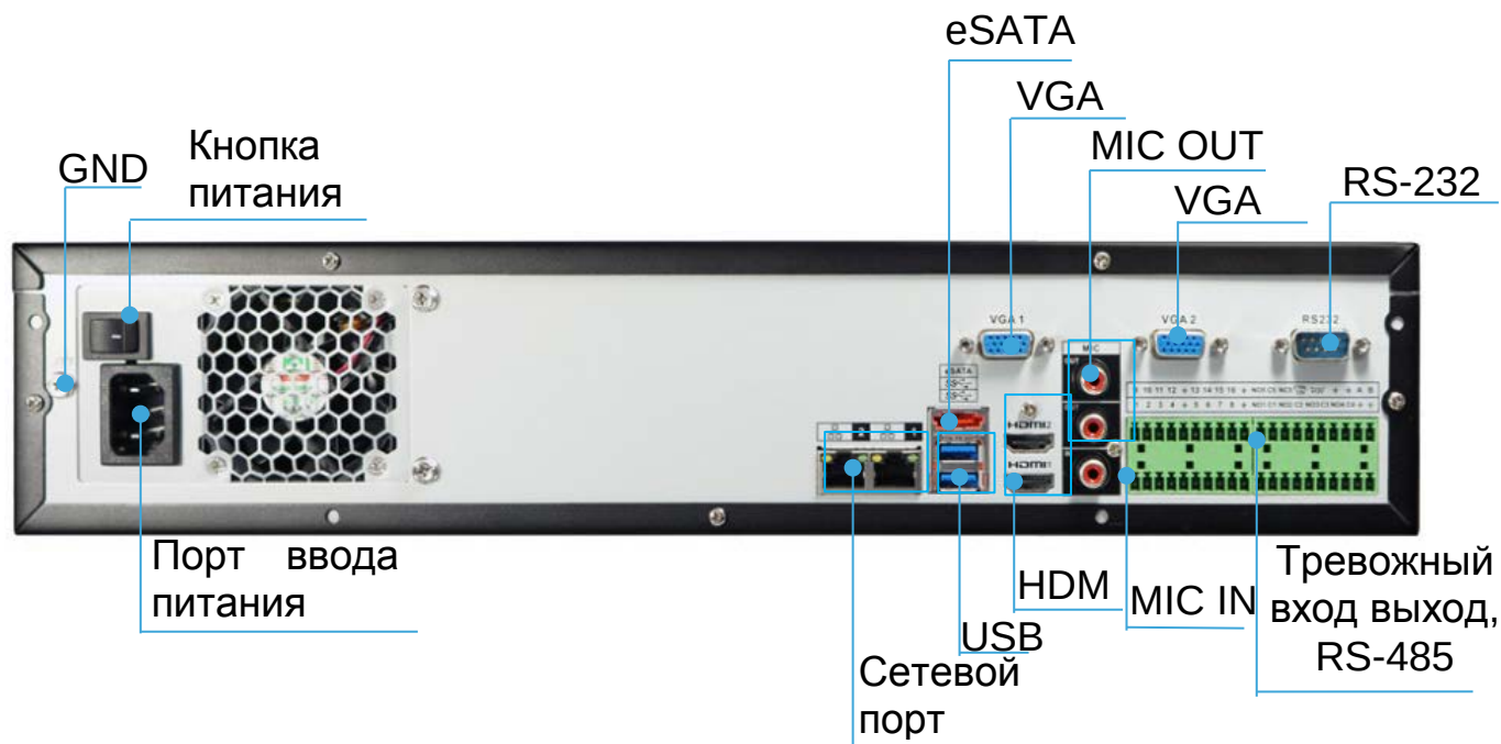
Рисунок 3.2 – Внешний вид задней панели корпуса
