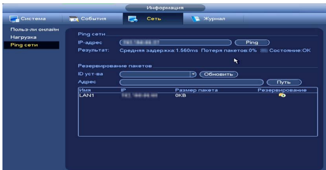
Рисунок 11.17 – Проверка IP-адреса
