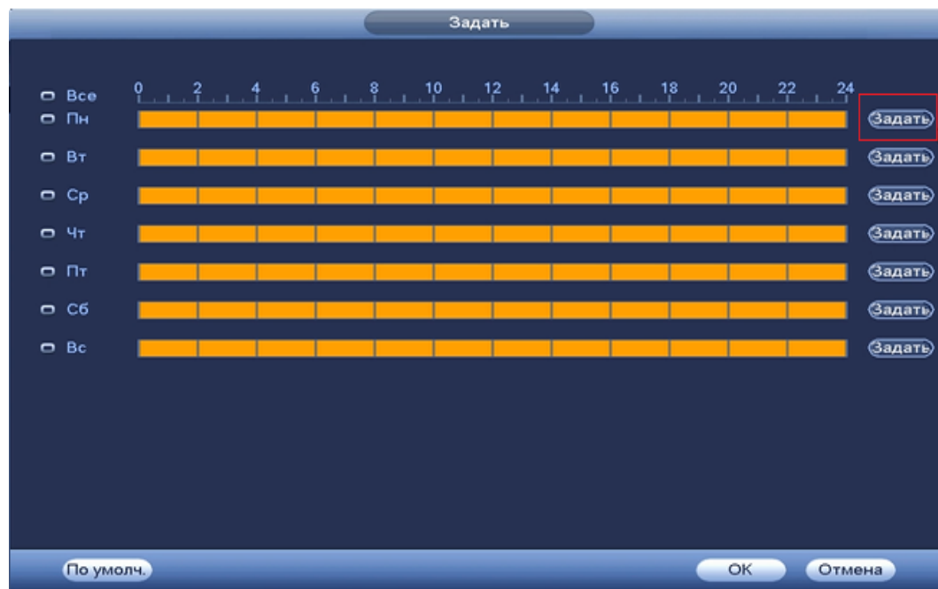
Рисунок 8.3.3.1.2.2 Настройка расписания.
