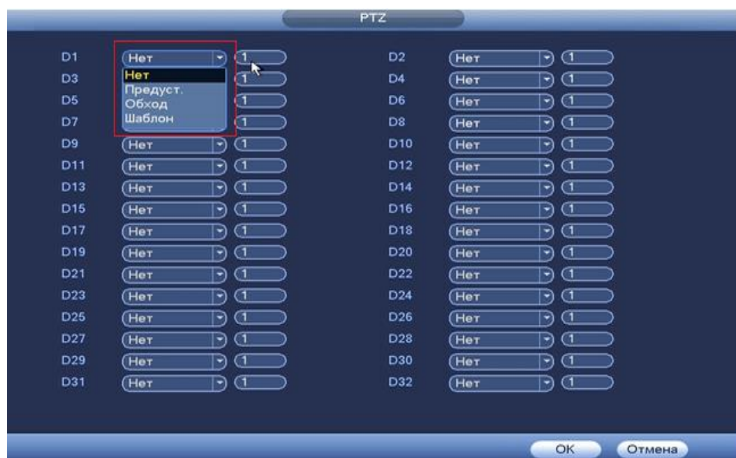
Рисунок 8.3.3.3.1.5 Установка предустановок.
