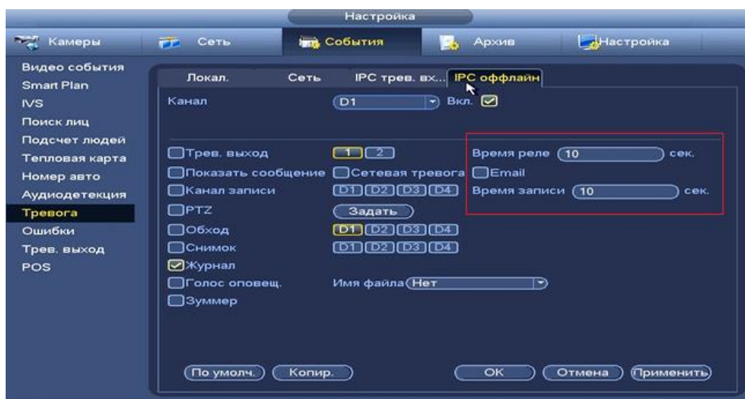
Рисунок 8.3.3.9.4.3 Установка настроек
