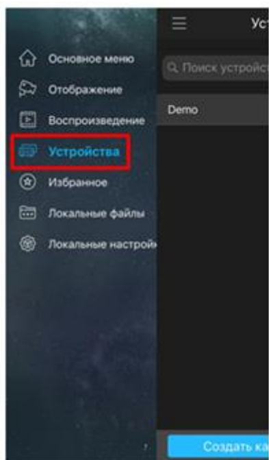
Рисунок 9.3.1 Меню устройства
