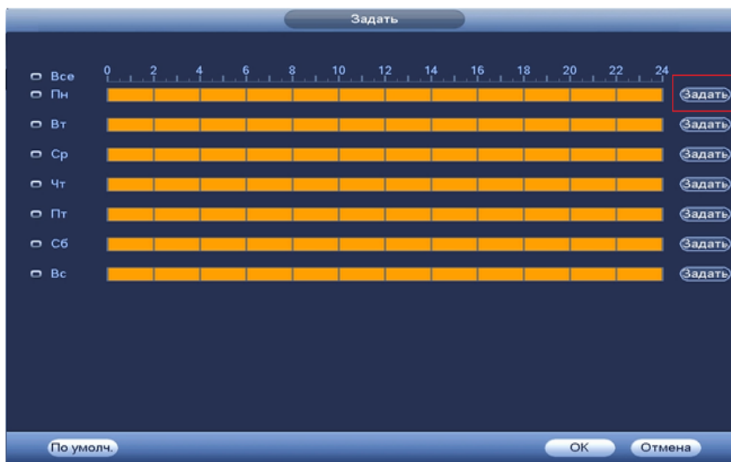
Рисунок 8.3.3.12.2 Настройка расписания.
