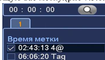
Рисунок 7.5.6.2 Выбор метки.
