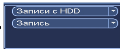
Рисунок 7.5.3.1 Тип поиска.
