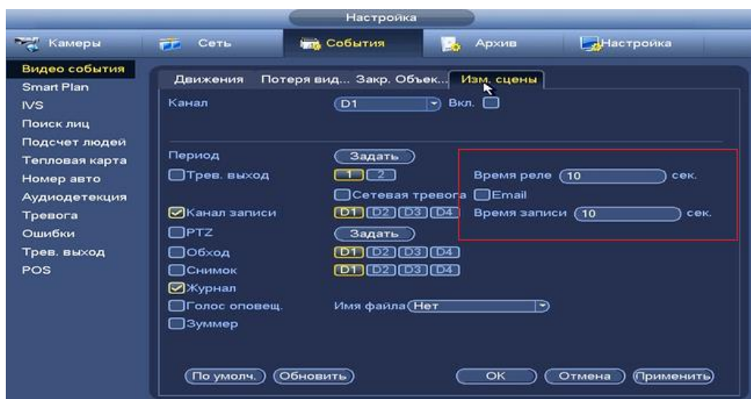
Рисунок 8.3.3.1.3.5 Установка настроек.
