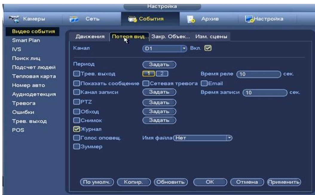
Рисунок 8.3.3.1.3.5 Установка настроек.
