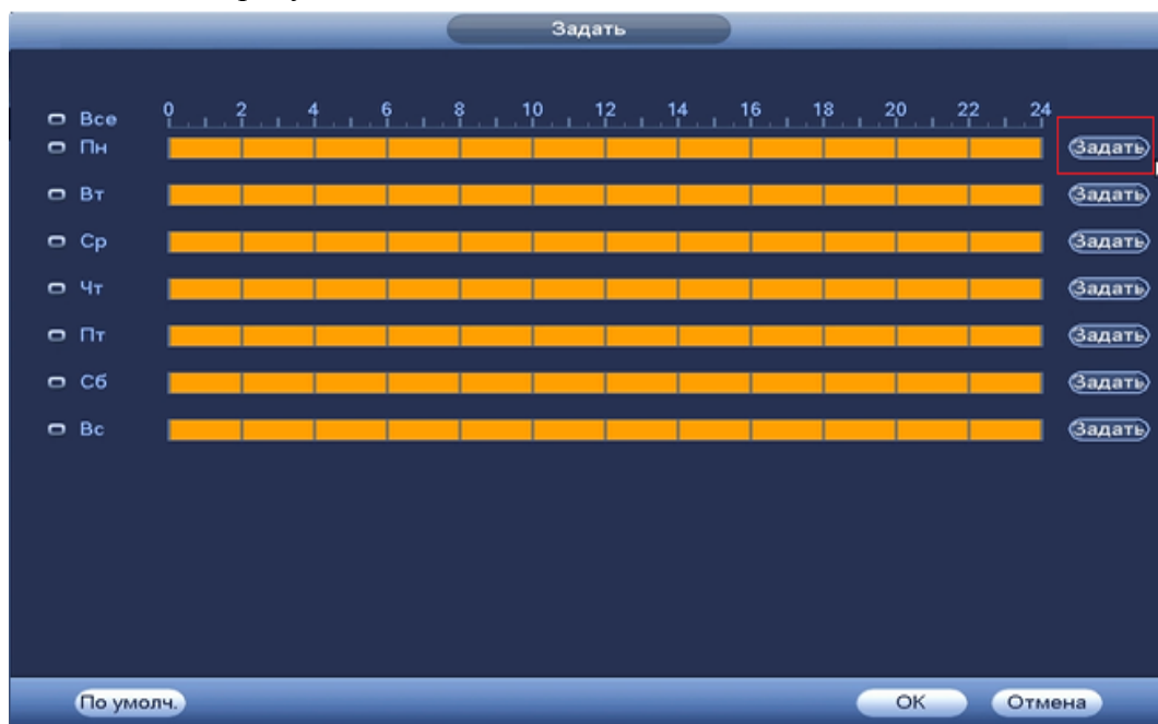
Рисунок 8.3.3.9.2.2 Настройка расписания.
