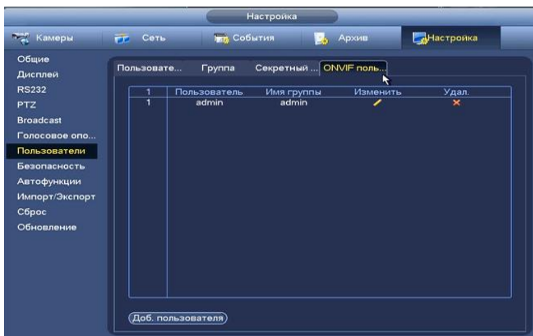
8.3.5.7.4.1 Настройка ONVIF.
