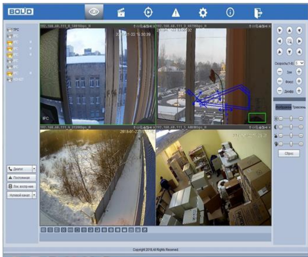
Рисунок 11.1 Web-интерфейс
