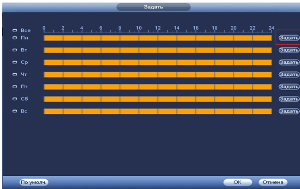
Рисунок 8.3.3.1.1.3 Настройка расписания.
