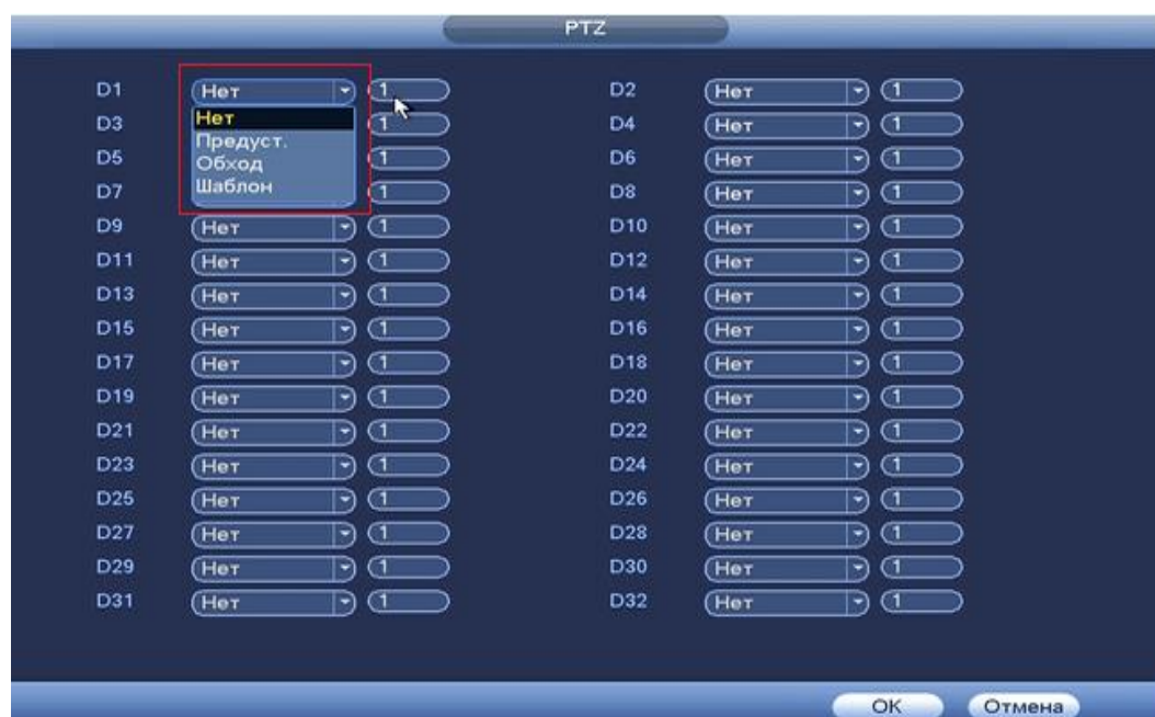
Рисунок 8.3.3.3.5 Установка предустановок.
