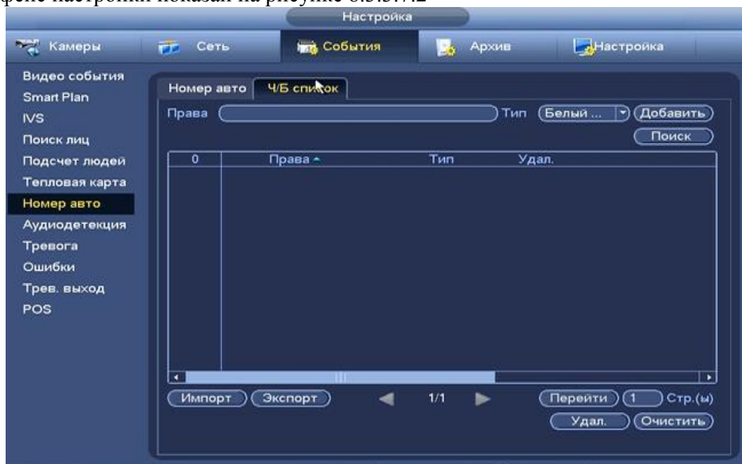
Рисунок 8.3.3.7.2 Ч/Б список
