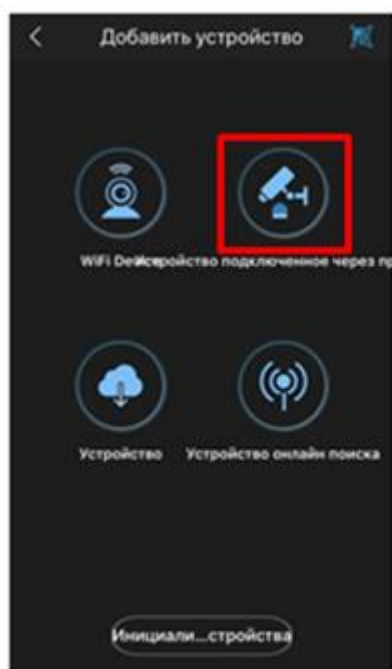
Рисунок 9.3.3 Меню добавления
