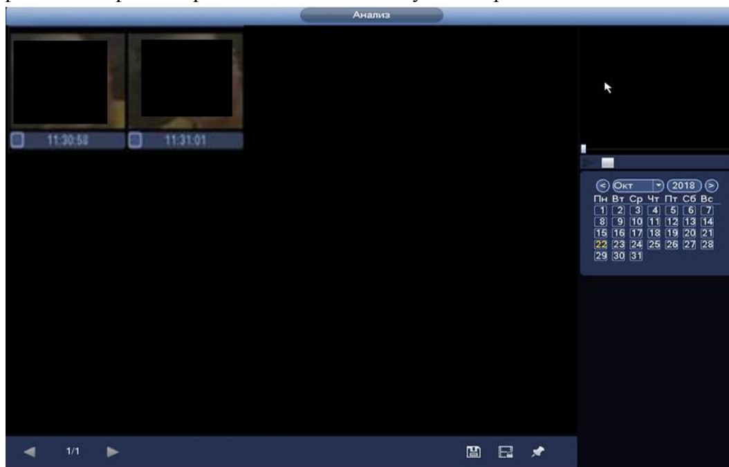
Рисунок 8.1.2.2.1 Распознавание лиц.
