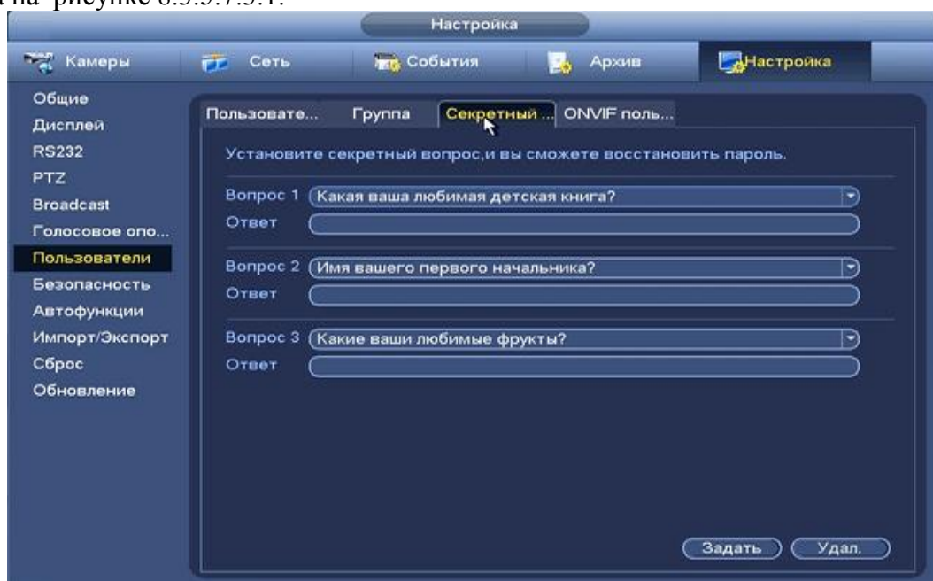
Рисунок 8.3.5.7.3.1 Интерфейс настройки
