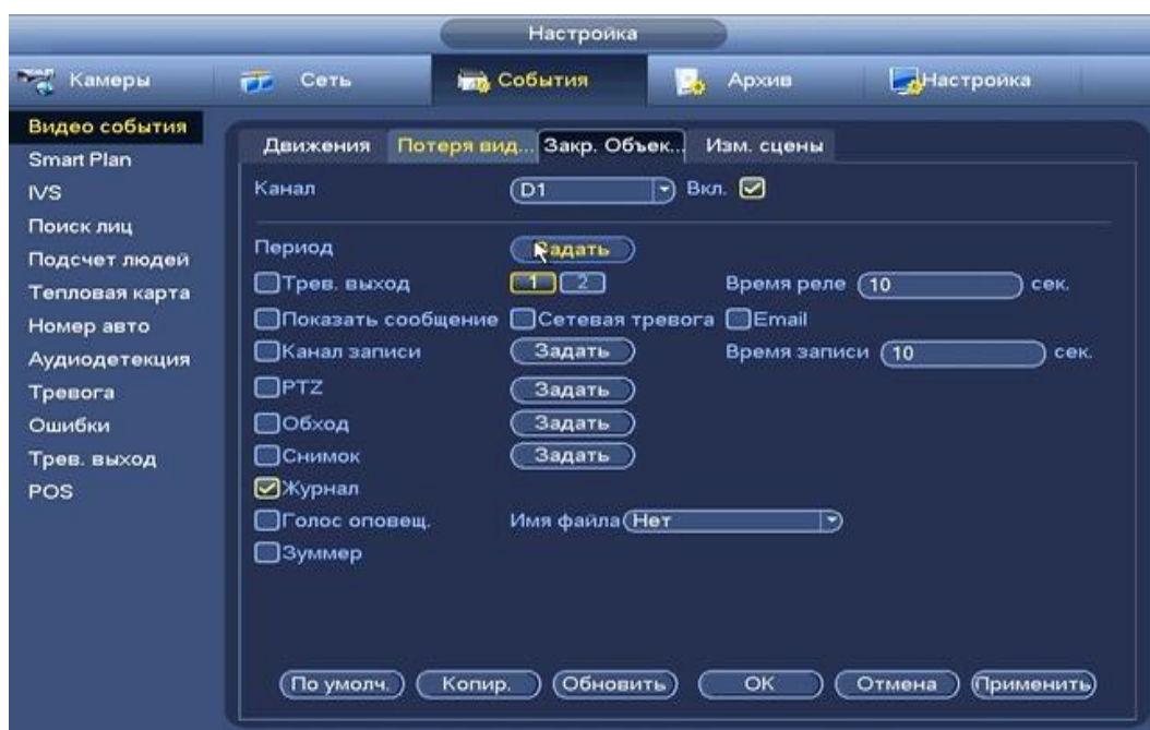
Рисунок 8.3.3.1.2.5 Установка настроек.
