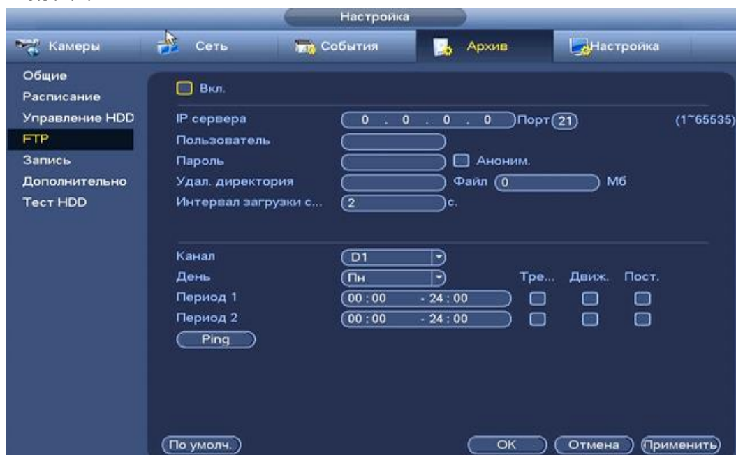
Рисунок 8.3.4.4.1 Настройка FTP
