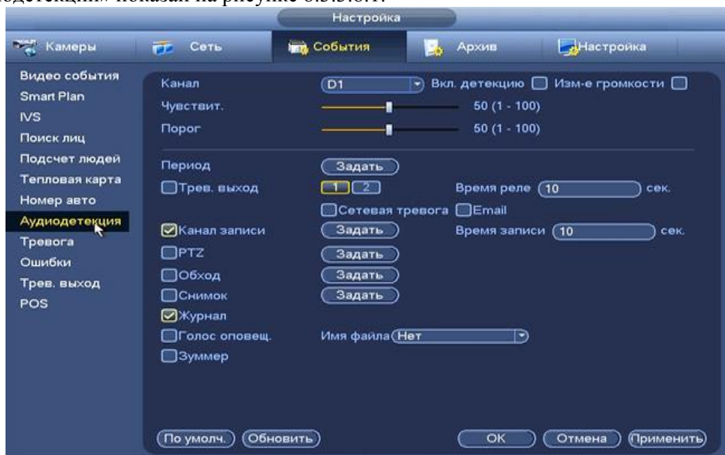
Рисунок 8.3.3.8.1 Настройка аудиодетекция.
