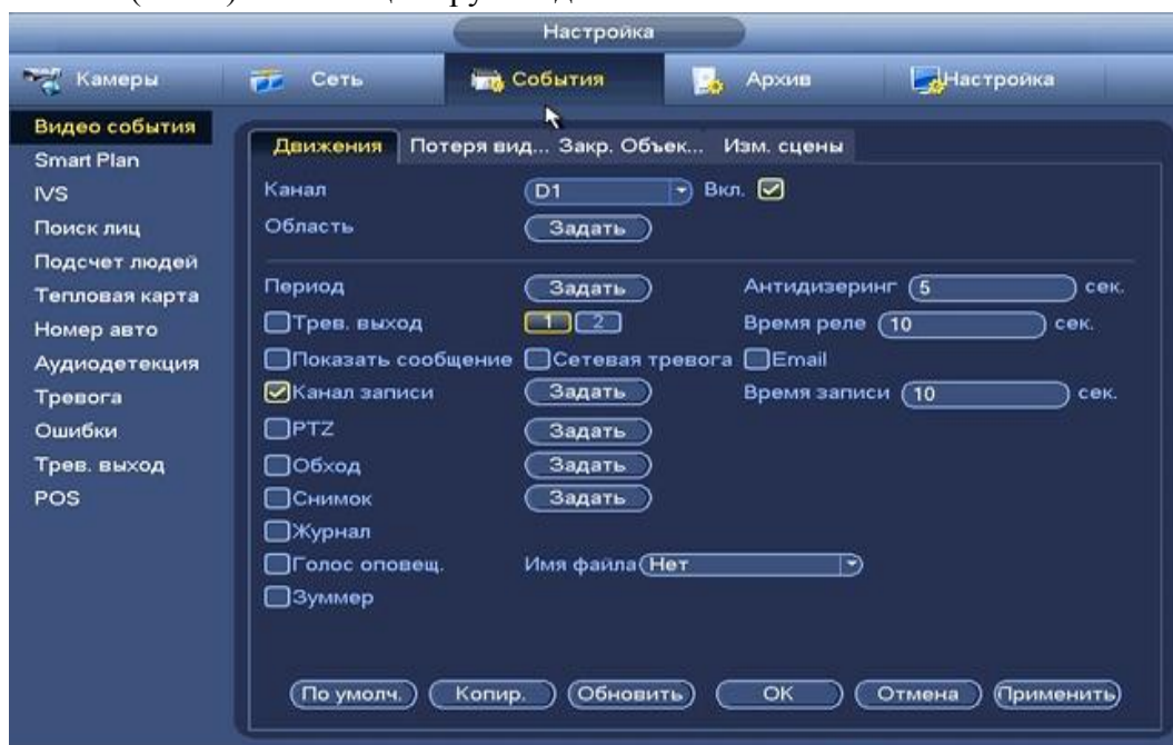
Рисунок 8.3.3.1.1.6 Установка настроек
