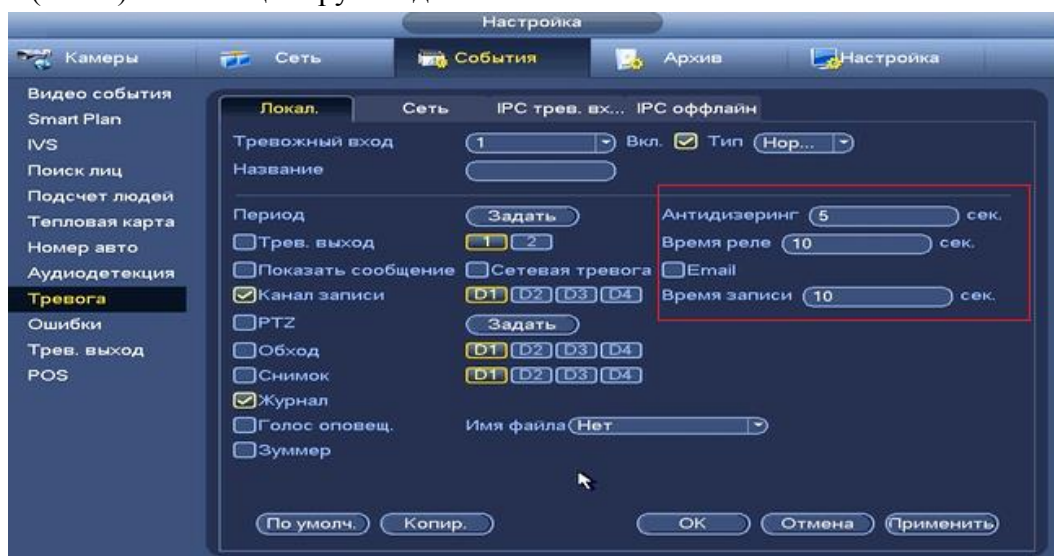
Рисунок 8.3.3.9.1.5 Установка настроек.
