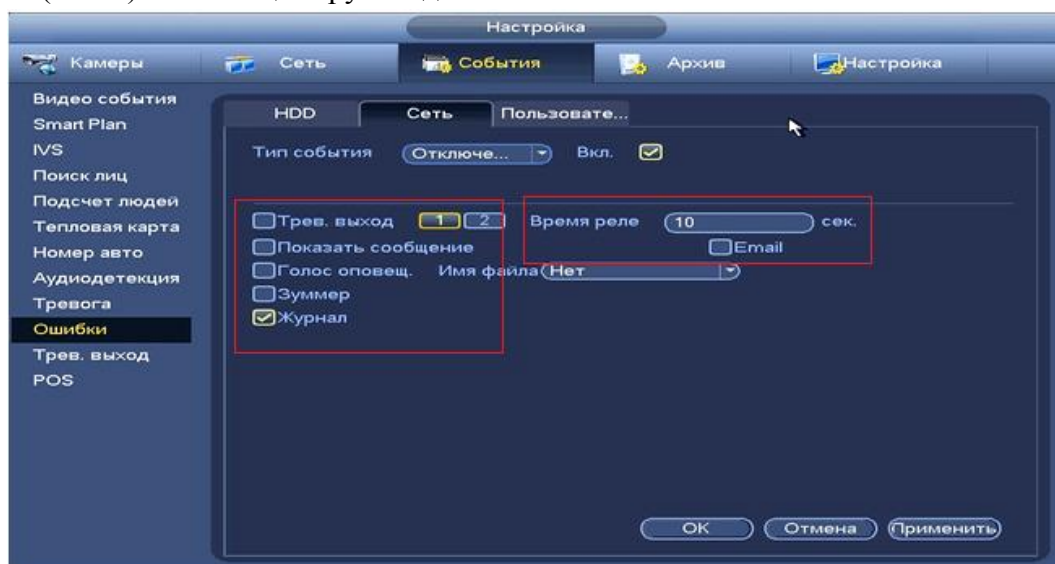
Рисунок 8.3.3.10.2.2 Установка настроек.
