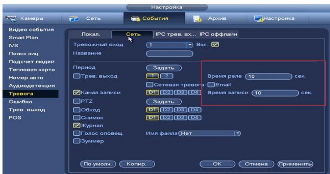
Рисунок 8.3.3.9.2.5 Установка настроек.
