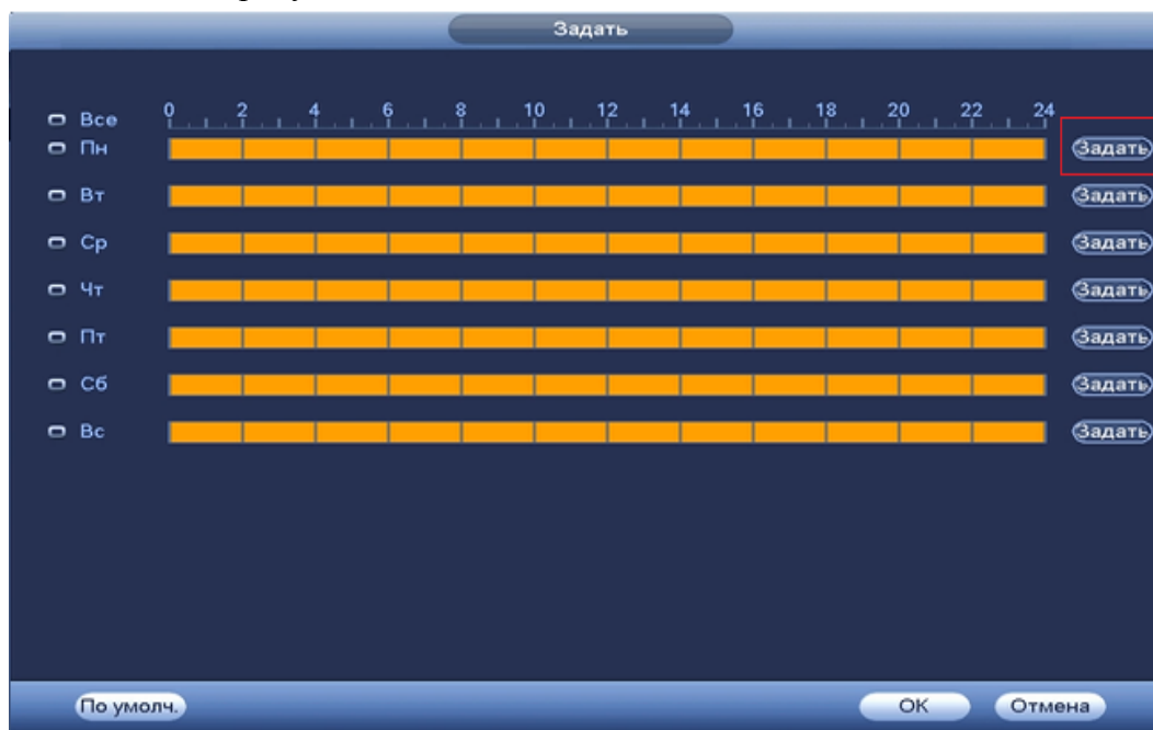
Рисунок 8.3.3.2.3 Настройка расписания.
