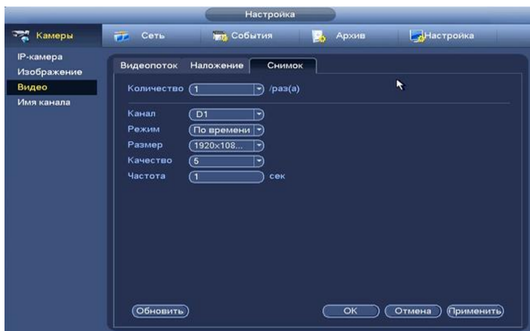
Рисунок 8.3.1.3.2.1 Настройка снимка
