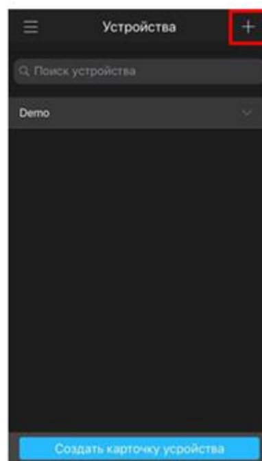
Рисунок 9.3.2 Меню устройства.
