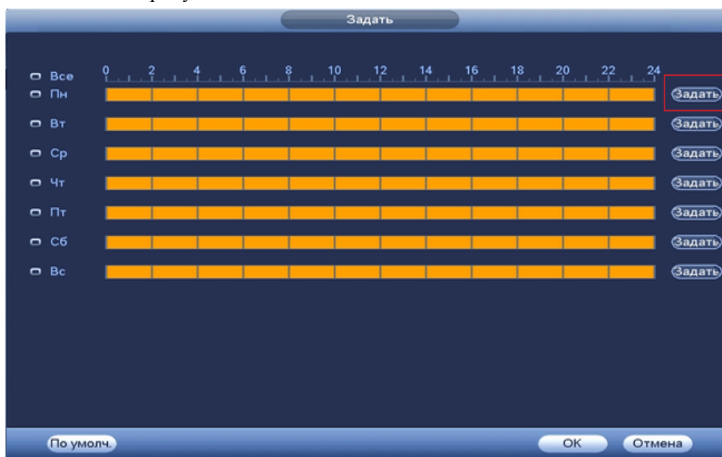
Рисунок 8.3.3.1.2.2 Настройка расписания.
