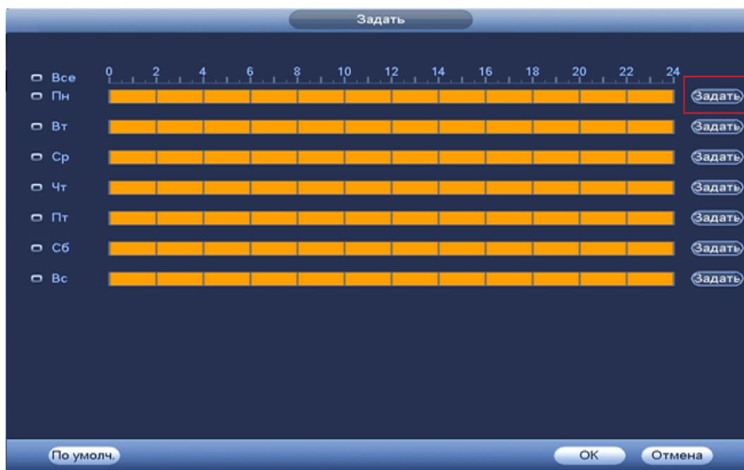
Рисунок 8.3.3.8.2 Настройка расписания.
