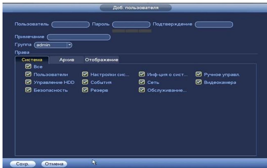
Рисунок 8.3.5.7.1.2 Назначение прав.
