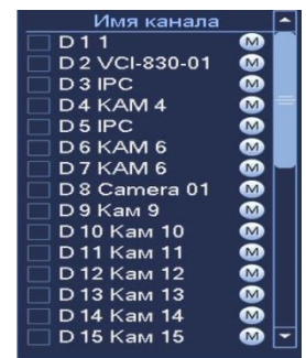
Рисунок 8.1.5.1 Каналы воспроизведения
