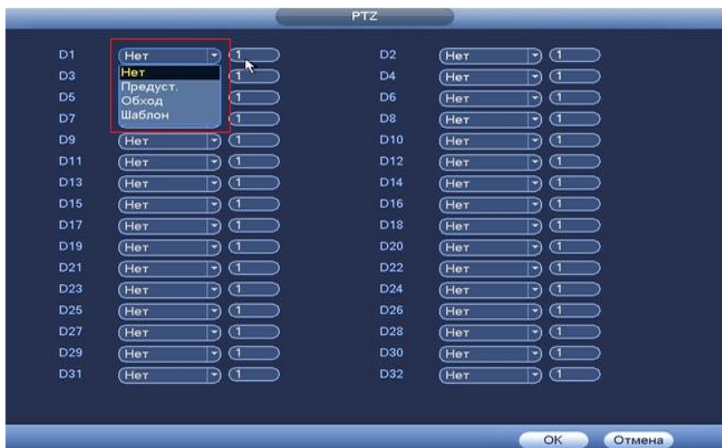
Рисунок 8.3.3.4.5 Установка предустановок.
