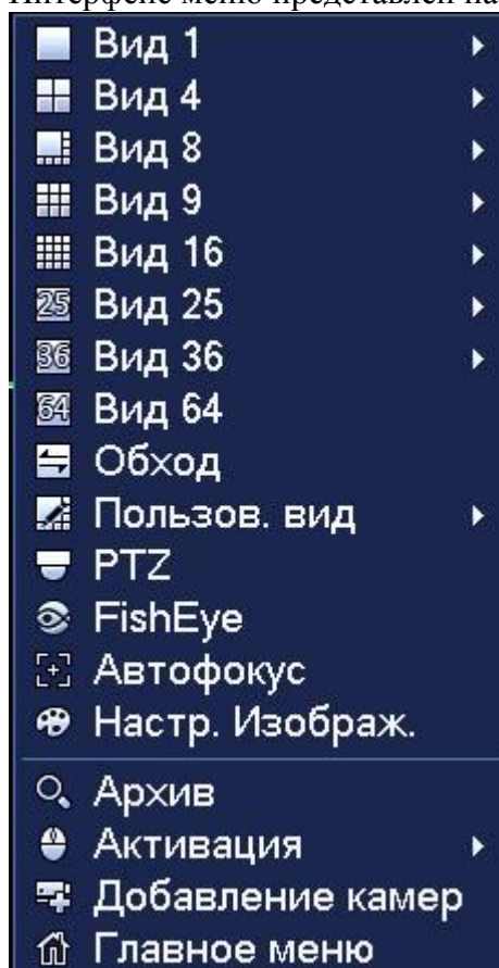
Рисунок 7.1 Контекстное меню.
