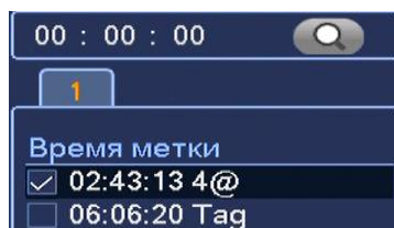
Рисунок 8.1.6.2 Выбор метки.
