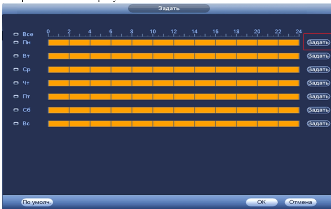
Рисунок 8.3.3.4.3 Настройка расписания.
