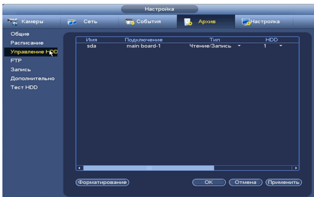
Рисунок 8.3.4.3.1 Интерфейс настройки
