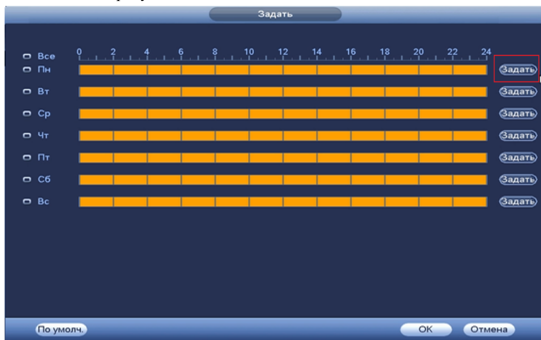
Рисунок 8.3.3.9.3.2 Настройка расписания.
