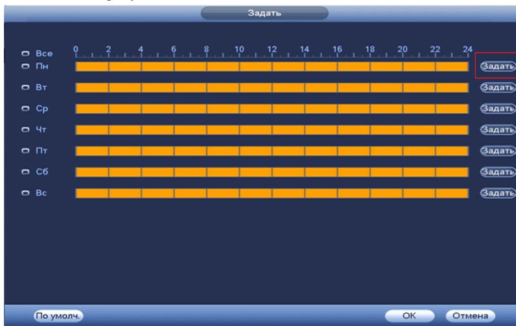
Рисунок 8.3.3.1.3.2 Настройка расписания.
