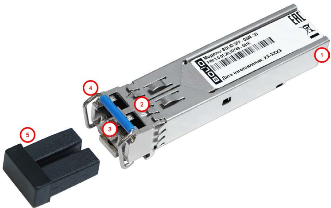
Рисунок 4.1 – Устройство SFP-модуля
