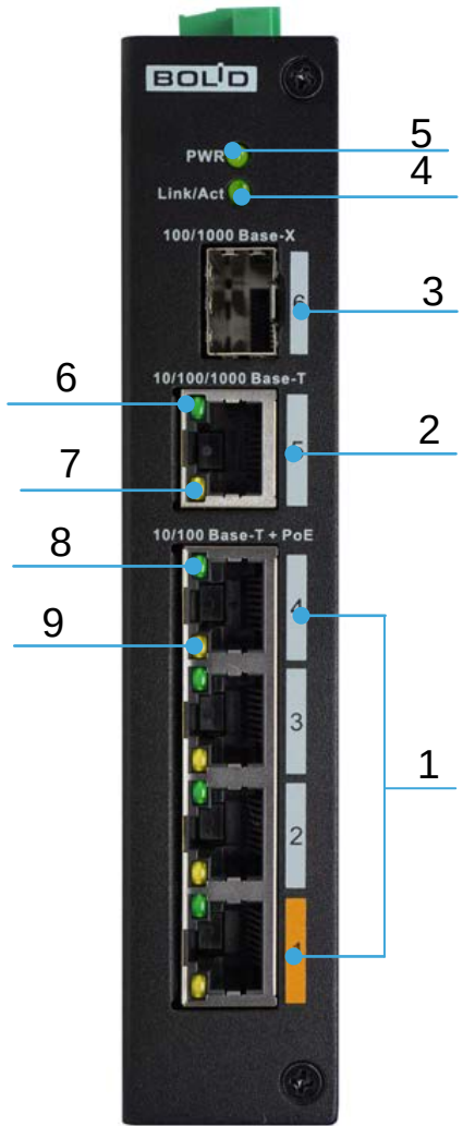
Рисунок 5.2 – Передняя панель Расшифровка передней панели (Таблица 5.2).
