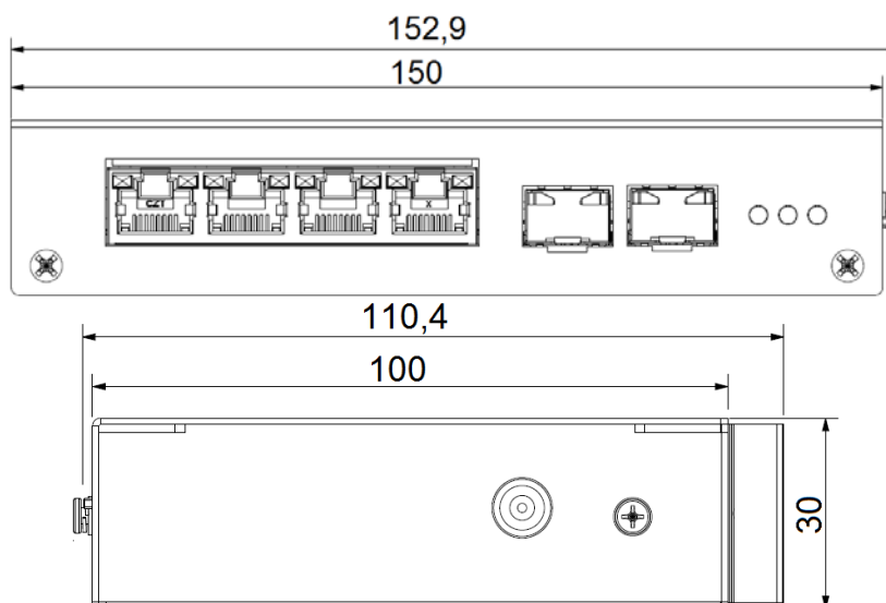
Рисунок 5.1 – Габаритные размеры
