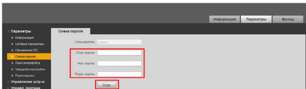
Рисунок 6.2 – Смена пароля
