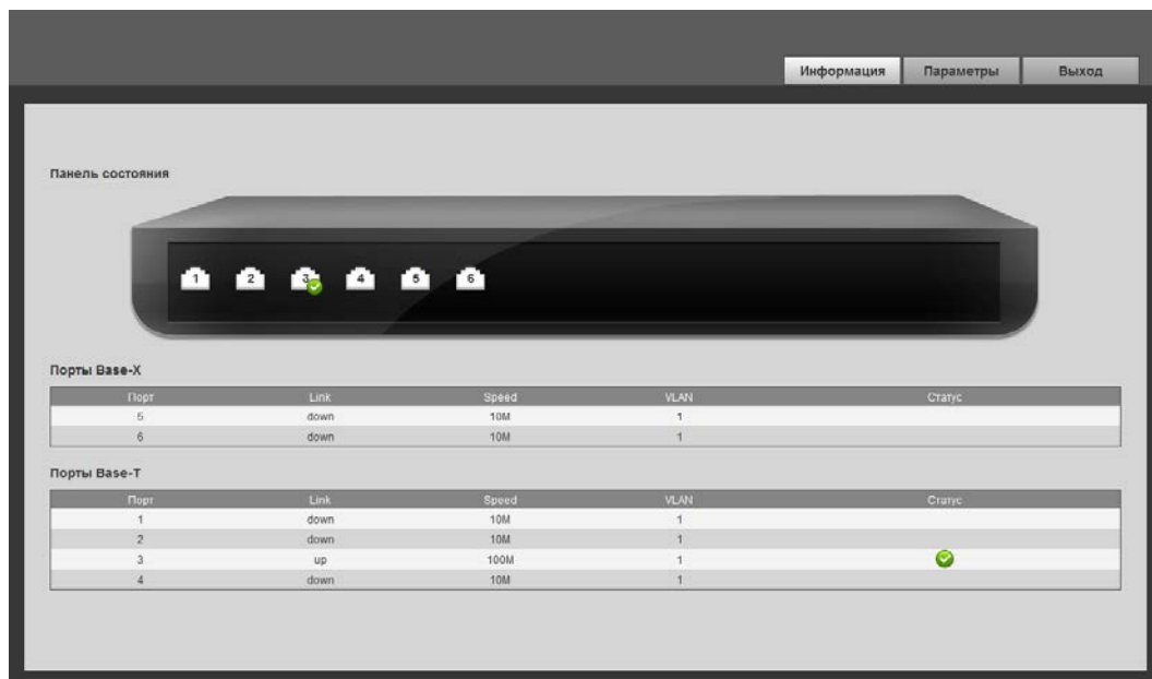
Рисунок 7.1 – Информационная панель
