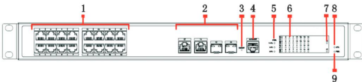
Рисунок 1 – Передняя панель
