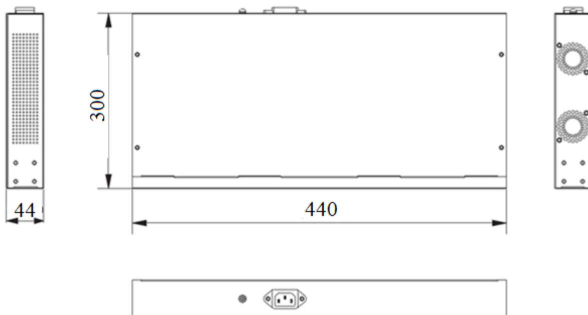
Рисунок 2 – Габаритные размеры
