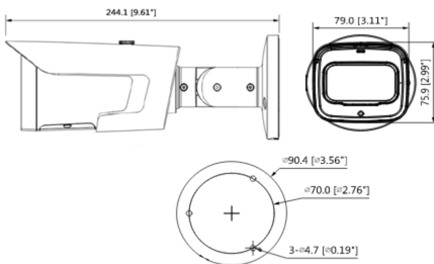
Рисунок 5.1 – Габаритные размеры видеокамеры
