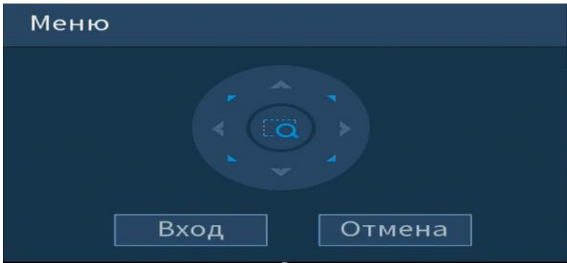
Рисунок 7.3 – Виртуальный джойстик
