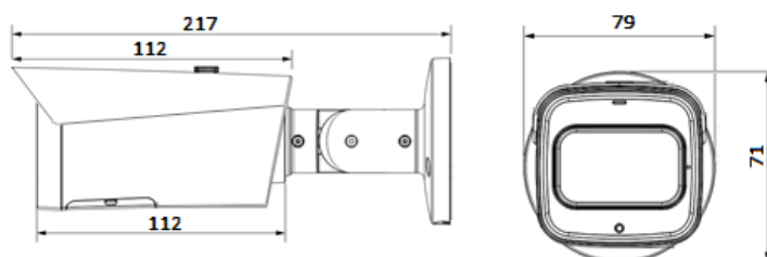
Рисунок 5.1 – Габаритные размеры видеокамеры
