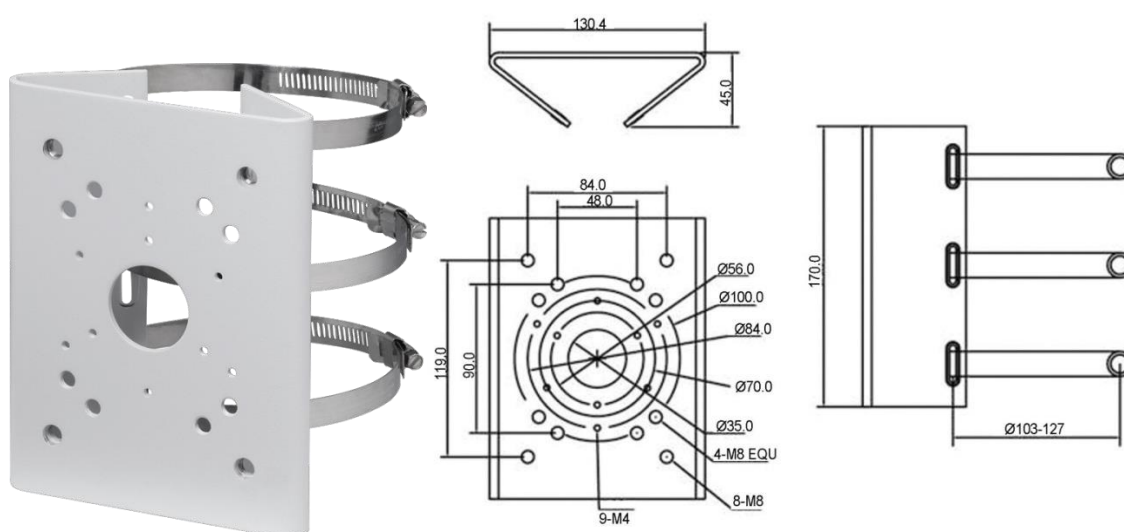
Рисунок 5.7 – Столбвой кронштейн BR-103
