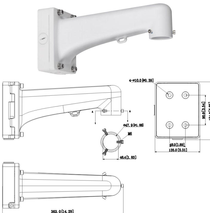
Рисунок 5.7 – Настенный кронштейн BR-110
