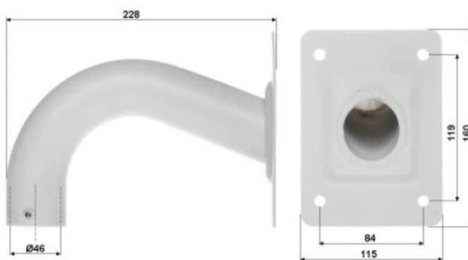
Рисунок 5.2 – Габаритные размеры настенного кронштейна
