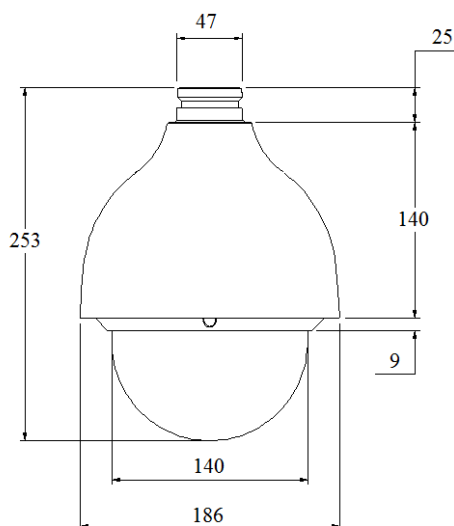
Рисунок 5.1 – Габаритные размеры видеокamеры
