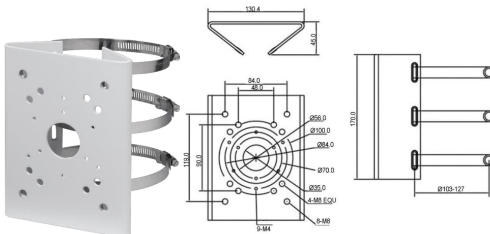
Рисунок 5.14 – Столбовой кронштейн BR-103
