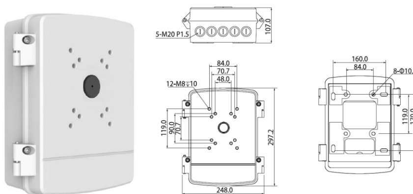
Рисунок 5.5 – Монтажная коробка BR-203
