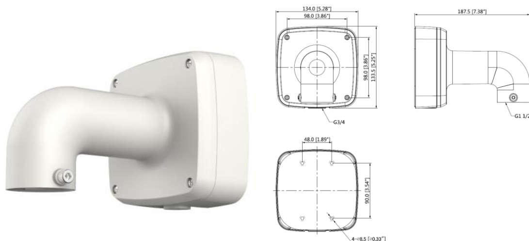
Рисунок 5.9 – Настенный кронштейн BR-107
