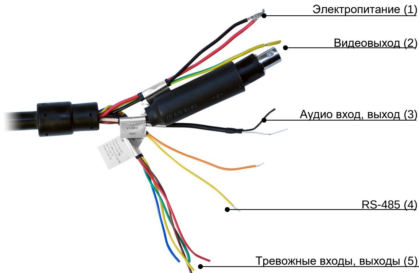
Рисунок 6.1 – Группы концевой раскладки кабеля видеокamеры
