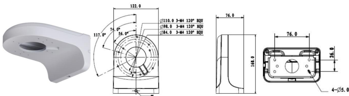
Рисунок 5.4 – Внешний вид и габаритные размеры кронштейна BR-105
