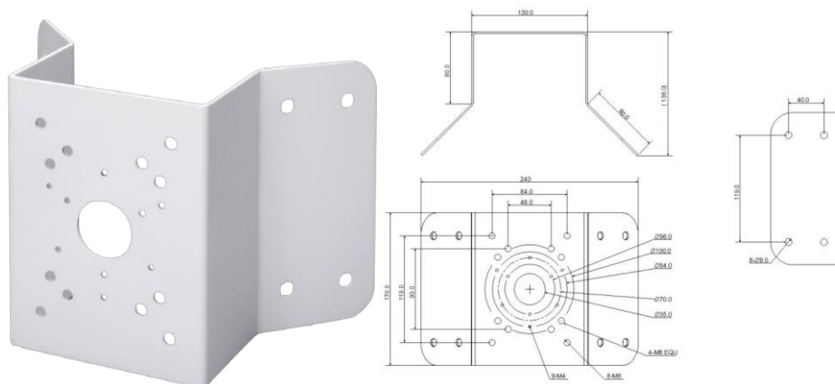
Рисунок 5.10 – Угловой кронштейн BR-102
