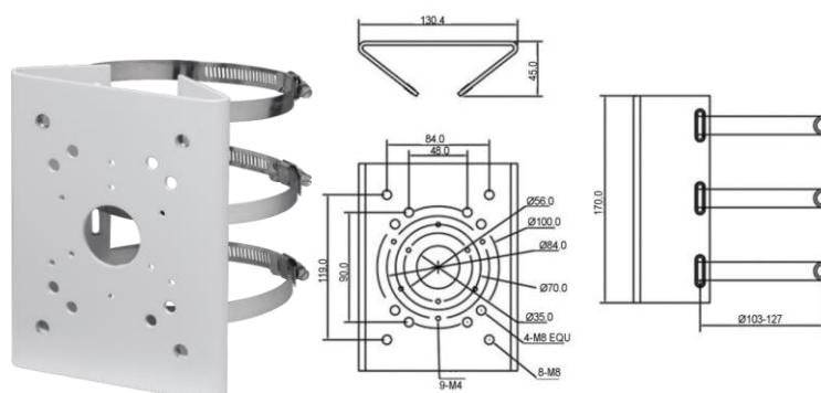
Рисунок 5.13 – Столбвой кронштейн BR-103
