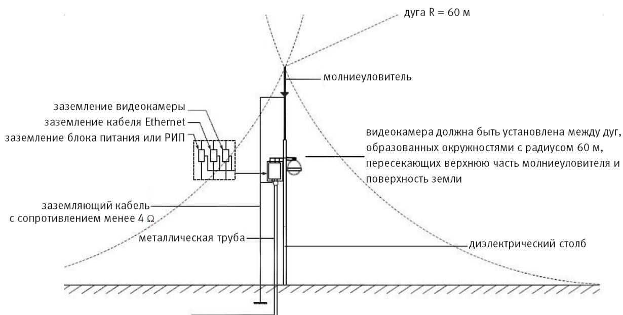
Рисунок 6.7 – Установка молниеотвода
