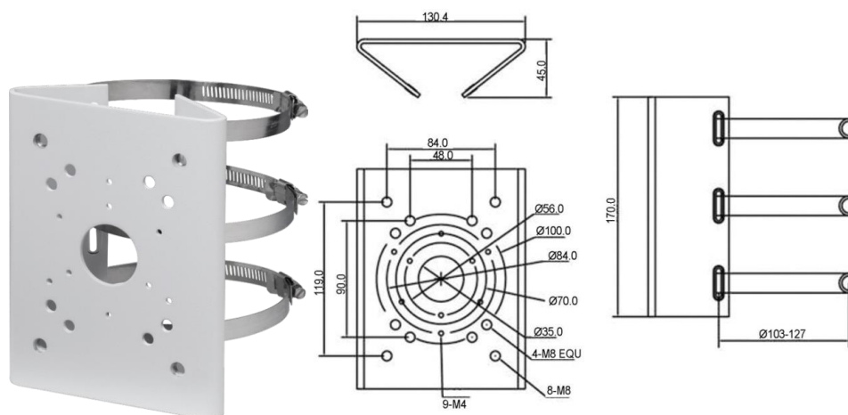
Рисунок 5.11 — Столбвой кронштейн BR-103
