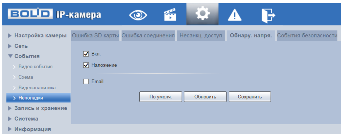
Рисунок 7.82 — Вкладка «Обнаружение напряжения»
