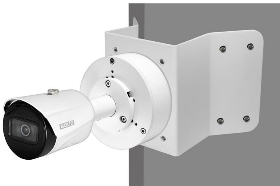
Рисунок 5.10 — Монтаж видеокамеры и монтажной коробки BR-204 на угловом кронштейне BR-102
