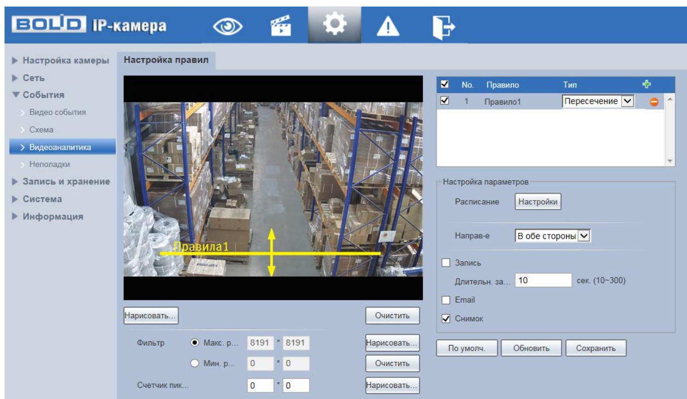
Рисунок 7.76 — Создание правила видеоаналитики «Пересечение линии»
