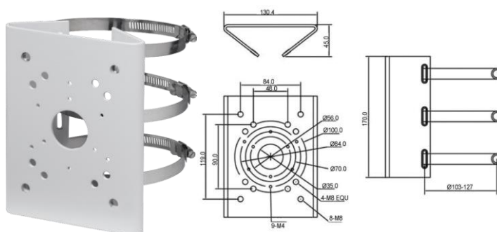
Рисунок 5.11 – Столбовой кронштейн BR-103
