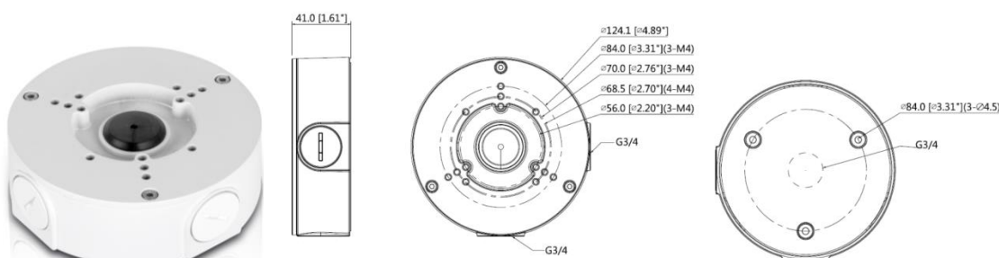
Рисунок 5.3 – Монтажная коробка BR-204
