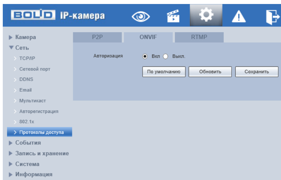
Рисунок 7.64 – Вкладка «ONVIF»
