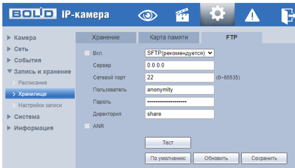
Рисунок 7.98 – Вкладка «FTP»
