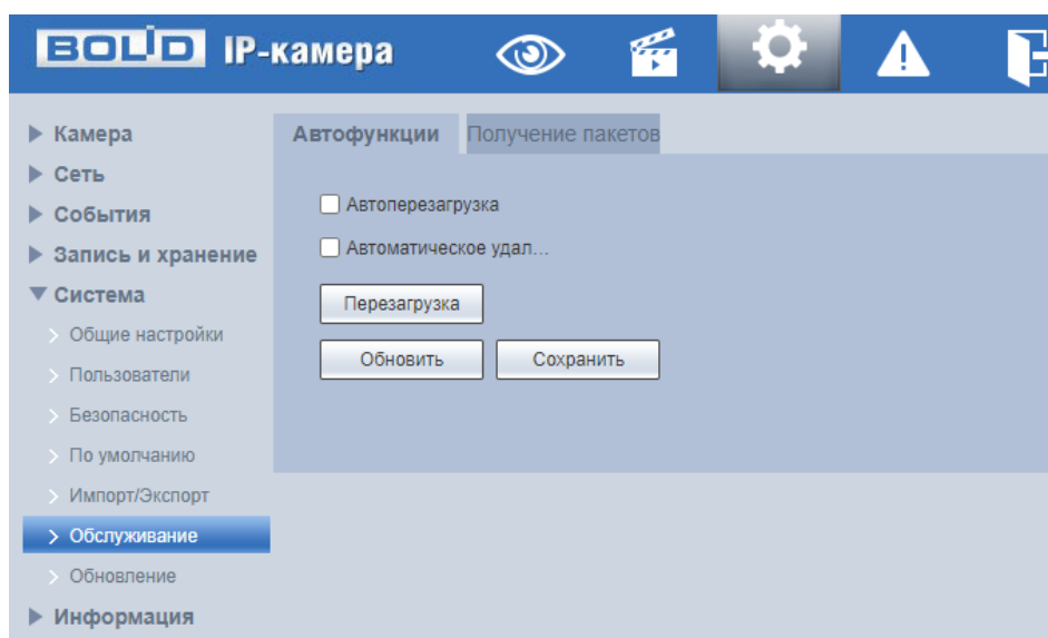
Рисунок 7.121 – Вкладка «Автофункции»
