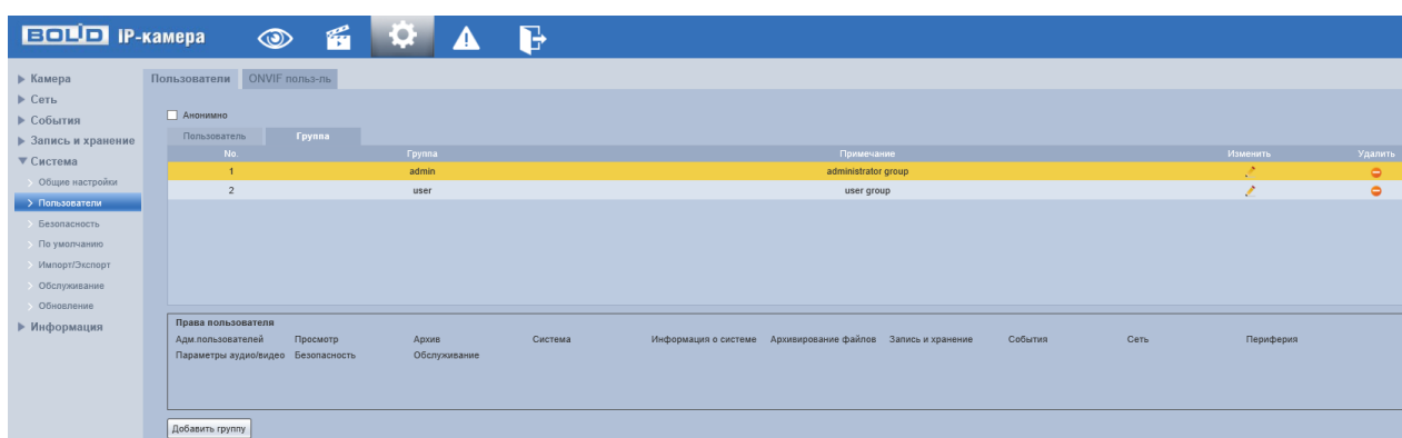
Рисунок 7.108 – Вкладка «Группа»
