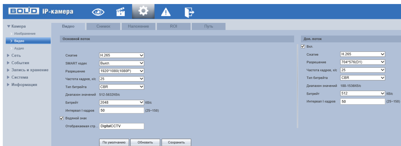
Рисунок 7.40 – Вкладка «Видео»
