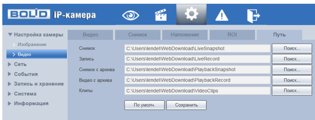
Рисунок 7.49 – Вкладка «Путь»
