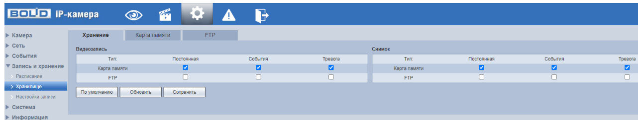
Рисунок 7.96 – Вкладка «Хранение»
