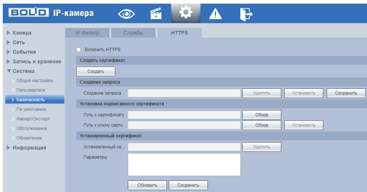
Рисунок 7.116 – Вкладка «HTTPS»
