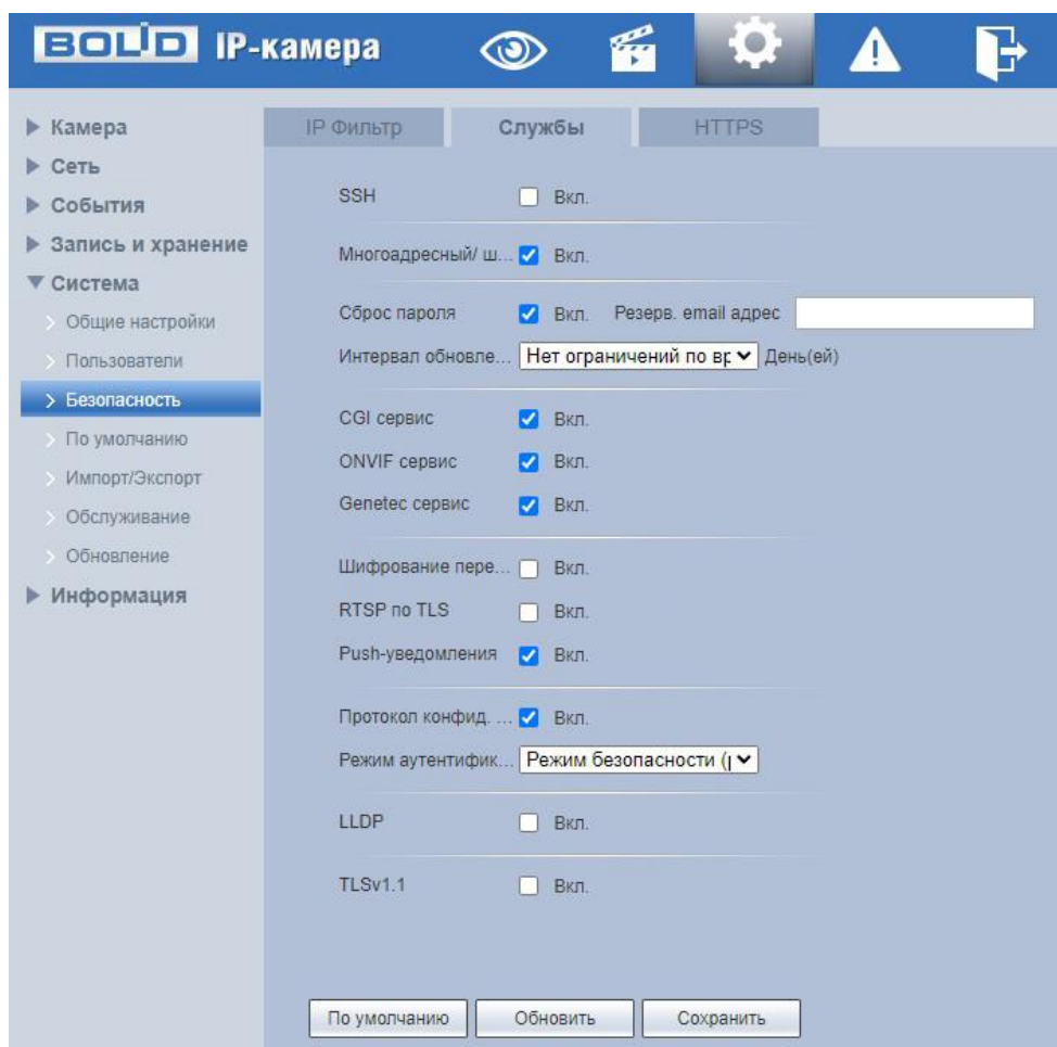
Рисунок 7.115 – Вкладка «Службы»
