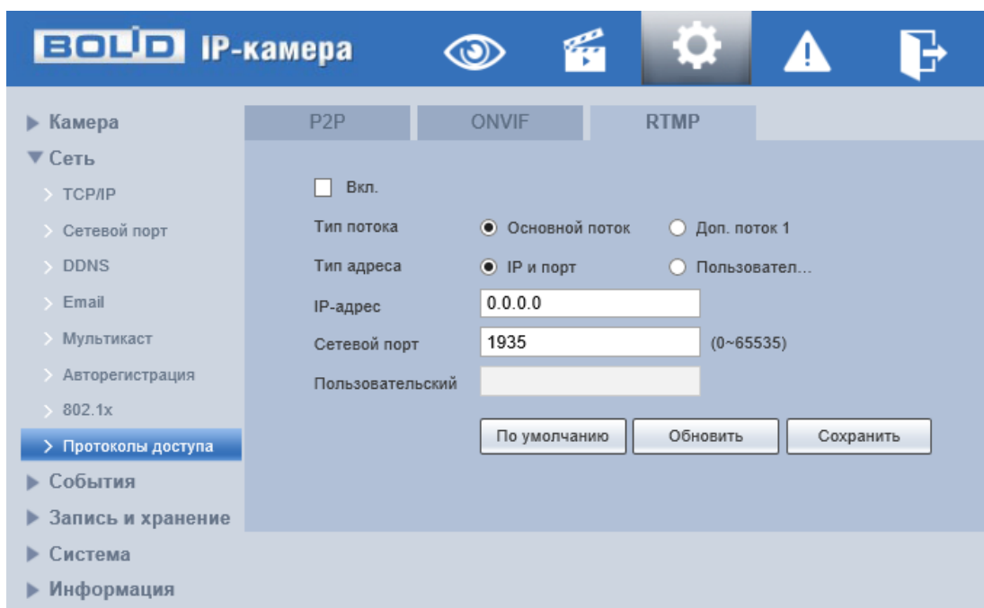
Рисунок 7.65 – Вкладка «RTMP»
