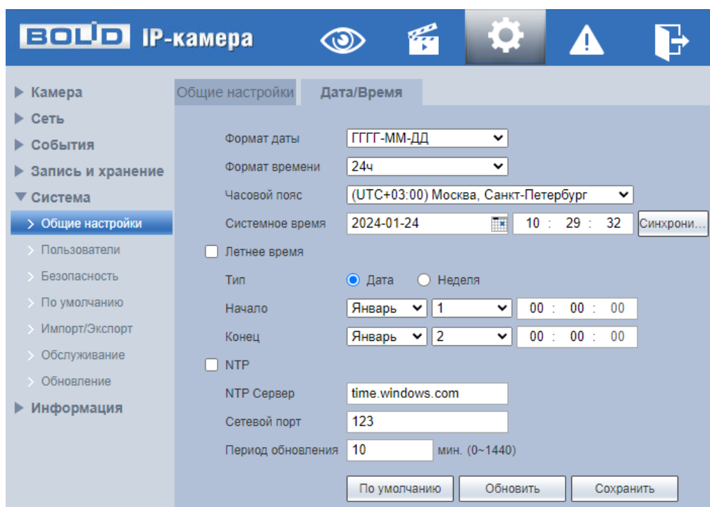
Рисунок 7.104 – Вкладка «Дата/Время»
