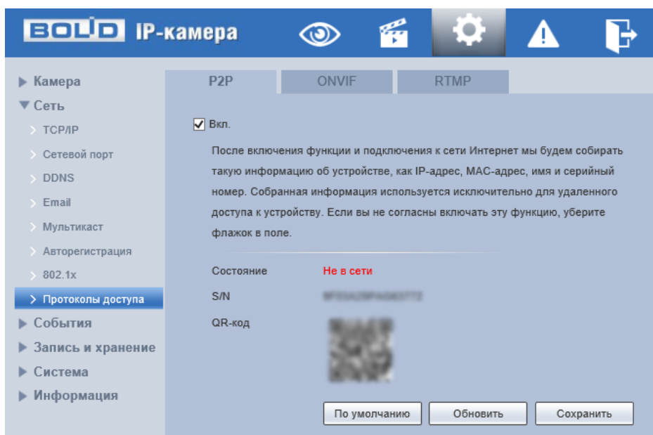
Рисунок 7.63 – Вкладка «P2P»
