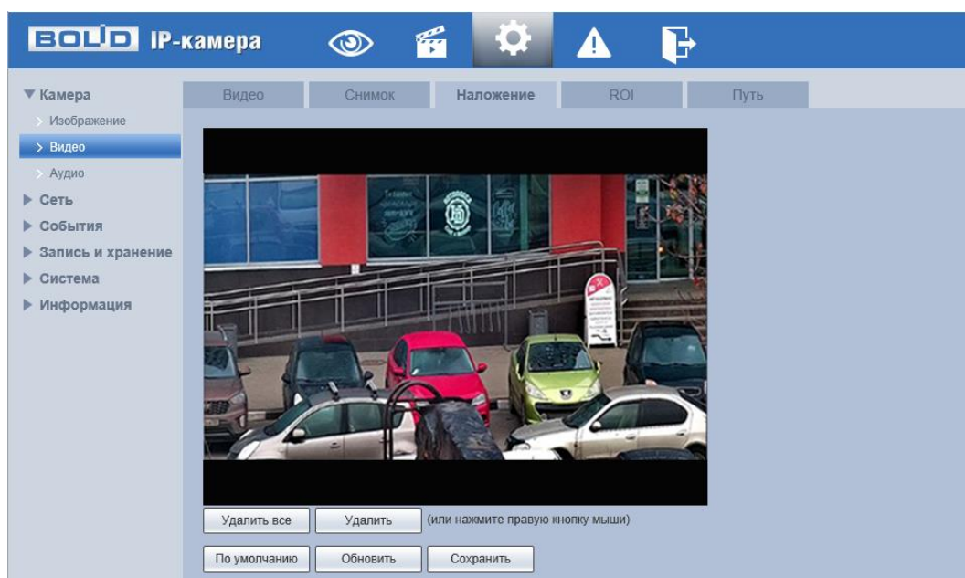
Рисунок 7.42 – Вкладка «Наложение»
