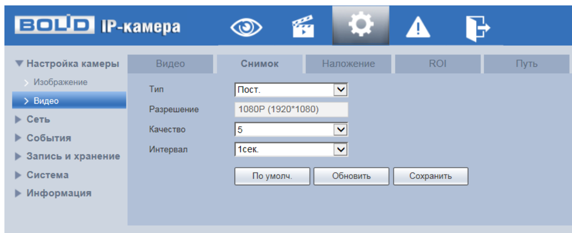
Рисунок 7.41 – Вкладка «Снимок»
