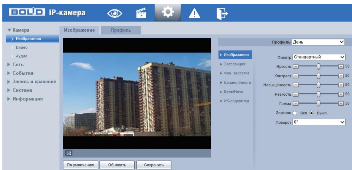
Рисунок 7.29 – Вкладка «Изображение»
