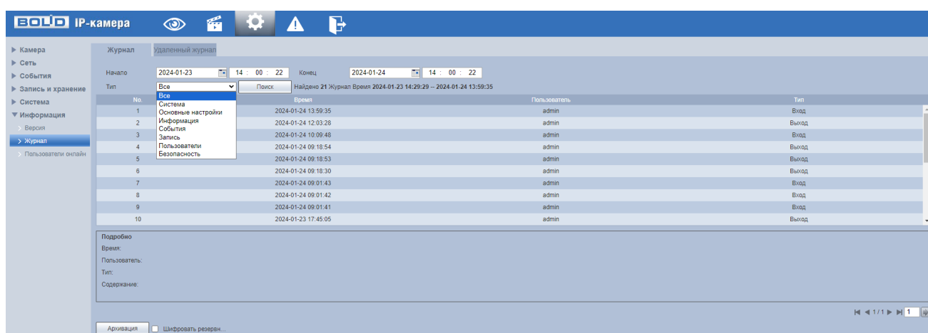
Рисунок 7.127 – Вкладка «Журнал»
