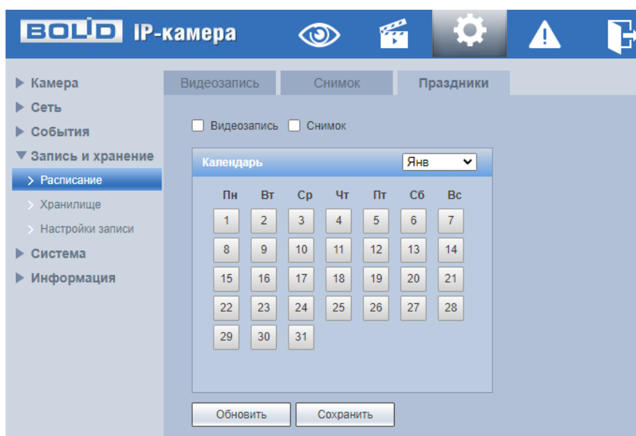
Рисунок 7.94 – Вкладка «Праздники»
