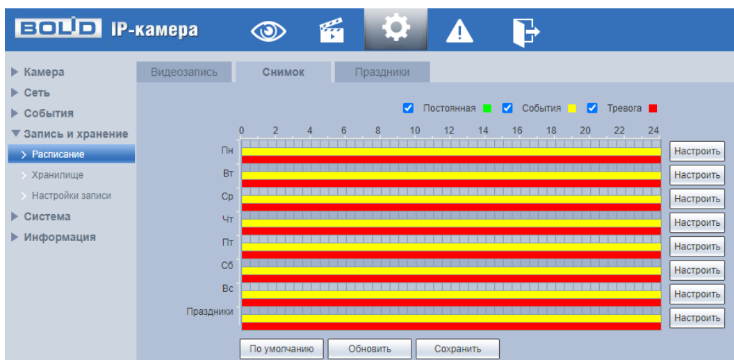
Рисунок 7.92 – Вкладка «Снимок»
