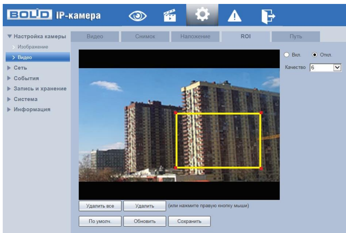
Рисунок 7.48 – Вкладка «ROI»
