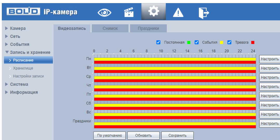
Рисунок 7.90 – Вкладка «Видеозапись»
