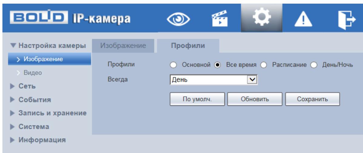
Рисунок 7.38 – Вкладка «Профиль»
